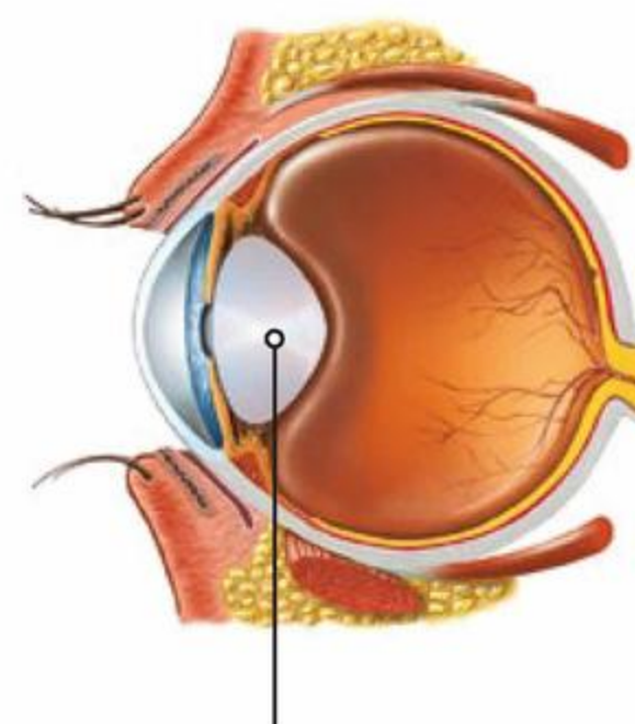
soczewka wypukła
