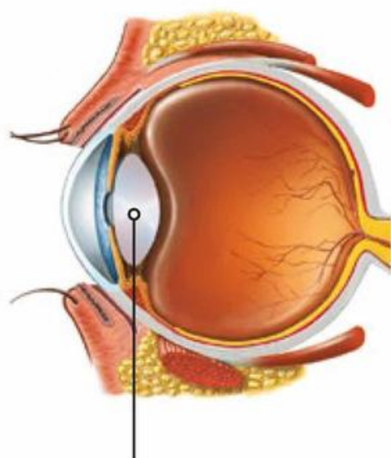
soczewka spłaszczona
