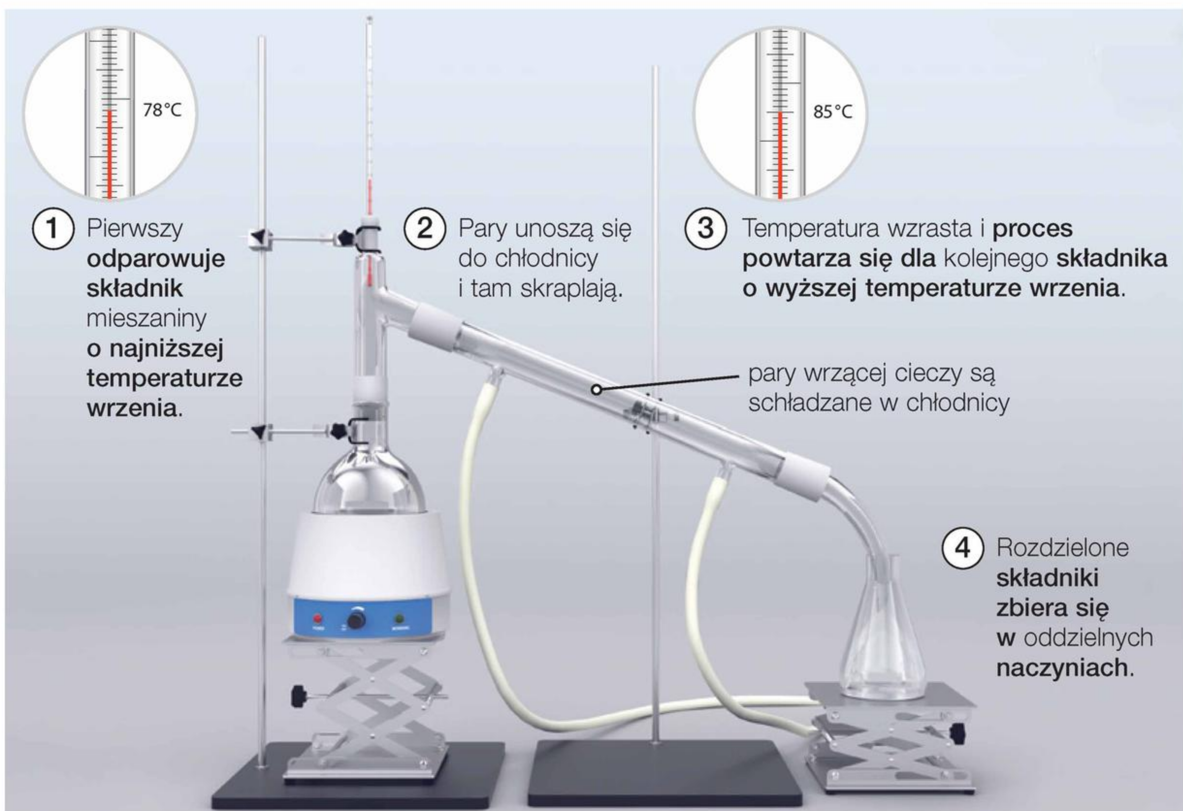
Rys. 4. Zestaw do destylacji.
