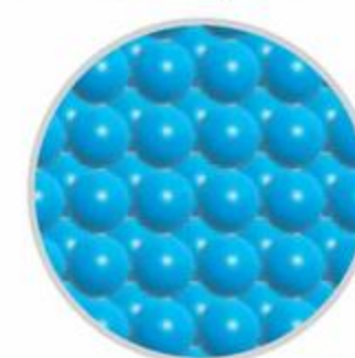
substancja stała
