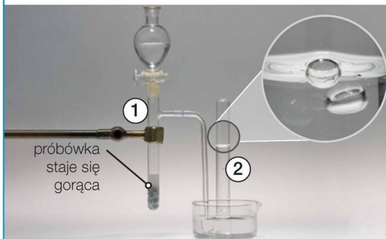
Fot. 56. Otrzymywanie wodoru w reakcji cynku z kwasem chlorowodorowym.
