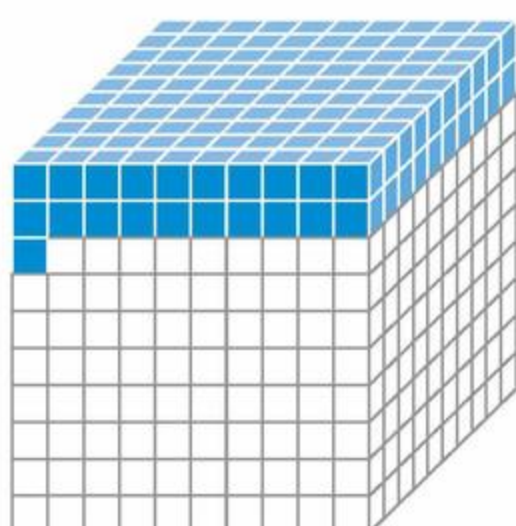
Rys. 6. Procent objętościowy tlenu (21%) w powietrzu.
