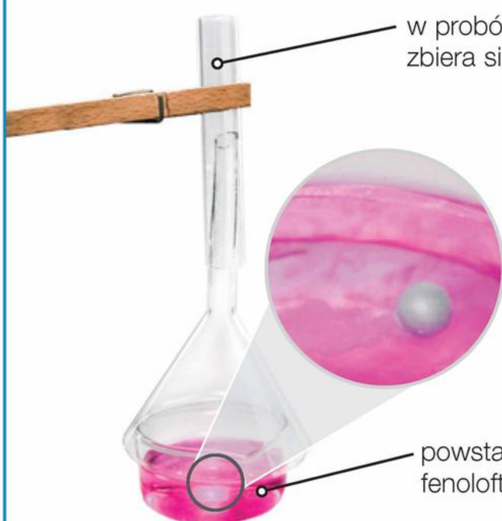
Fot. 135. Otrzymywanie wodorotlenku sodu w reakcji sodu z wodą.
