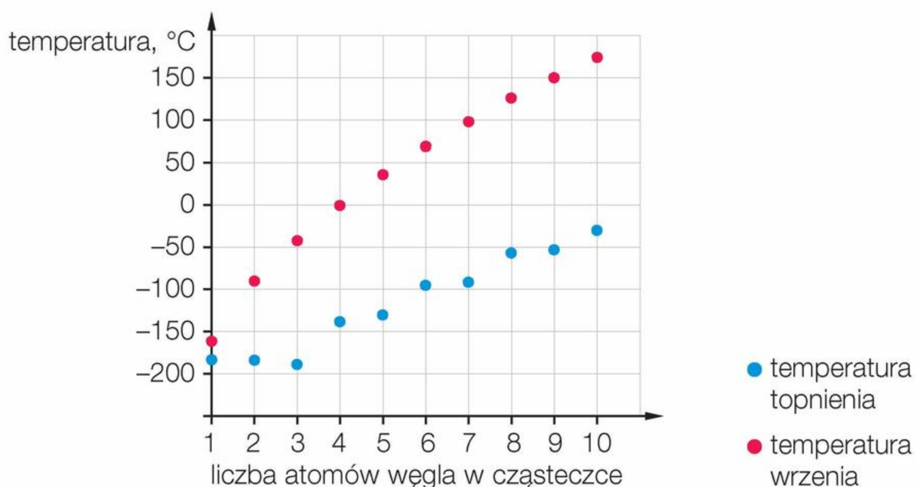
Rys. 6. Wykres zależności temperatur wrzenia i topnienia alkanów od liczby atomów węgla w ich cząsteczkach (mierzone pod ciśnieniem 1013 hPa).
