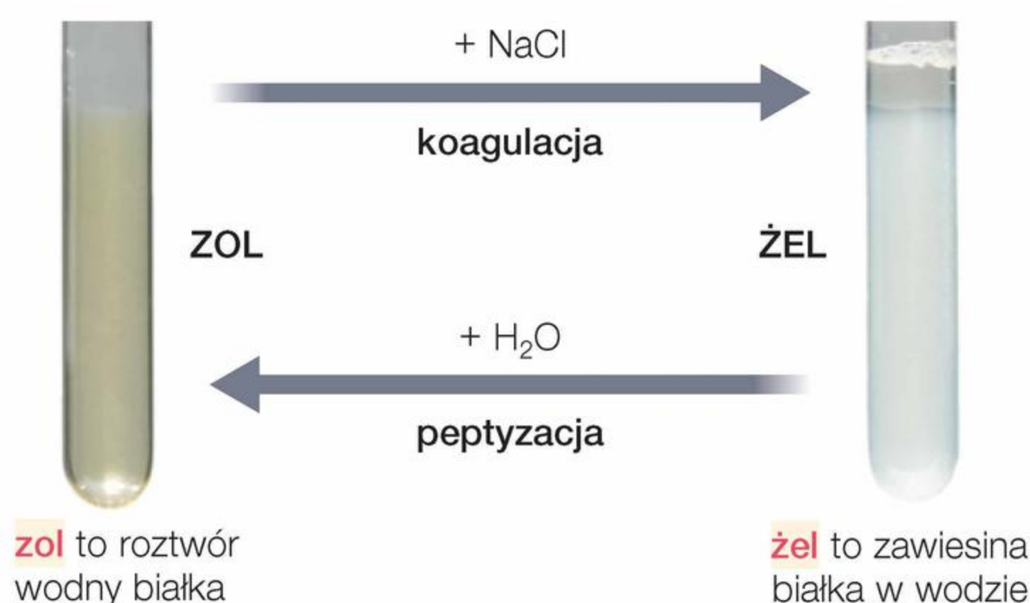
Fot. 139. Koagulacja odwracalna i peptyzacja.
