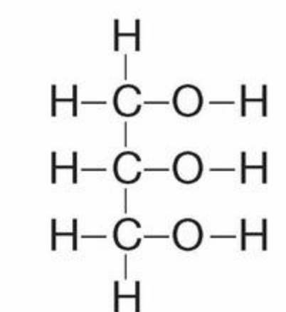
wzór strukturalny
