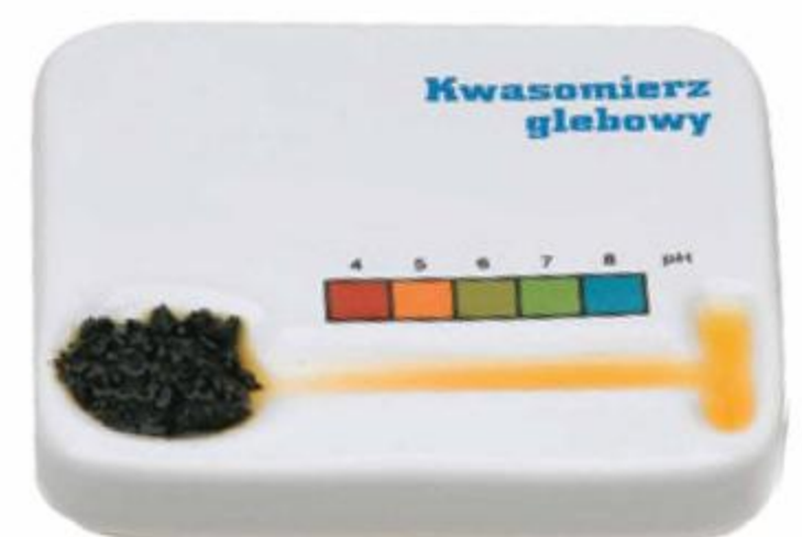
Fot. 30. pH gleby można zbadać kwasomierzem.
