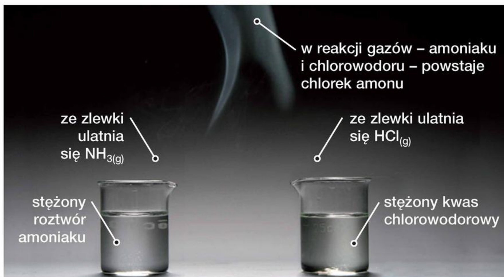
Fot. 54. Biała chmura widoczna nad zlewkami to mikroskopijnej wielkości kryształki soli – chlorku amonu \text{NH}_4\text{Cl} .
