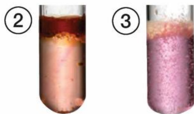
Fot. 118. Reakcja zakwaszonego wodnego roztworu manganianu(VII) potasu z: kwasem stearynowym ②, kwasem oleinowym ③.
