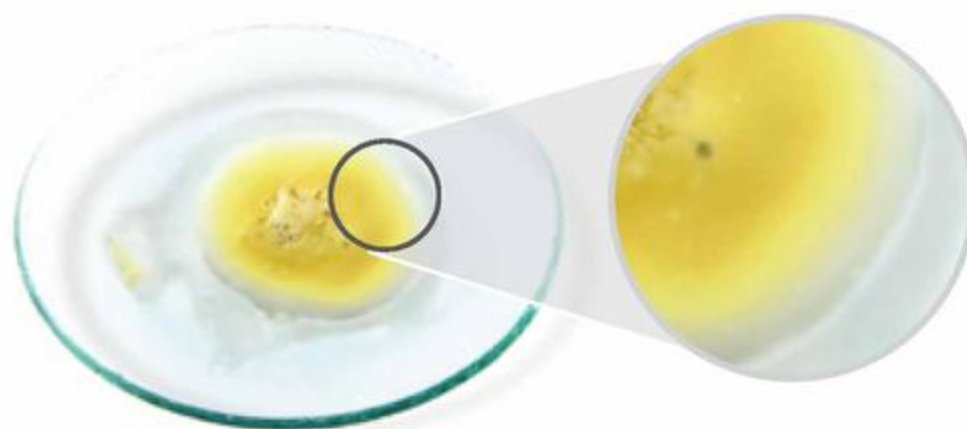
Fot. 17. Wpływ stężonego roztworu \text{HNO}_3 na białko.
