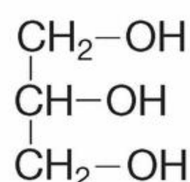
wzór półstrukturalny
