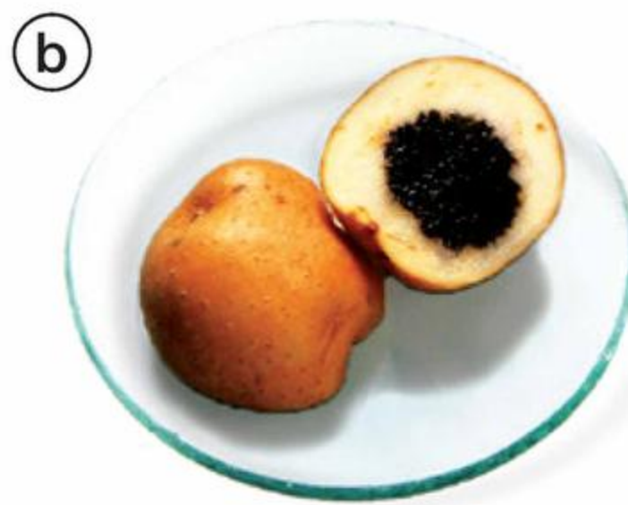
Fot. 156. Reakcja charakterystyczna skrobi – wykrywanie obecności skrobi w:
