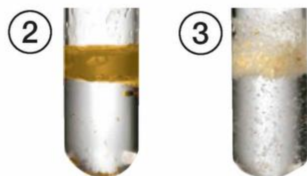
Fot. 117. Badanie rozpuszczalności w wodzie: kwasu stearynowego (2); kwasu oleinowego (3).
