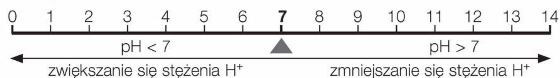
Rys. 2. Skala pH.
