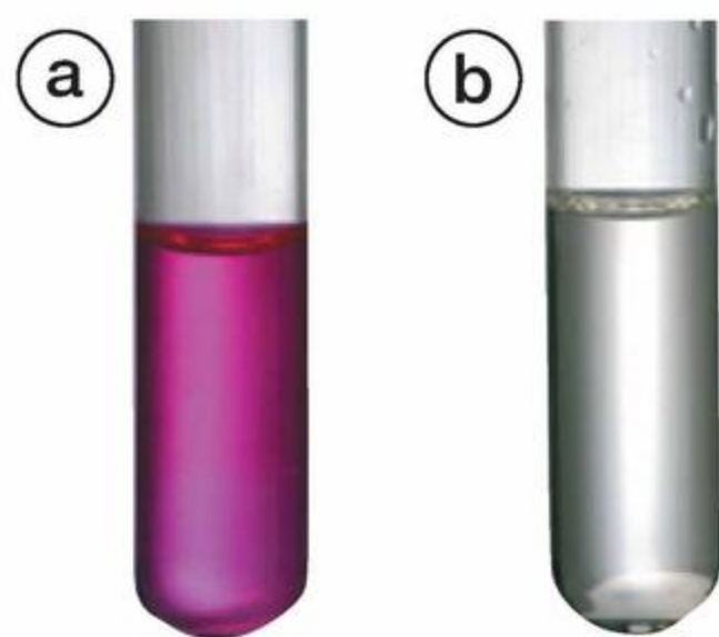
Fot. 38. Otrzymywanie soli: (a) roztwór NaOH z fenoloftaleiną; (b) odbarwienie fenoloftaleiny pod wpływem \text{HCl} i \text{H}_2\text{SO}_4 .
