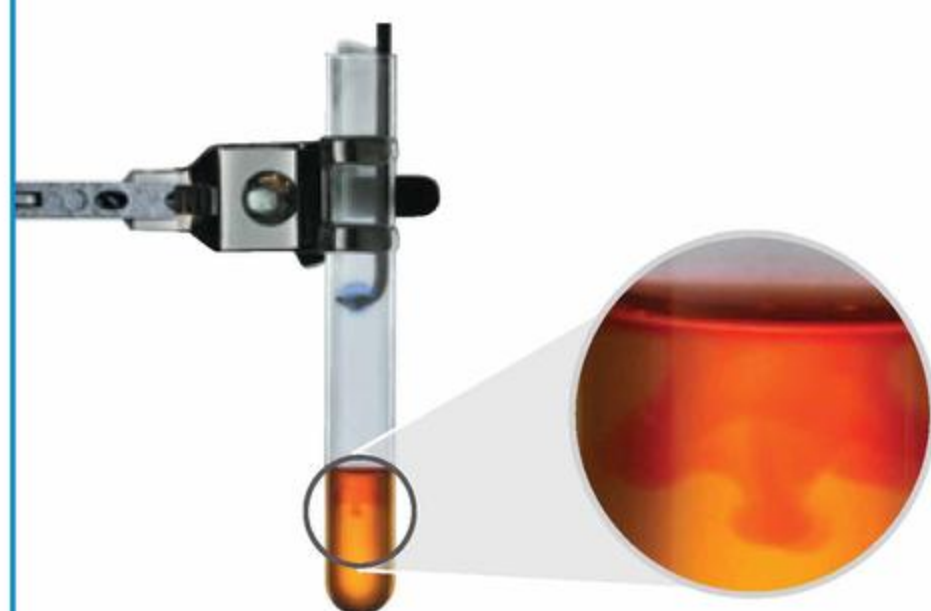
Fot. 9. Otrzymywanie kwasu siarkowego(IV).
