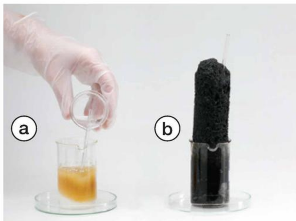
Fot. 144. Stężony roztwór kwasu siarkowego(VI) powoduje, że cukier żółknie (a), a potem pęcznieje i się zwęgla (b).
