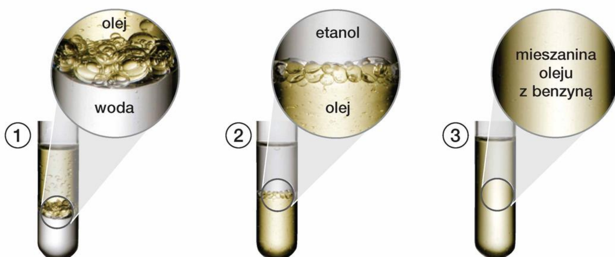
Fot. 131. Badanie rozpuszczalności oleju roślinnego w: wodzie ①, etanolu ②, benzynie ③.
