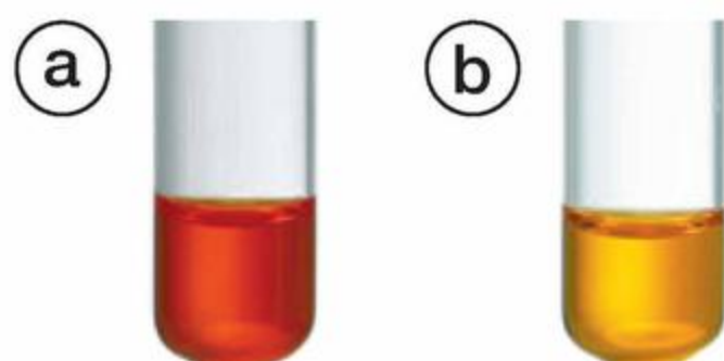
Fot. 10. Barwa roztworu przed ogrzaniem probówki (a) i po zakończeniu ogrzewania (b).
