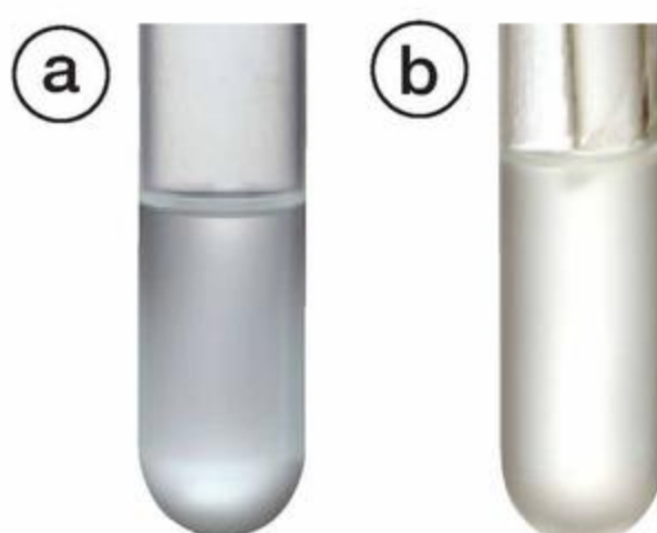
Fot. 155. Badanie rozpuszczalności skrobi: w zimnej wodzie (a), w gorącej wodzie (b).
