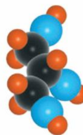
model cząsteczki
