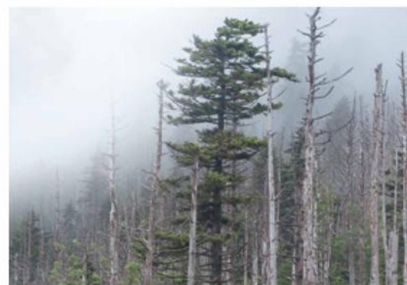
Fot. 26. Drzewa pobierają kwas też z chmur i mgły.
