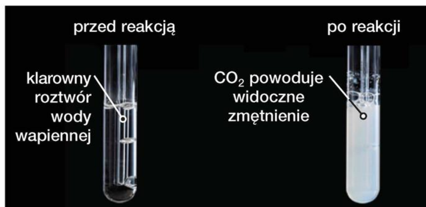
Fot. 48. Reakcja wody wapiennej z tlenkiem węgla(IV).
