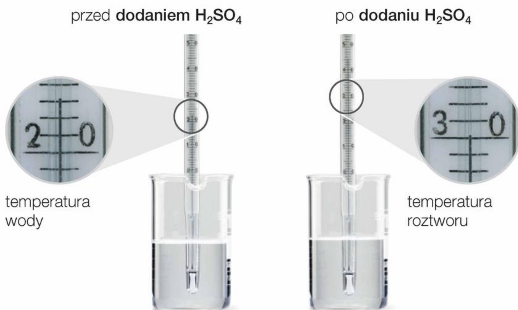
Fot. 13. Rozcieńczanie stężonego roztworu kwasu siarkowego(VI).
