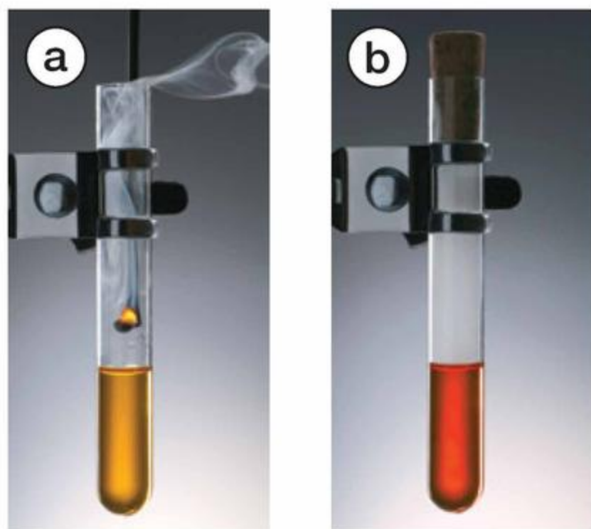
Fot. 21. Tlenek fosforu(V) powstaje w wyniku spalania fosforu czerwonego (a). Czerwona barwa wody z roztworem oranżu metylowego (b) świadczy o powstaniu kwasu fosforowego(V).
