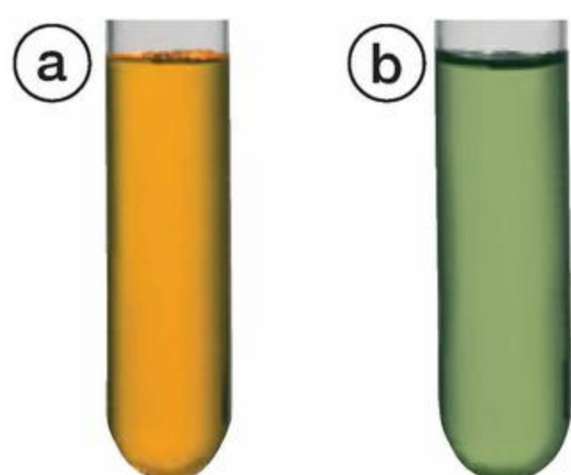
Fot. 97. Pomarańczowy roztwór dichromianu(VI) potasu (a) pod wpływem etanolu zmienia barwę na zieloną (b).
