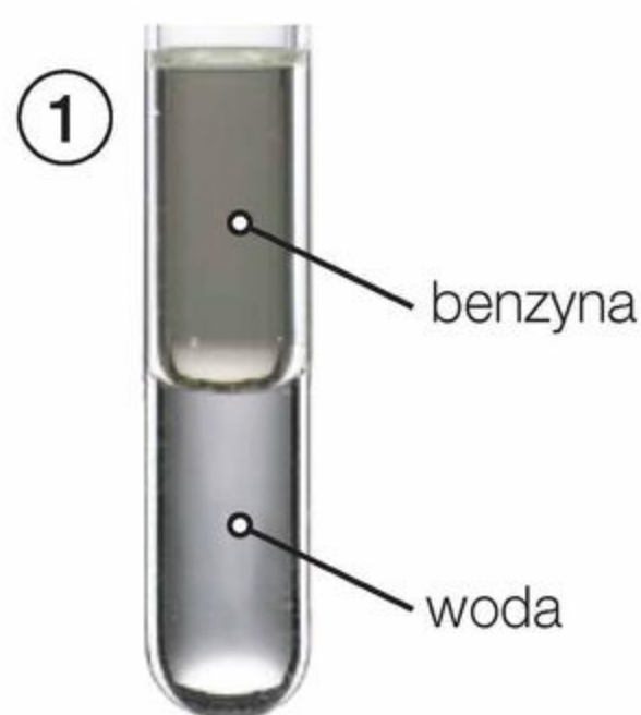
Fot. 76. Badanie palności benzyny i jej rozpuszczalności: w wodzie ① i oleju ②.
