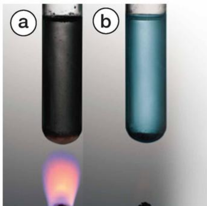
Fot. 114. Roztwór kwasu octowego z tlenkiem miedzi(II): przed ogrzewaniem (a); po ogrzewaniu (b).
