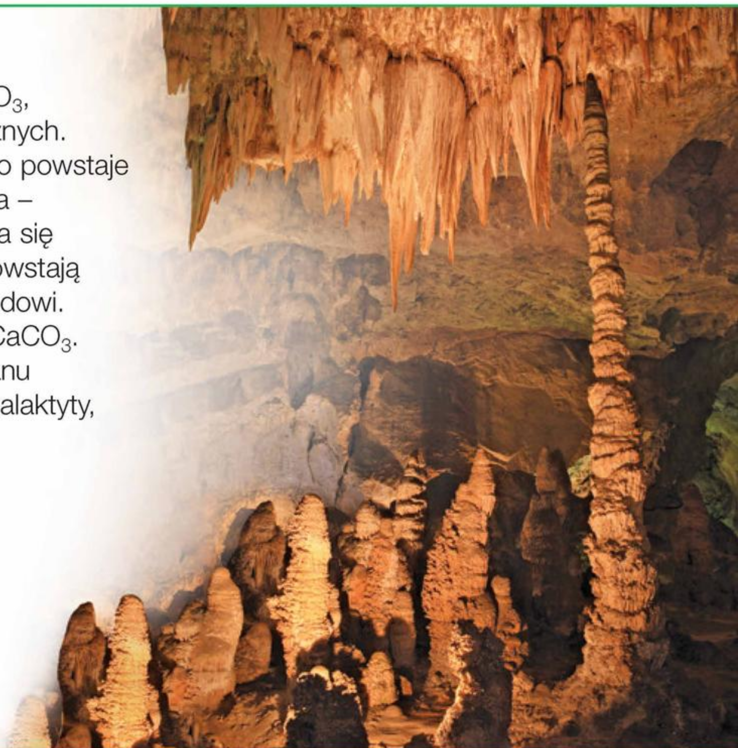
Fot. 62. Stalaktyty i stalagmity.
