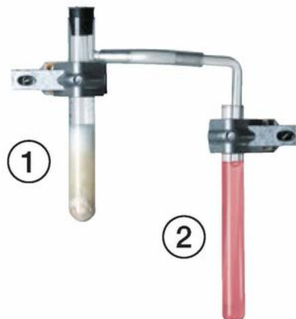
Fot. 18. Otrzymywanie \text{H}_2\text{CO}_3 .
