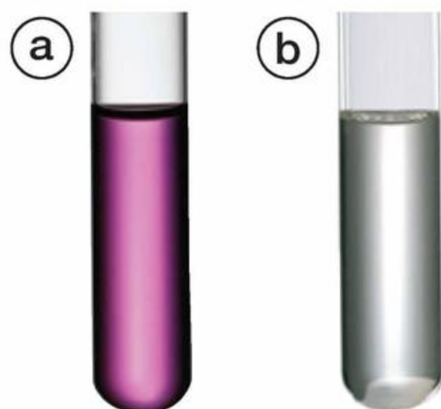
Fot. 113. Fenoloftaleina barwi się w zasadzie sodowej na malinowo (różowoczerwono) (a); pod wpływem CH 3 COOH następuje odbarwienie roztworu (b).
