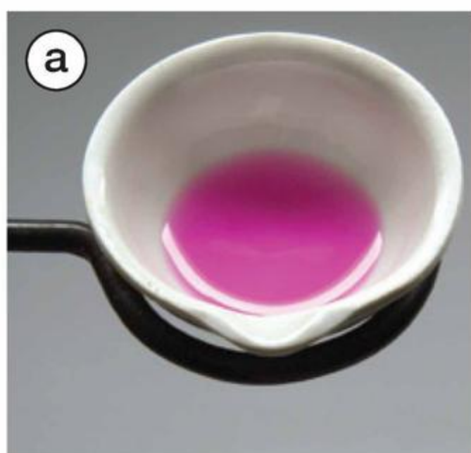
Fot. 119. Zawartość parownicy: przed dodaniem kwasu stearynowego (a), po dodaniu kwasu stearynowego (b).
