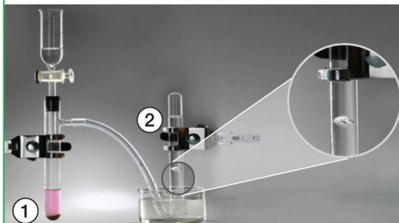
Fot. 82. Otrzymywanie etynu w reakcji karbidu z wodą.
