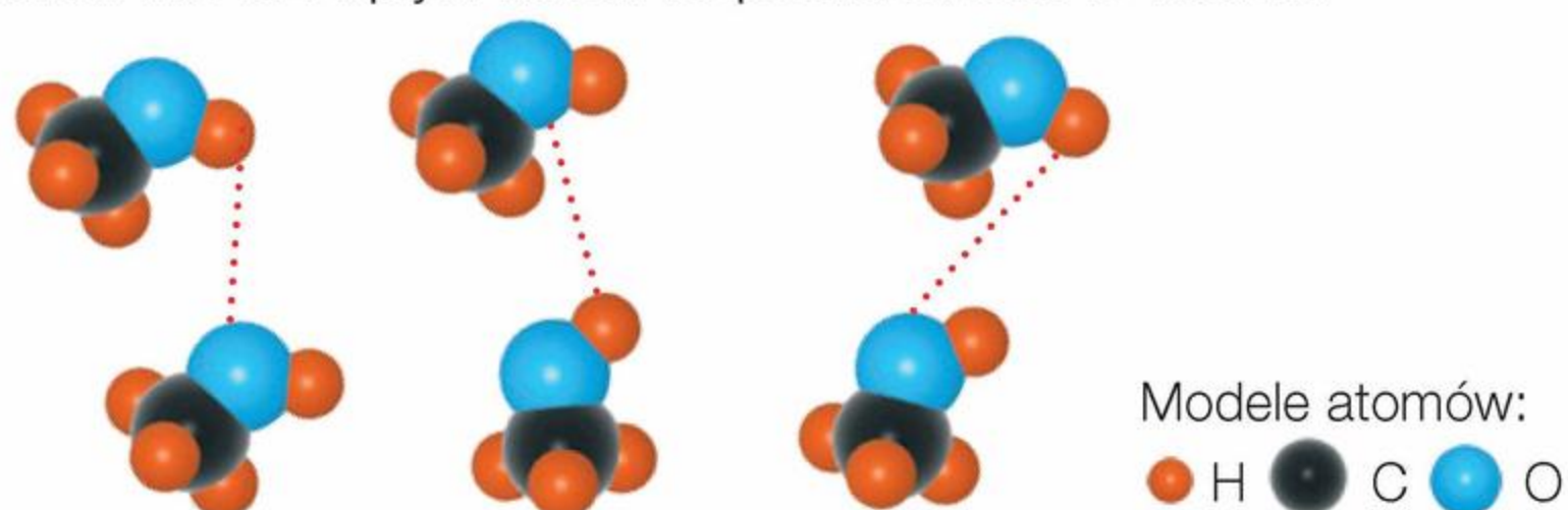
Rys. 8. Model wiązania, które powstaje między polarnymi cząsteczkami metanolu.
