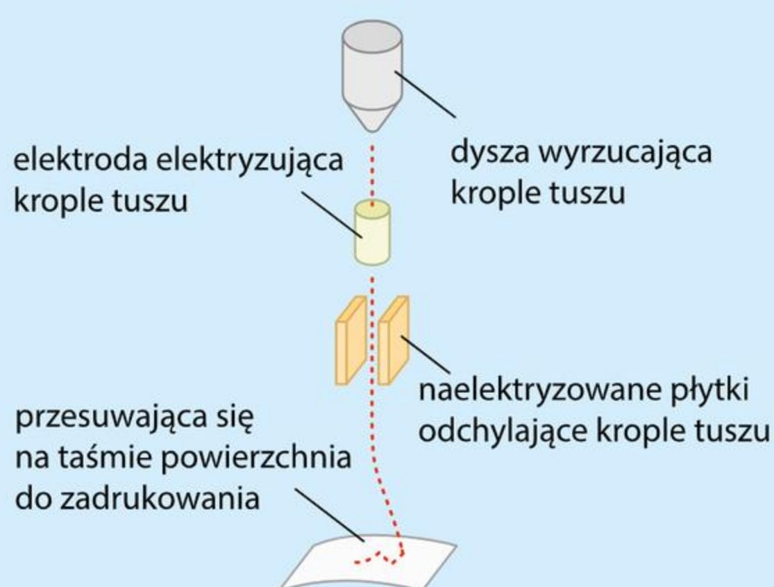
Schemat działania drukarki CIJ.
