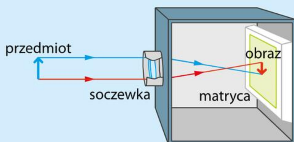
Powstawanie obrazu w aparacie fotograficznym.
