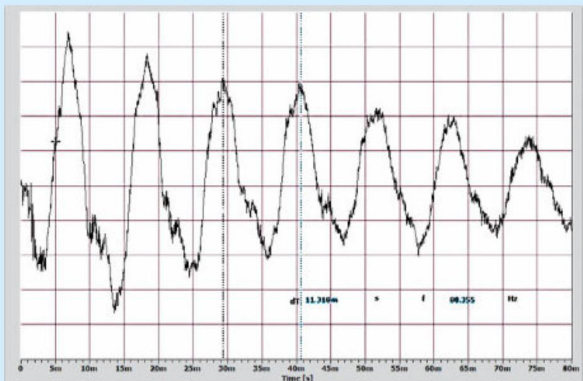
Przykładowy oscylogram uzyskany dla drgającej linijki.
