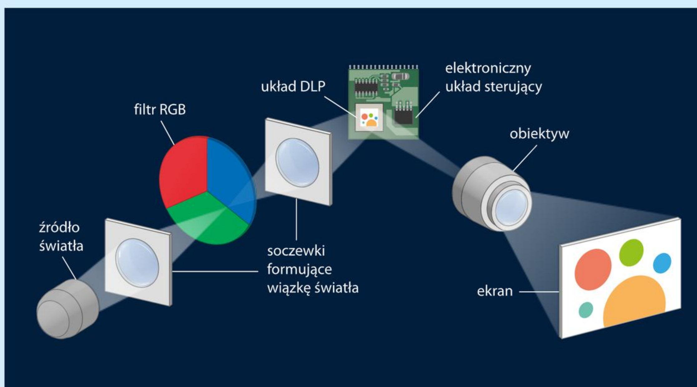
Schemat budowy i zasada działania projektora cyfrowego korzystającego z technologii DLP.
