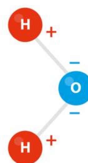
Cząsteczka wody.
