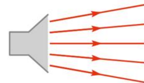
wiązka rozbieżna
