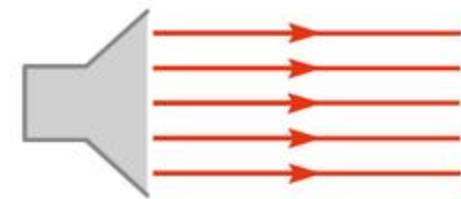
wiązka równoległa
