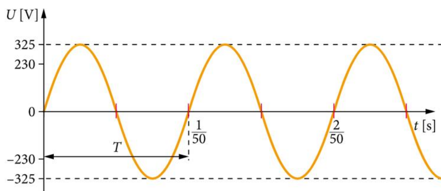
Zależność napięcia przemiennego od czasu.
