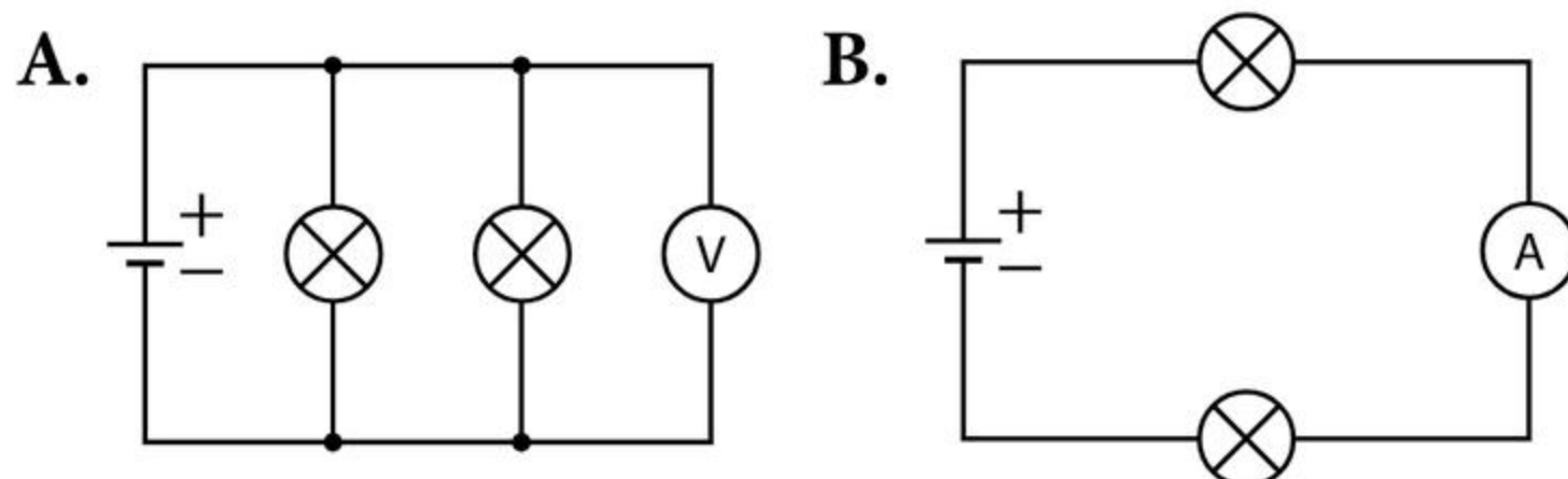
Przykładowe połączenie odbiorników energii (żarówek): A. równoległe, B. szeregowo.
