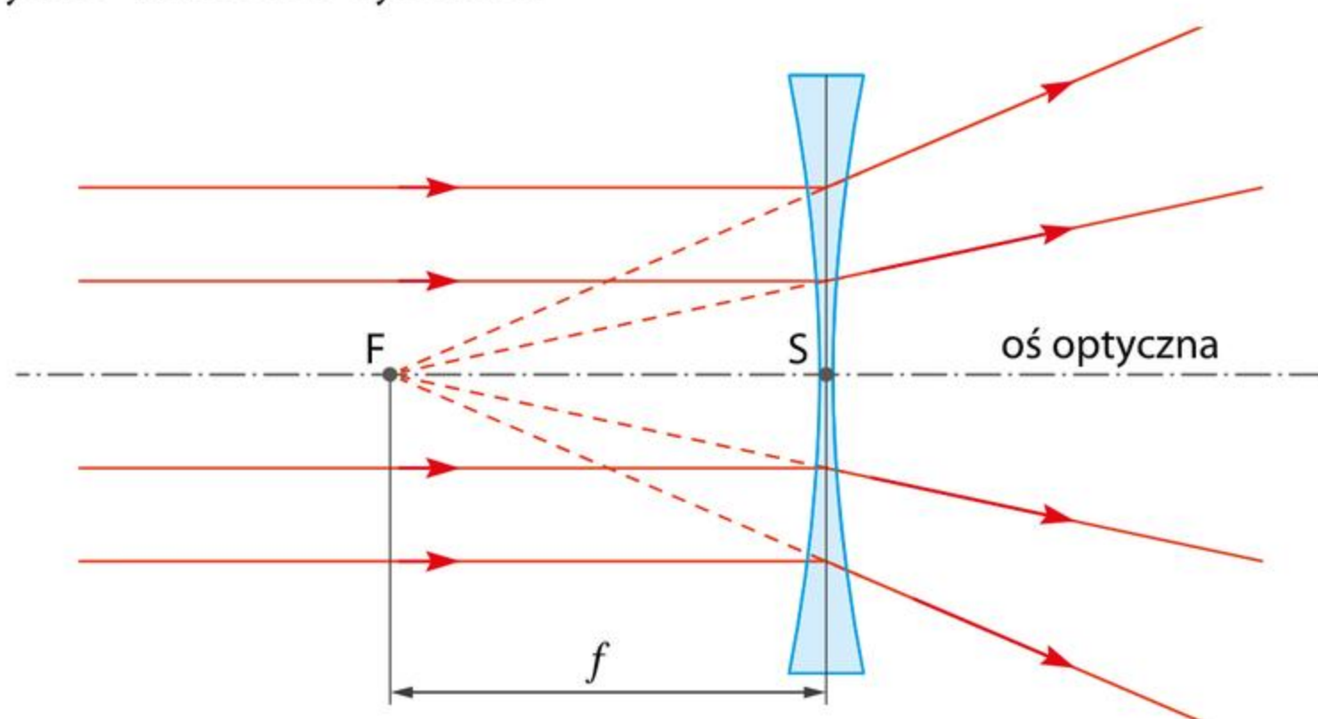
Konstrukcja ogniska pozornego soczewki rozpraszającej.
