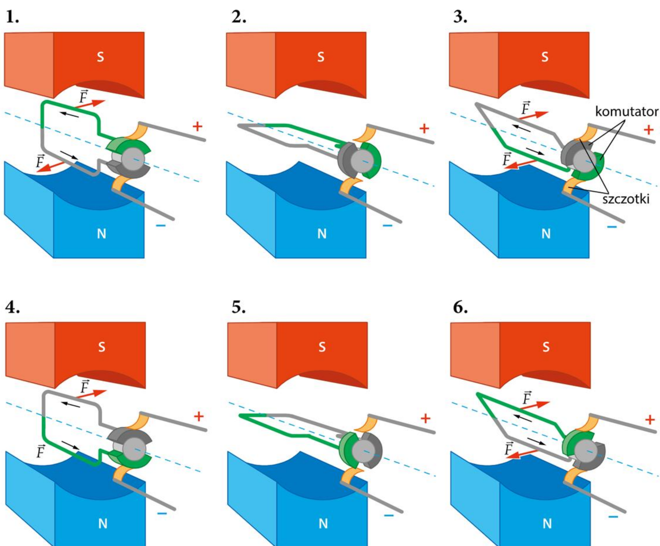
Schemat działania silnika elektrycznego.
