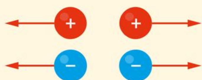
Ładunki jednoimienne (tego samego znaku) odpychają się.
