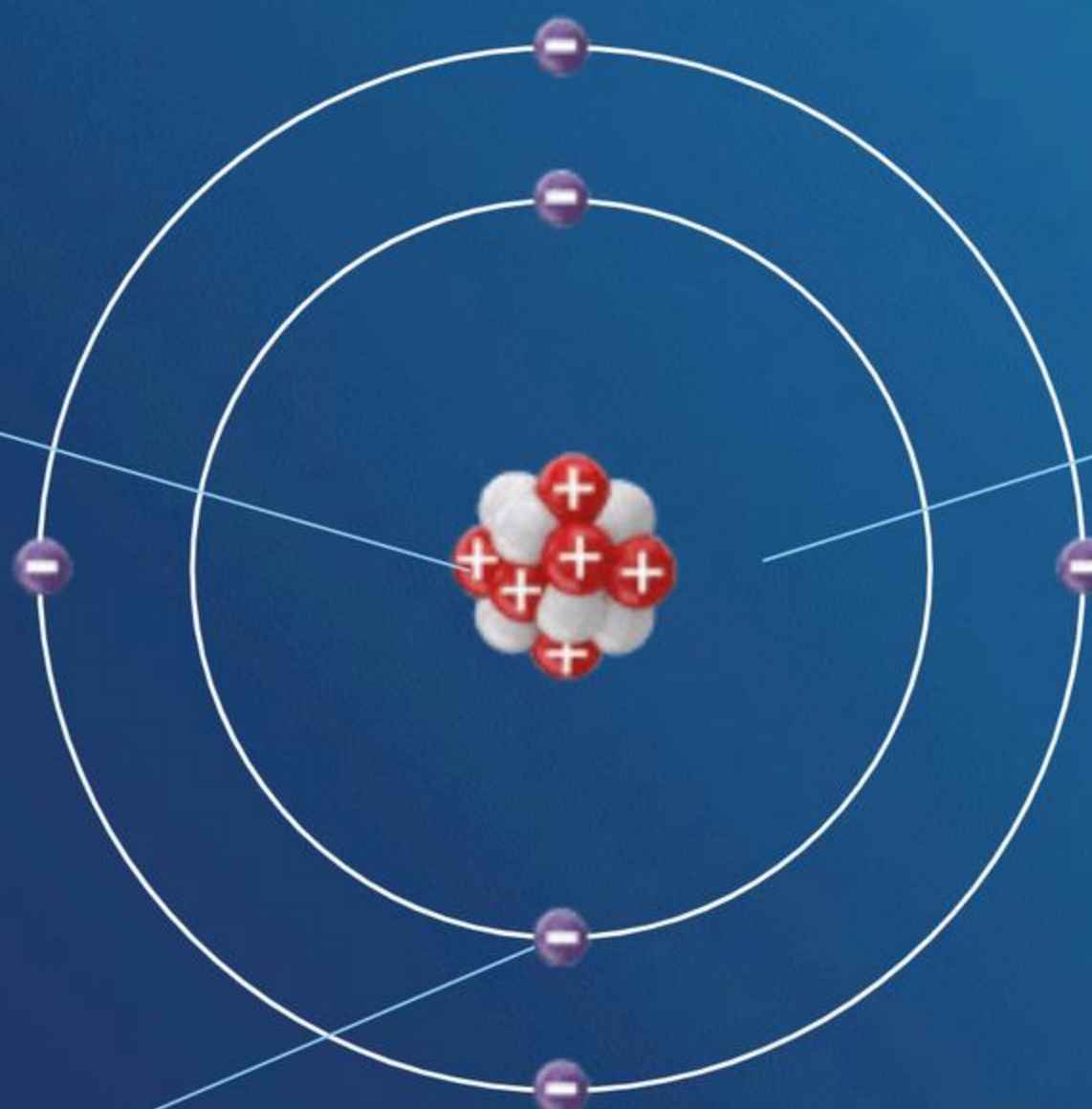
Uproszczony model atomu węgla.
