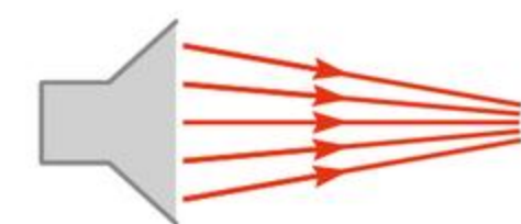
wiązka zbieżna
