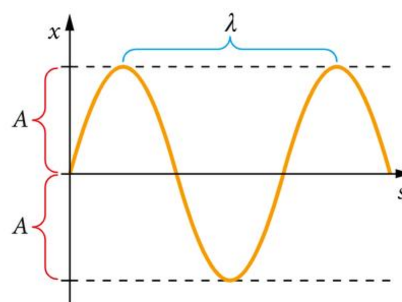
Długość fali \lambda to odległość między kolejnymi grzbietami.
