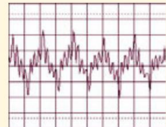
✂ Dźwięk gitary.
