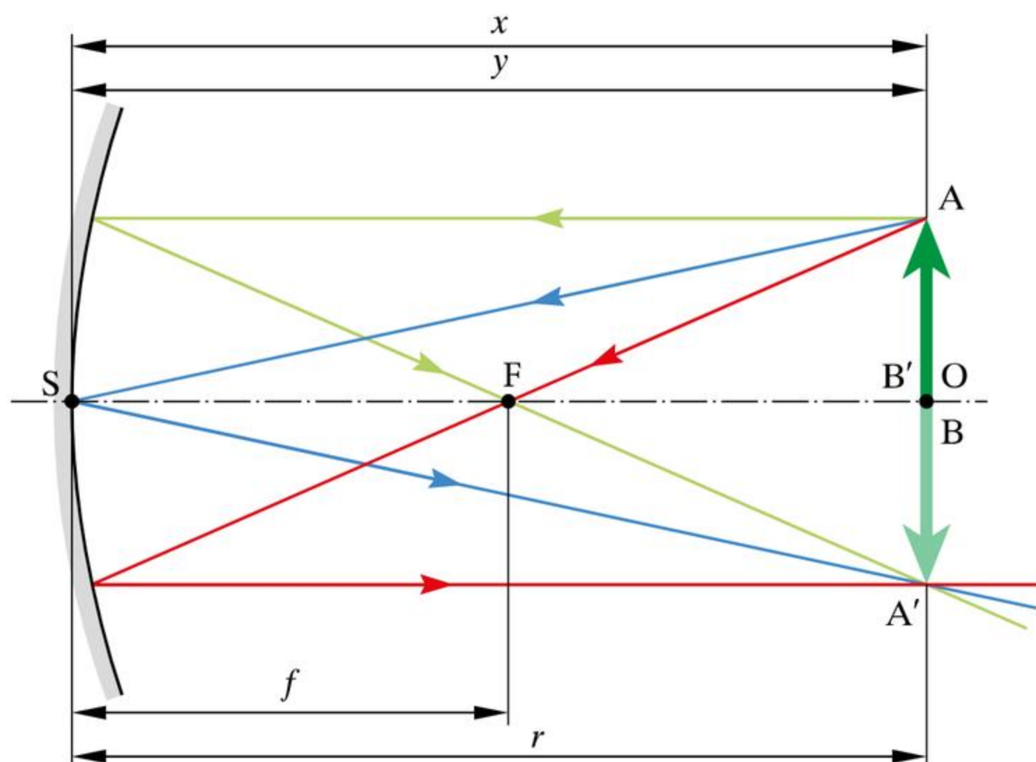
Konstrukcja obrazu dla x = r .
