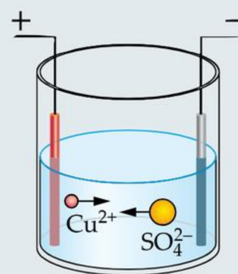
Schemat galwanizacji.
