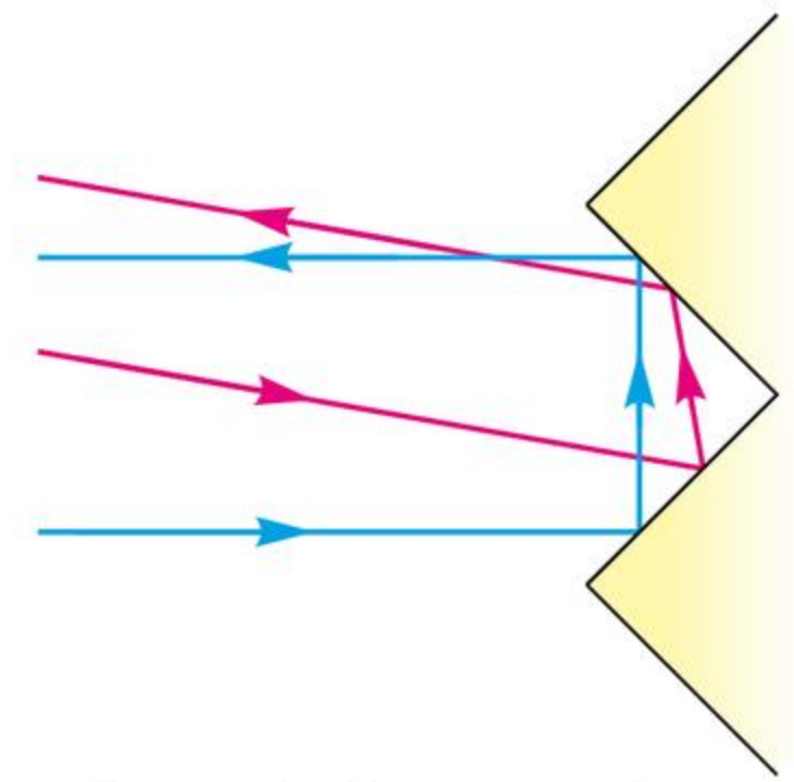
Schemat działania światelka odblaskowego.
