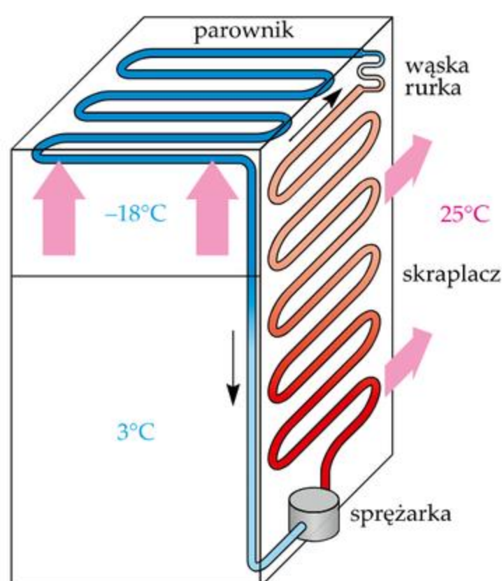
Schemat działania lodówki.
