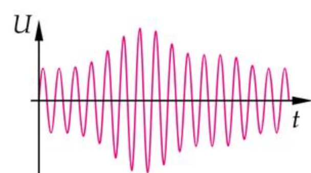
Modulacja amplitudy (AM).
