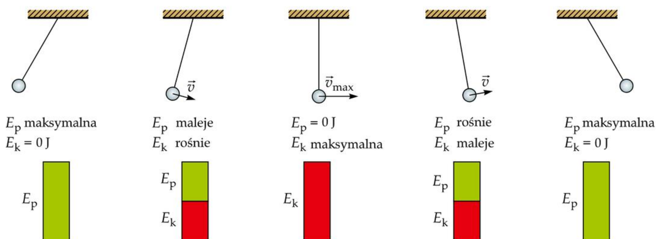
Diagram przedstawia przemiany energii kinetycznej E_k i energii potencjalnej E_p w ruchu wahadła.
