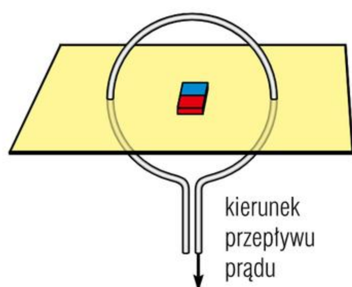
Najprostszy elektromagnes.
