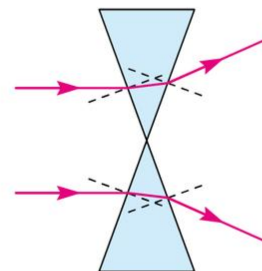
Soczewka wklęsła – rozpraszająca.
