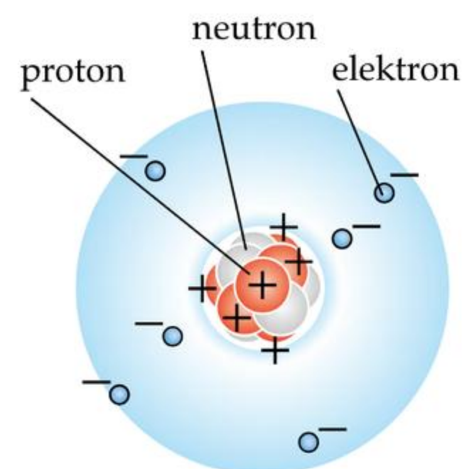
Budowa atomu.
