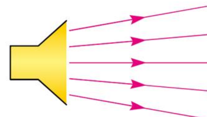
Wiązka rozbieżna.
