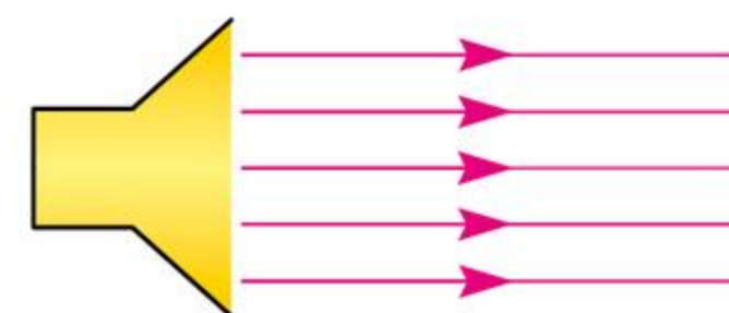
Wiązka równoległa.
