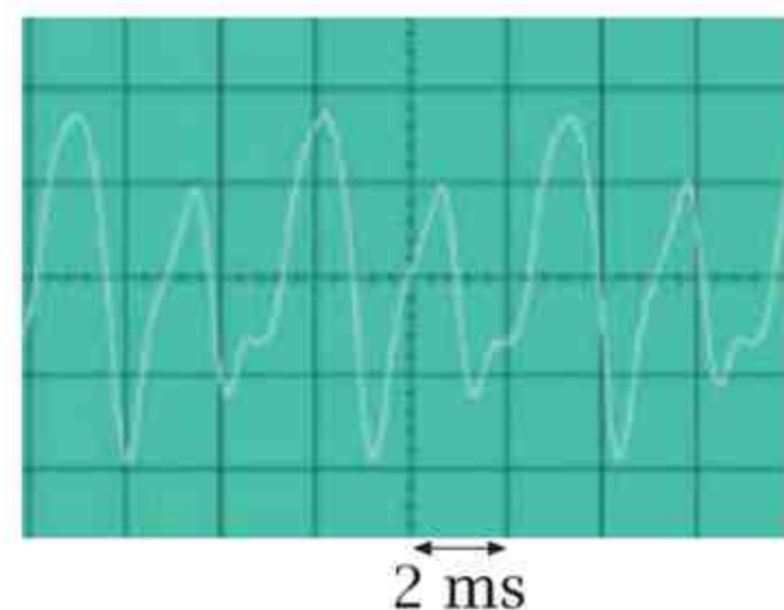
Oscylogram dźwięku powstałego na gitarze.
