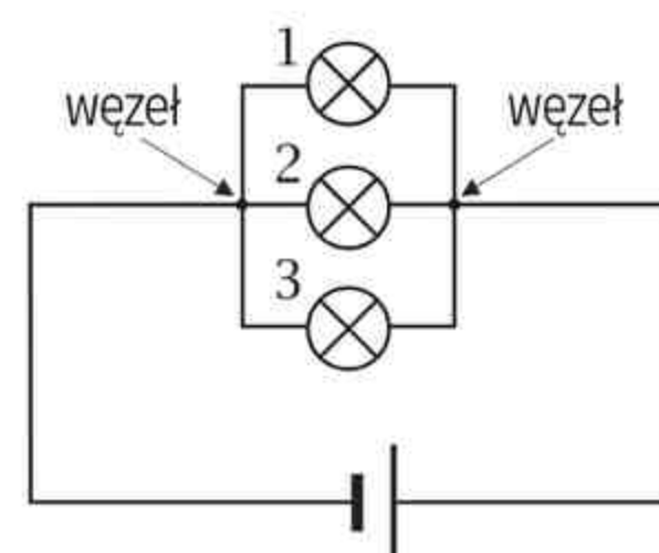
Trzy żarówki połączone równoległe.
