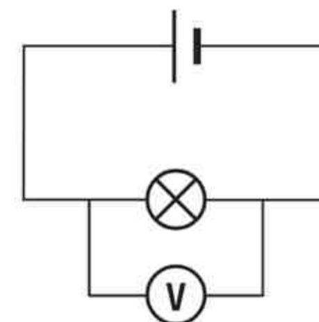
Sposób połączenia woltomierza z obwodem.
