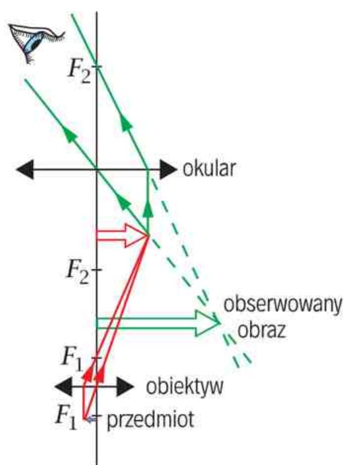
Schemat działania mikroskopu.
