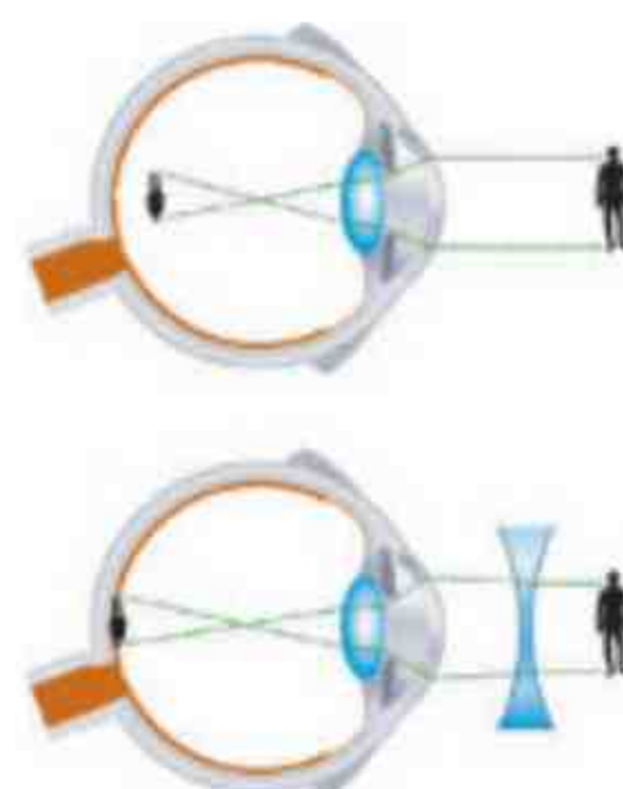
Krótkowzroczność.
