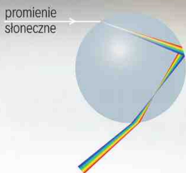
Rozszczepienie światła w kropli wody.
