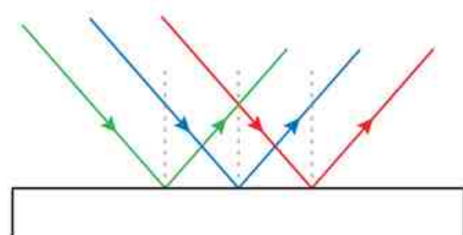
Promienie równoległe odbite od zwierciadła płaskiego.
