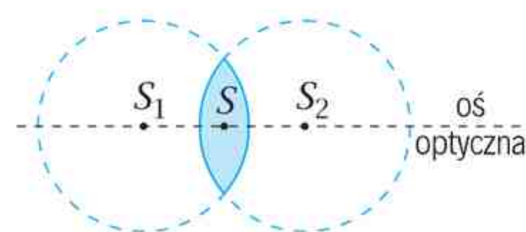
Soczewka dwuwypukła.
