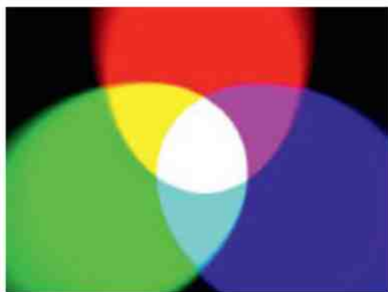
Mieszanie się światła w systemie RGB.
