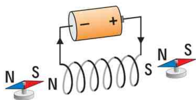
Bieguny magnetyczne zwojnicy można określić, używając igły magnetycznej.
