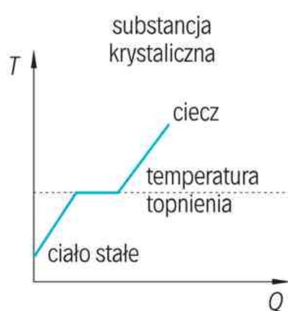
Zależność temperatury T porcji substancji od dostarczonego ciepła Q .
