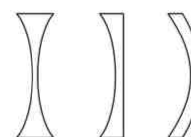
Soczewki wklęsłe, rozpraszające w powietrzu.
