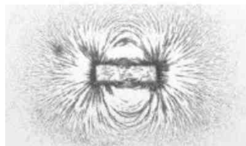
Małe igły magnetyczne lub opiłki żelaza rozsypane w okolicy magnesu ustawiają się wzdłuż linii pola magnetycznego.
