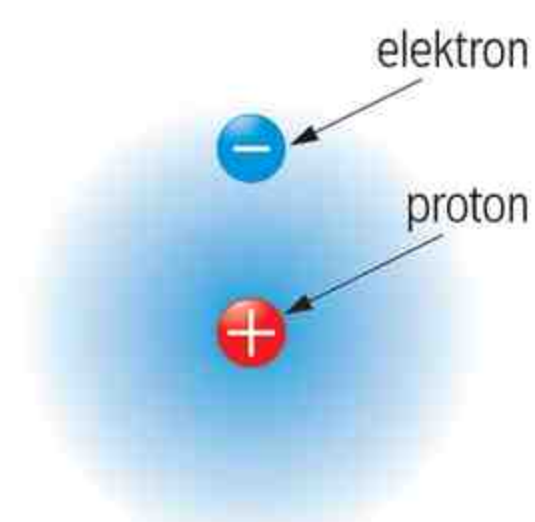
Atom wodoru.
