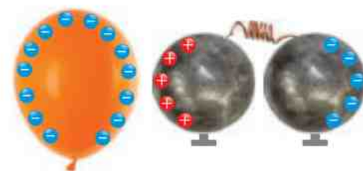
Kule połączone przewodem.
