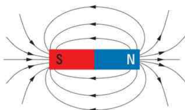
Linie pola magnetycznego wokół magnesu sztabkowego.
