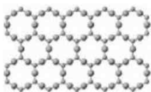
Struktura krystaliczna.
