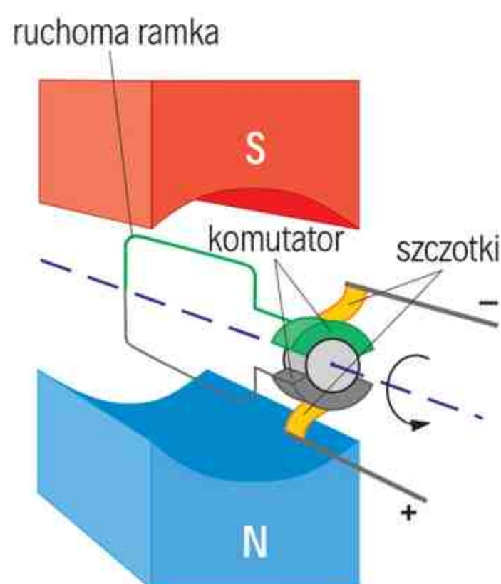
Komutator w modelu silnika. Ramka (zwoj) z prądem ciągle obraca się przeciwnie do ruchu wskazówek zegara.
