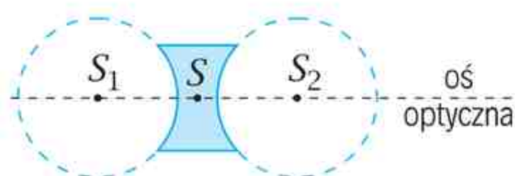
Soczewka dwuwklęsła.
