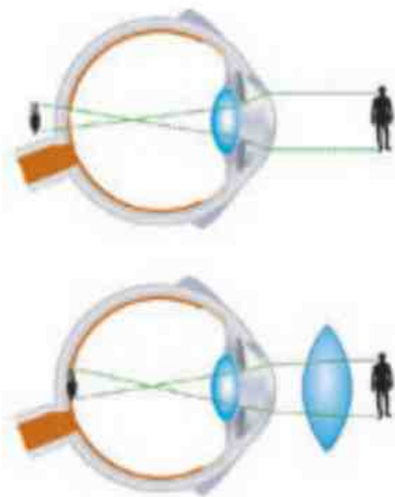
Dalekowzroczność.
