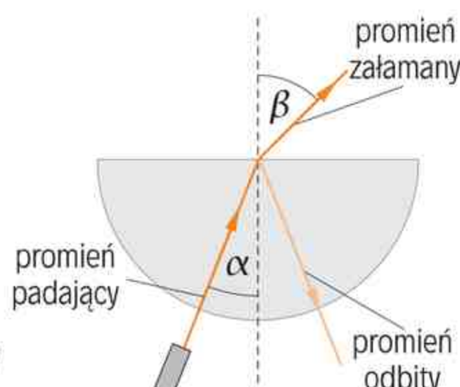
Przejście światła ze szkła do powietrza.
