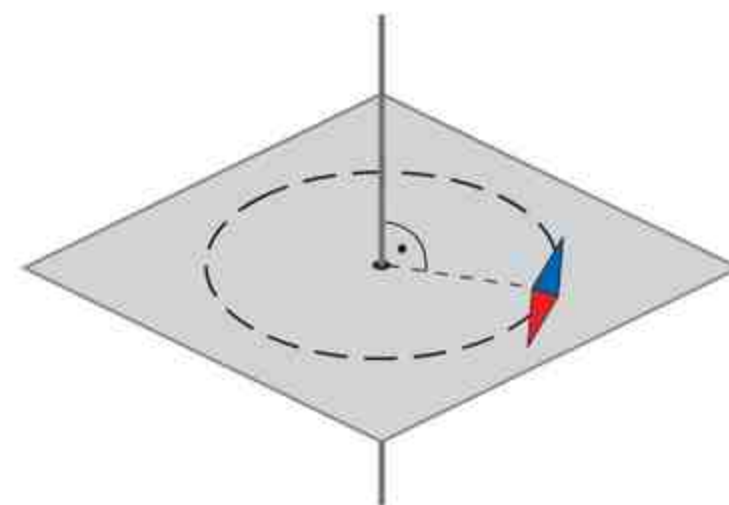
Ustawienie igły magnetycznej w pobliżu przewodnika z prądem.
