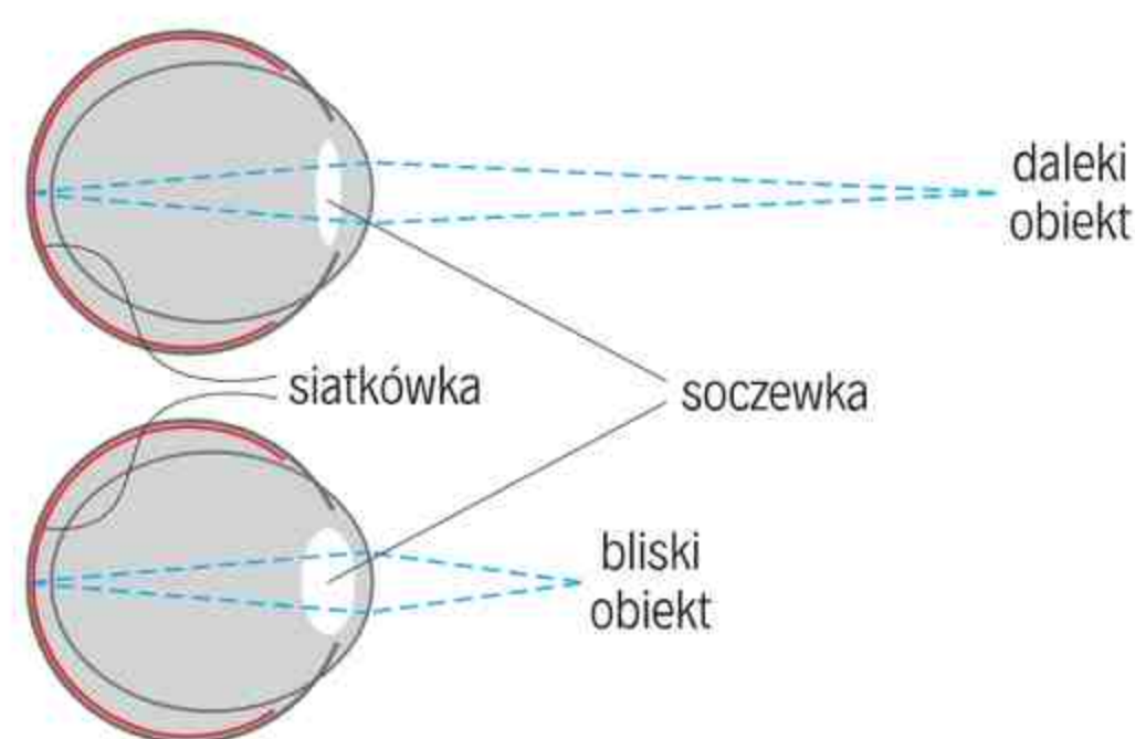
Akomodacja.
