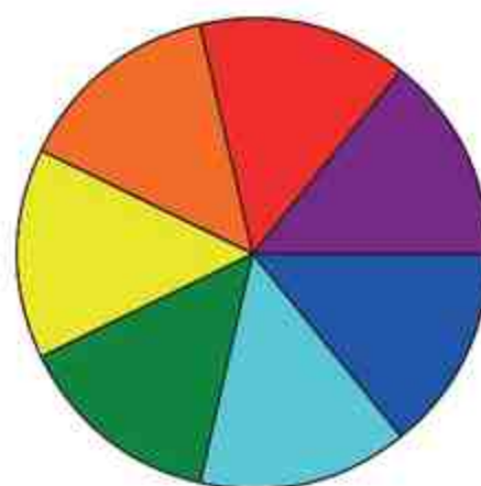
Krążek Newtona.
