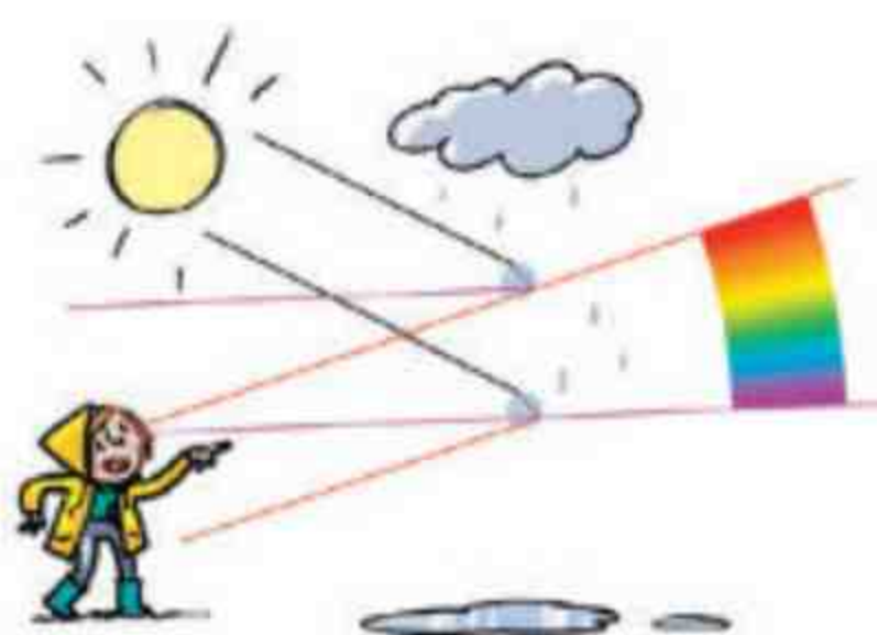
Schemat powstawania tęczy widzianej przez obserwatora.
