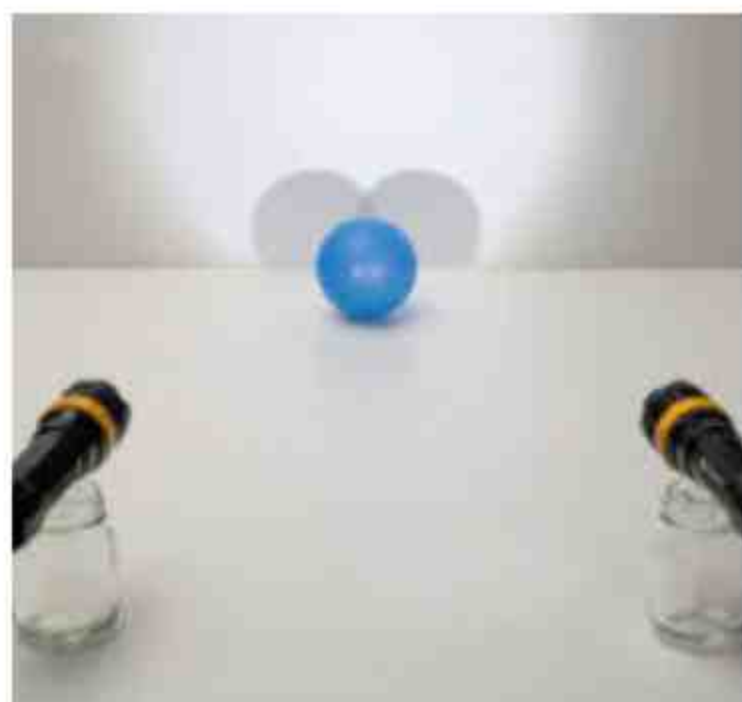
Cień oraz półcień.
