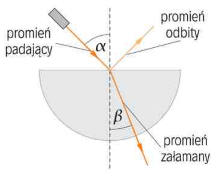
Przejście światła z powietrza do szkła.
