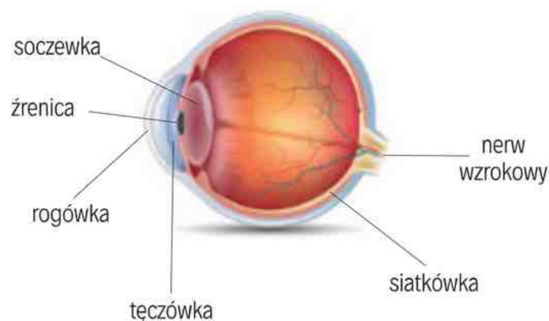
Budowa oka.
