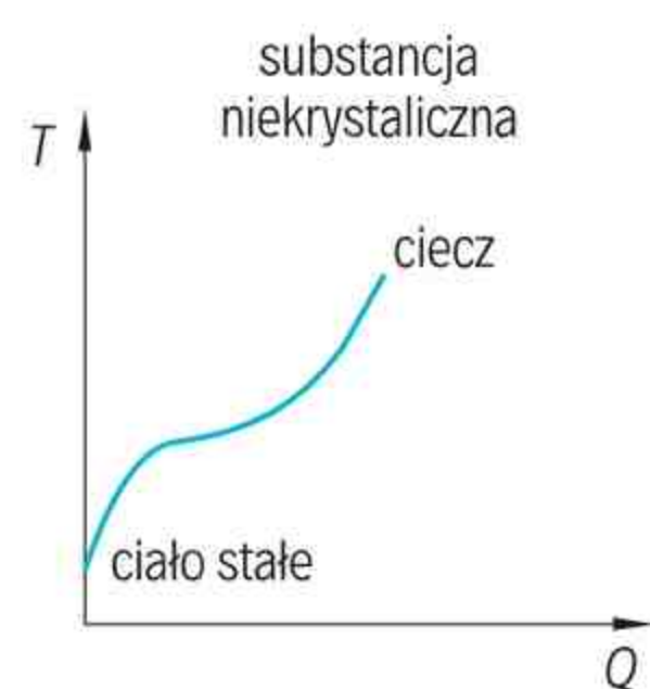
Zależność temperatury T porcji substancji od dostarczonego ciepła Q .
