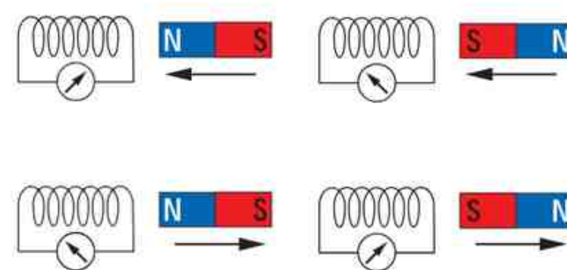
Zbliżanie i oddalanie magnesu wytwarza prąd elektryczny w zwojnicy.
