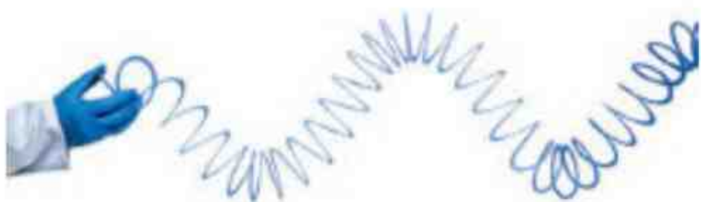
Fala poprzeczna w sprężynie.
