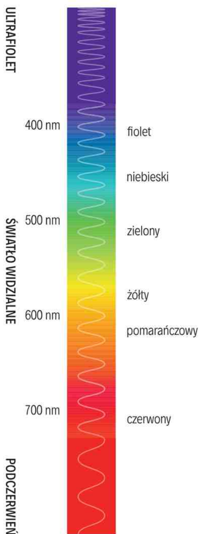
Widmo światła białego. Długość fal w próżni.
