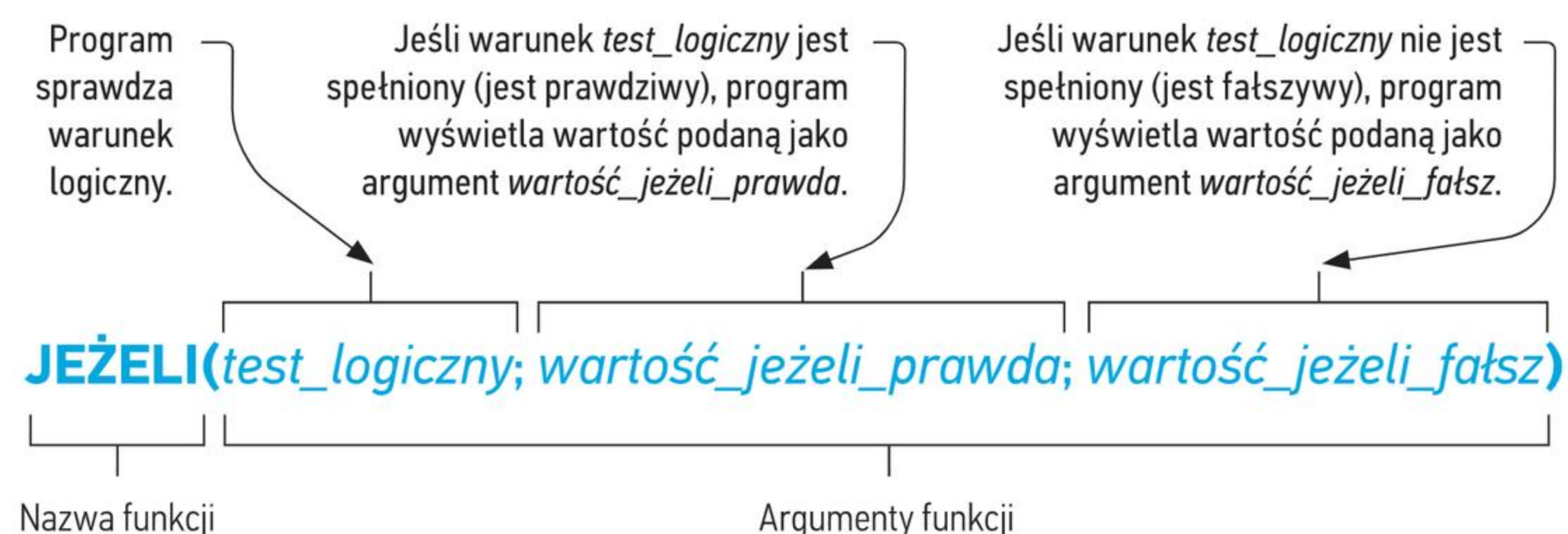
Rys. 5. Ogólna postać funkcji JEŻELI
