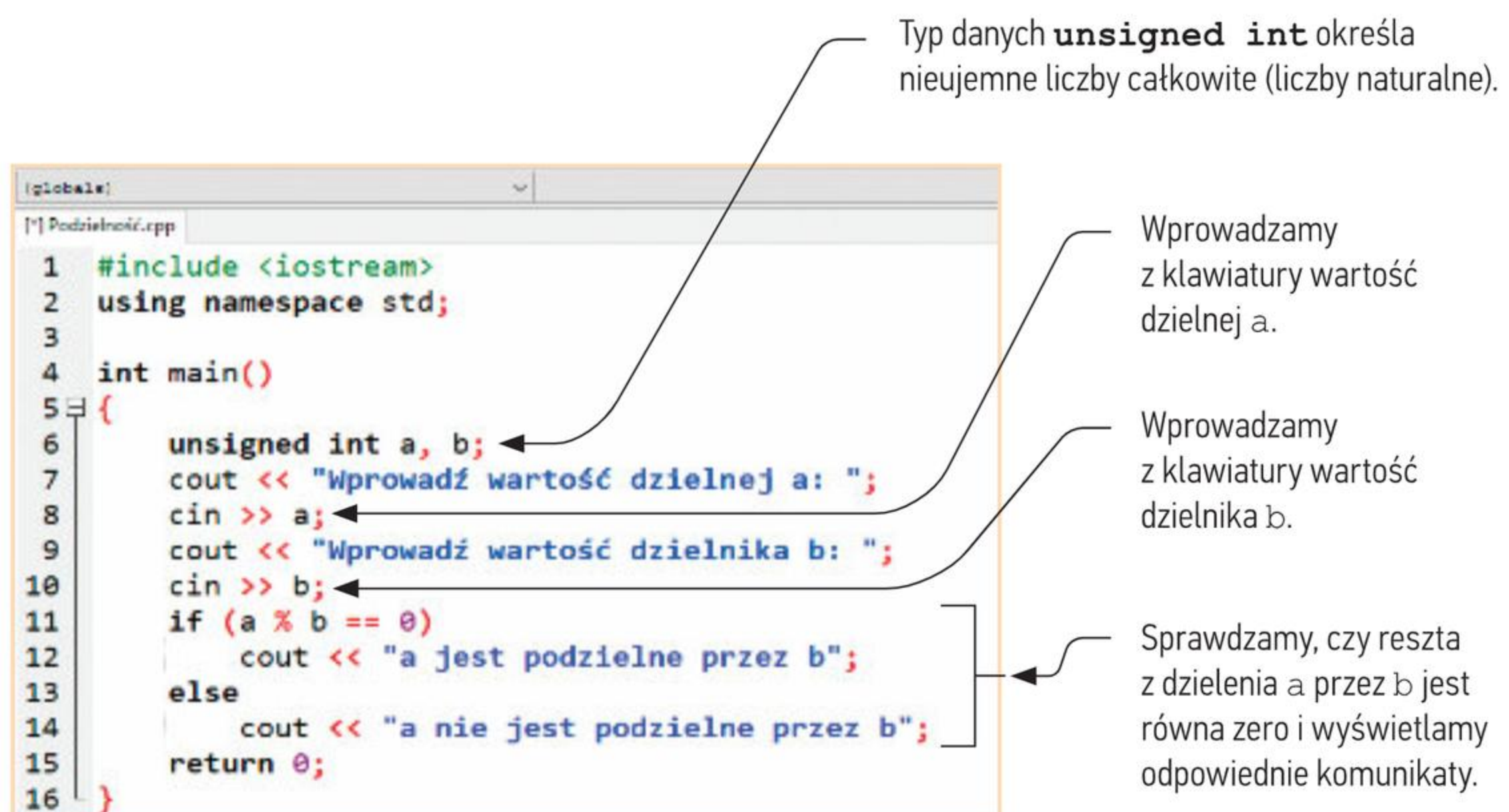
Rys. 3. Program w języku C++ realizujący algorytm badania podzielności liczb naturalnych
