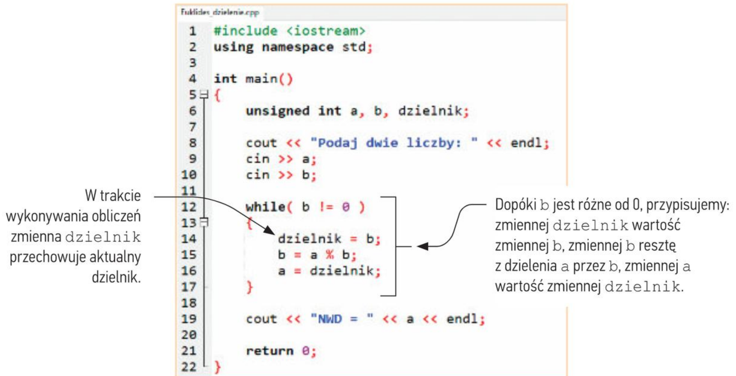
Rys. 8. Program w języku C++ realizujący algorytm Euklidesa w wersji z resztą z dzielenia
