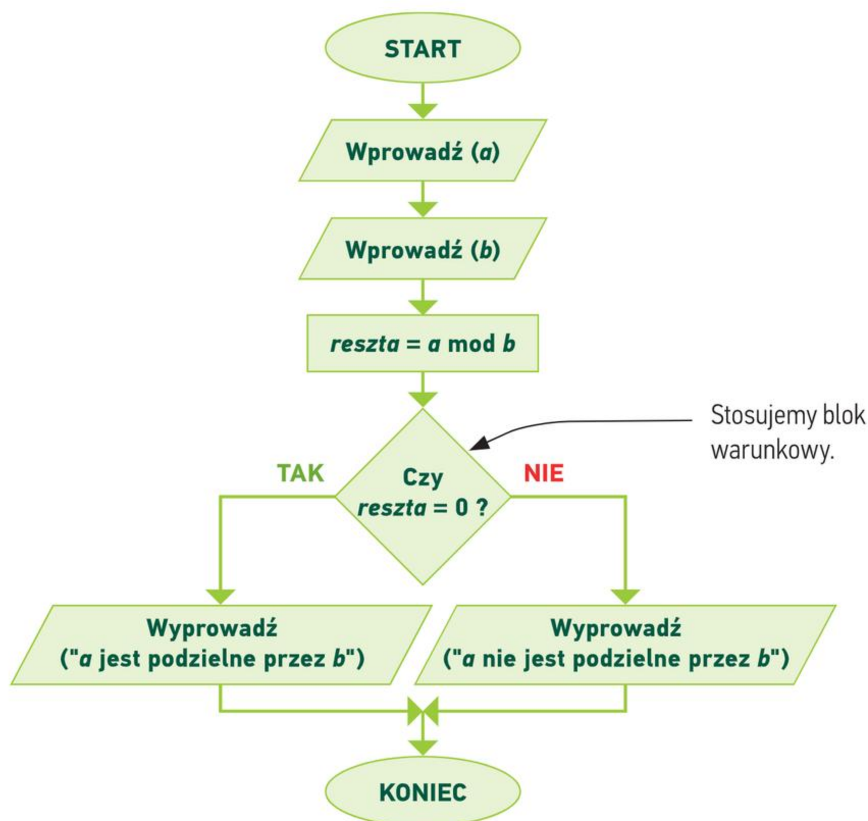
Rys. 2. Schemat blokowy algorytmu badania podzielności liczb
