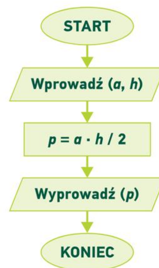
Rys. 2. Schemat blokowy algorytmu obliczania pola trójkąta
