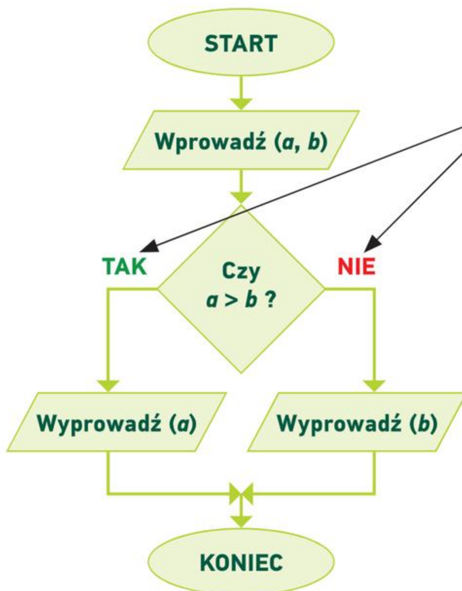
Rys. 4. Schemat blokowy algorytmu z warunkiem – ćwiczenie 5.
