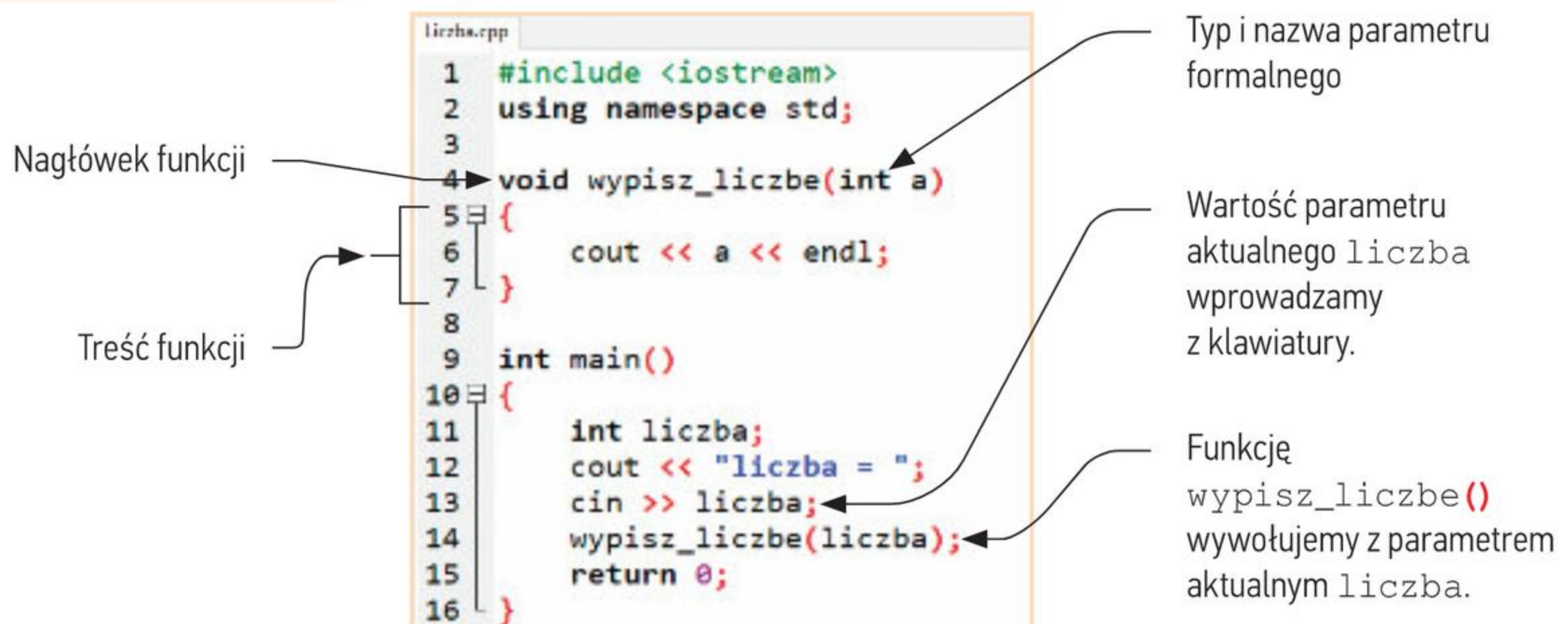
Rys. 11. Przykład definicji funkcji niezwracającej wartości w języku C++ – ćwiczenie 8.
