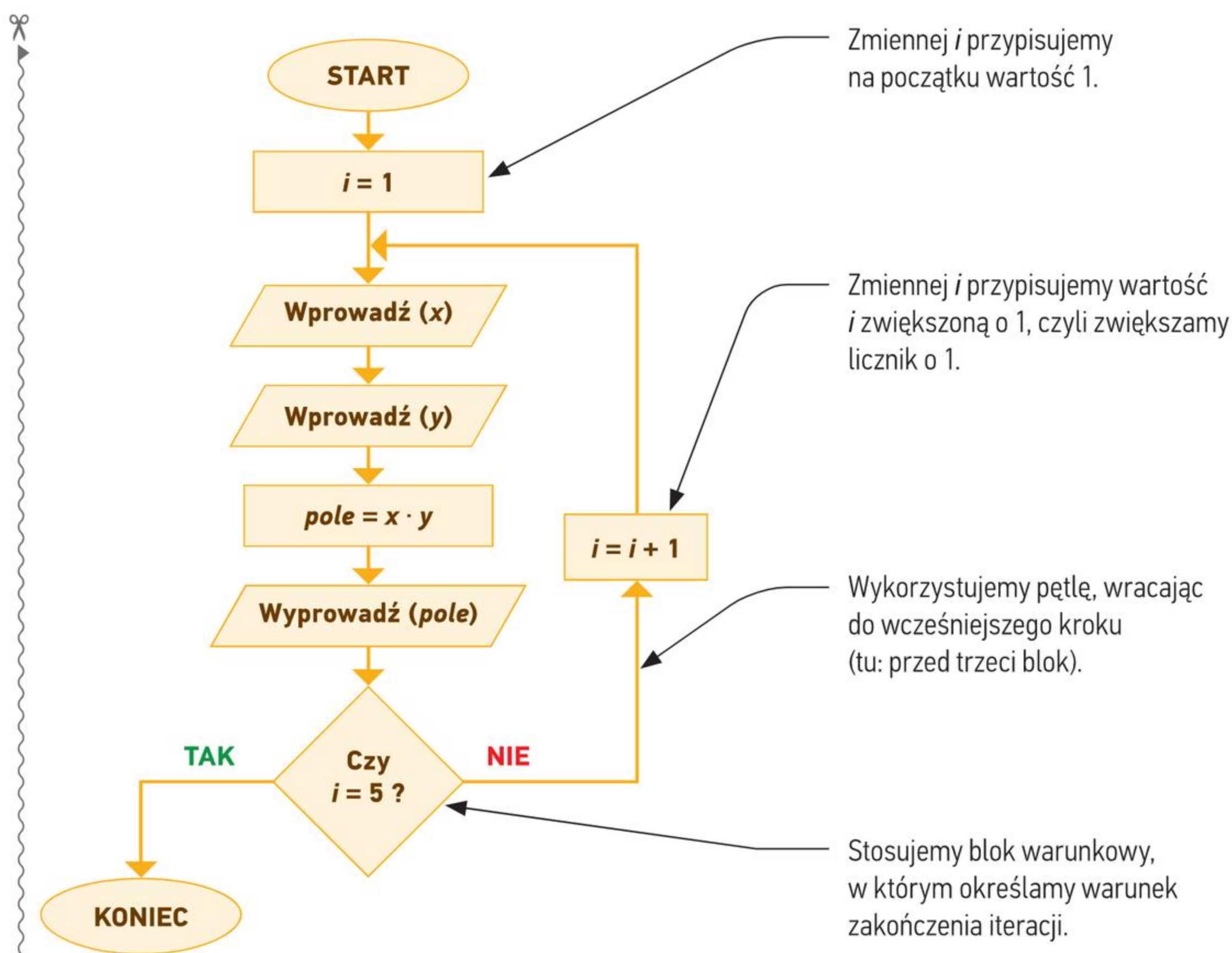
Rys. 7. Schemat blokowy algorytmu iteracyjnego – ćwiczenie 6.
