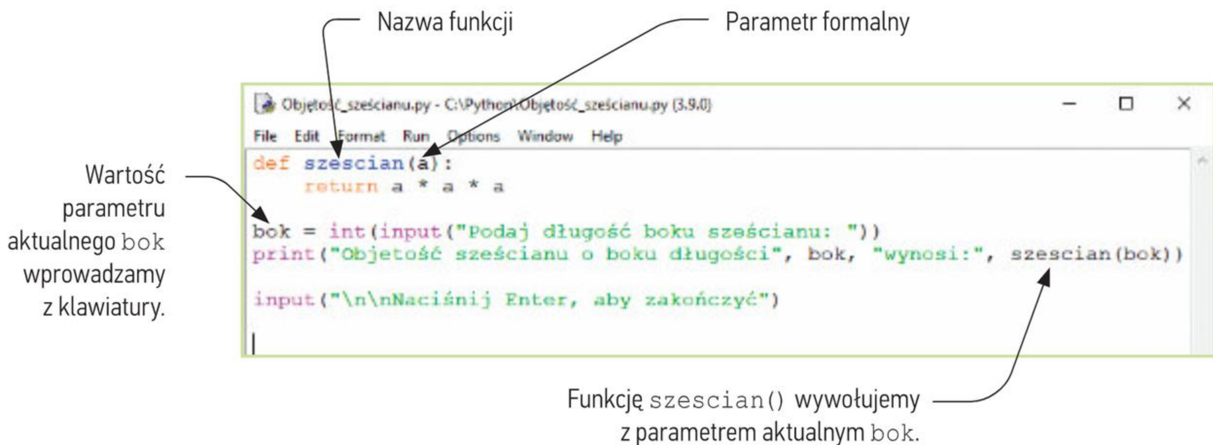
Rys. 12. Program w języku Python, w którym zdefiniowano funkcję zwracającą wartość z jednym parametrem – ćwiczenie 11.
