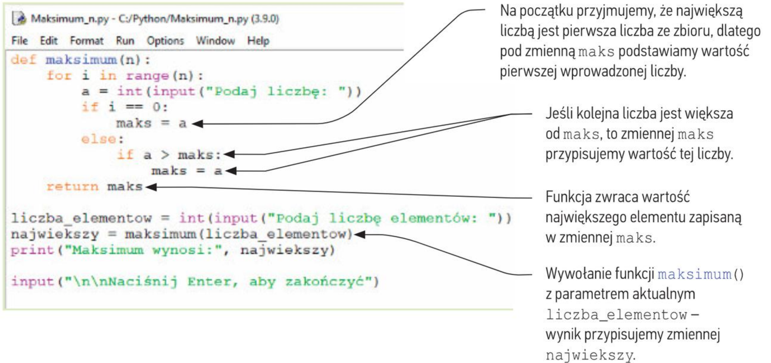
Rys. 2. Program w języku Python realizujący algorytm wyszukiwania największej liczby w zbiorze n -elementowym – ćwiczenie 3.
