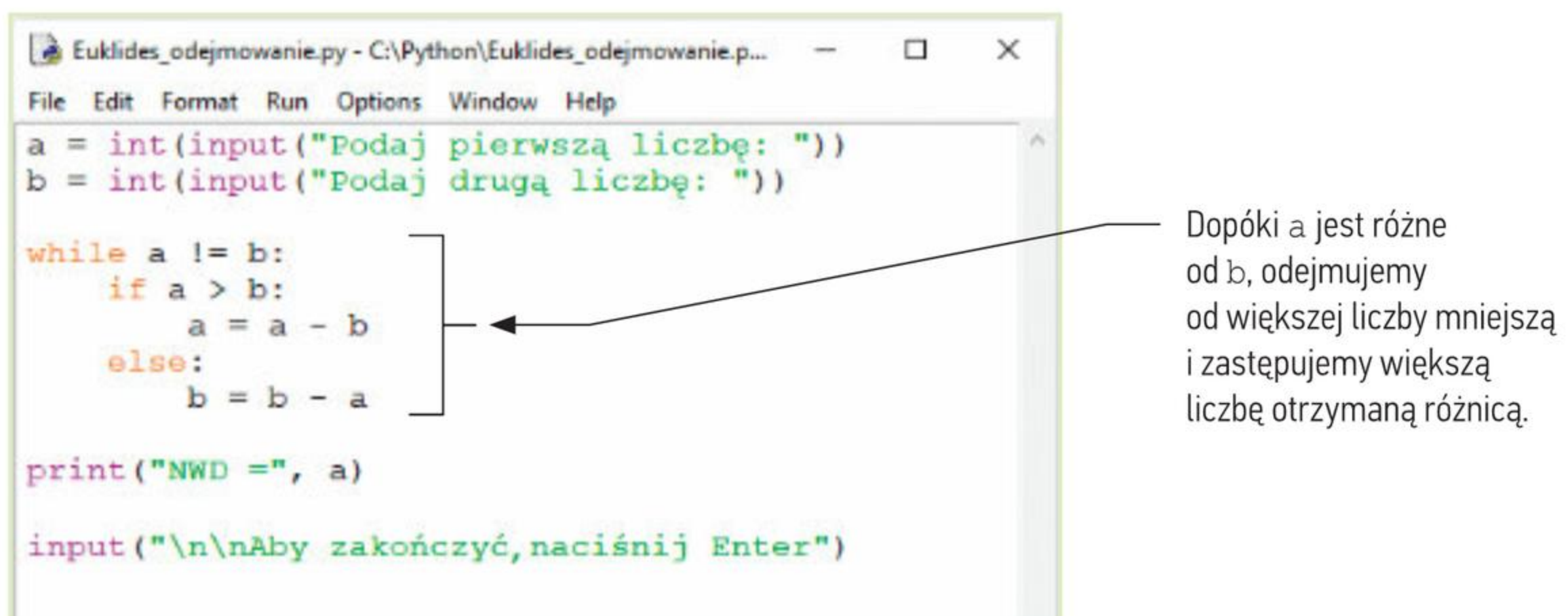
Rys. 7. Program w języku Python realizujący algorytm Euklidesa w wersji z odejmowaniem
