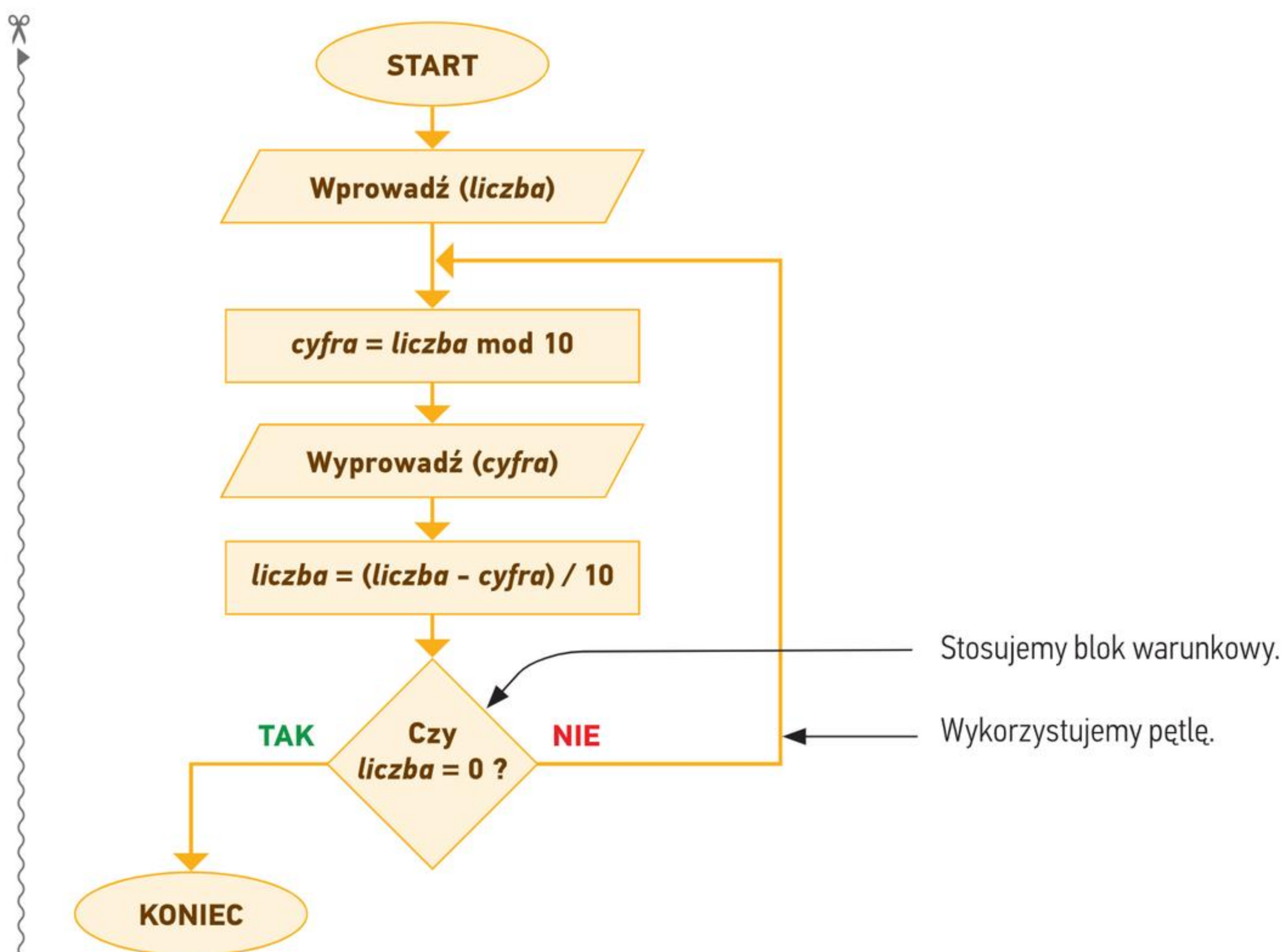
Rys. 9. Schemat blokowy algorytmu wyodrębniania cyfr danej liczby od cyfry jedności
