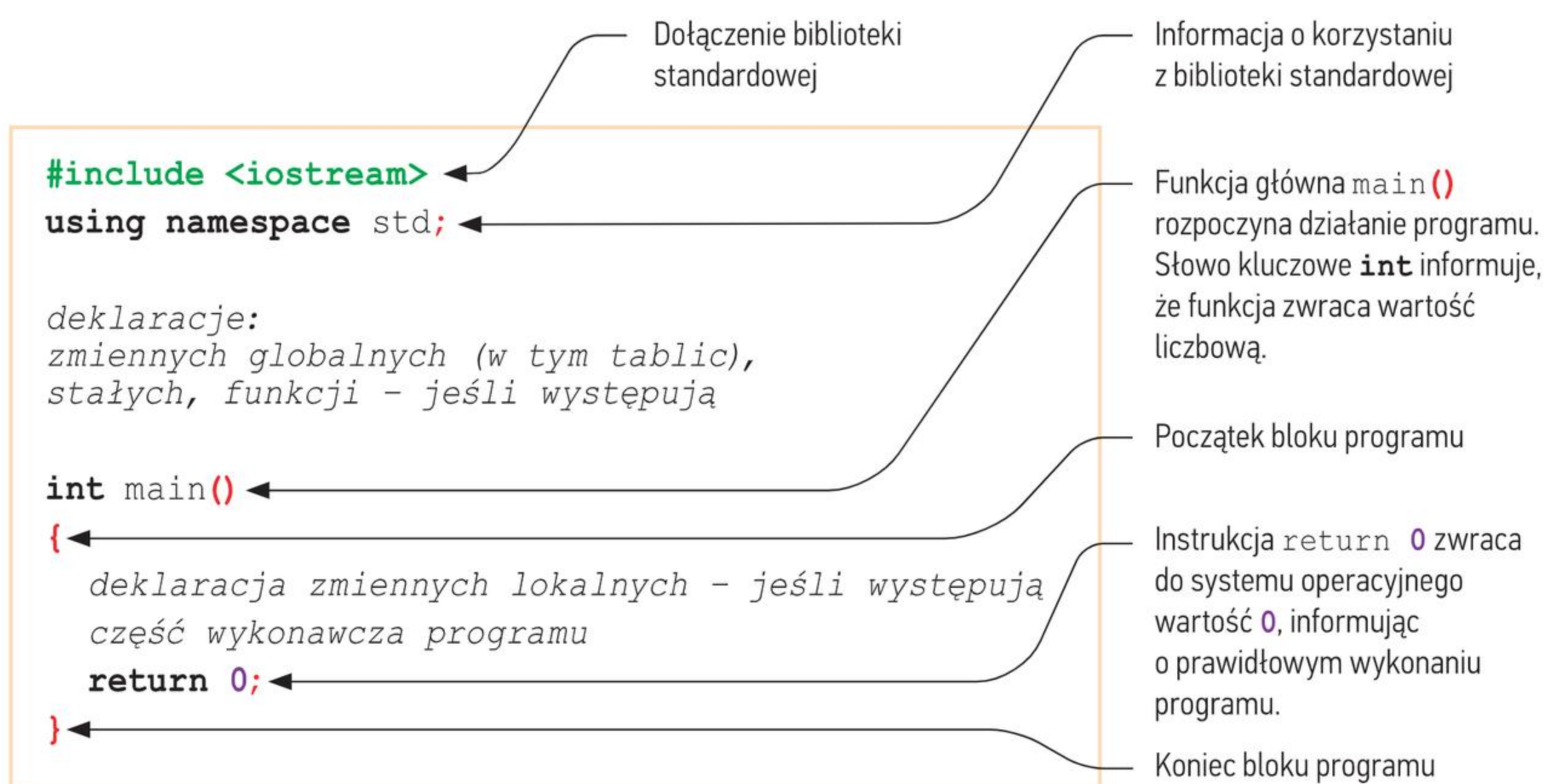
Rys. 6. Ogólna struktura programu w języku C++
