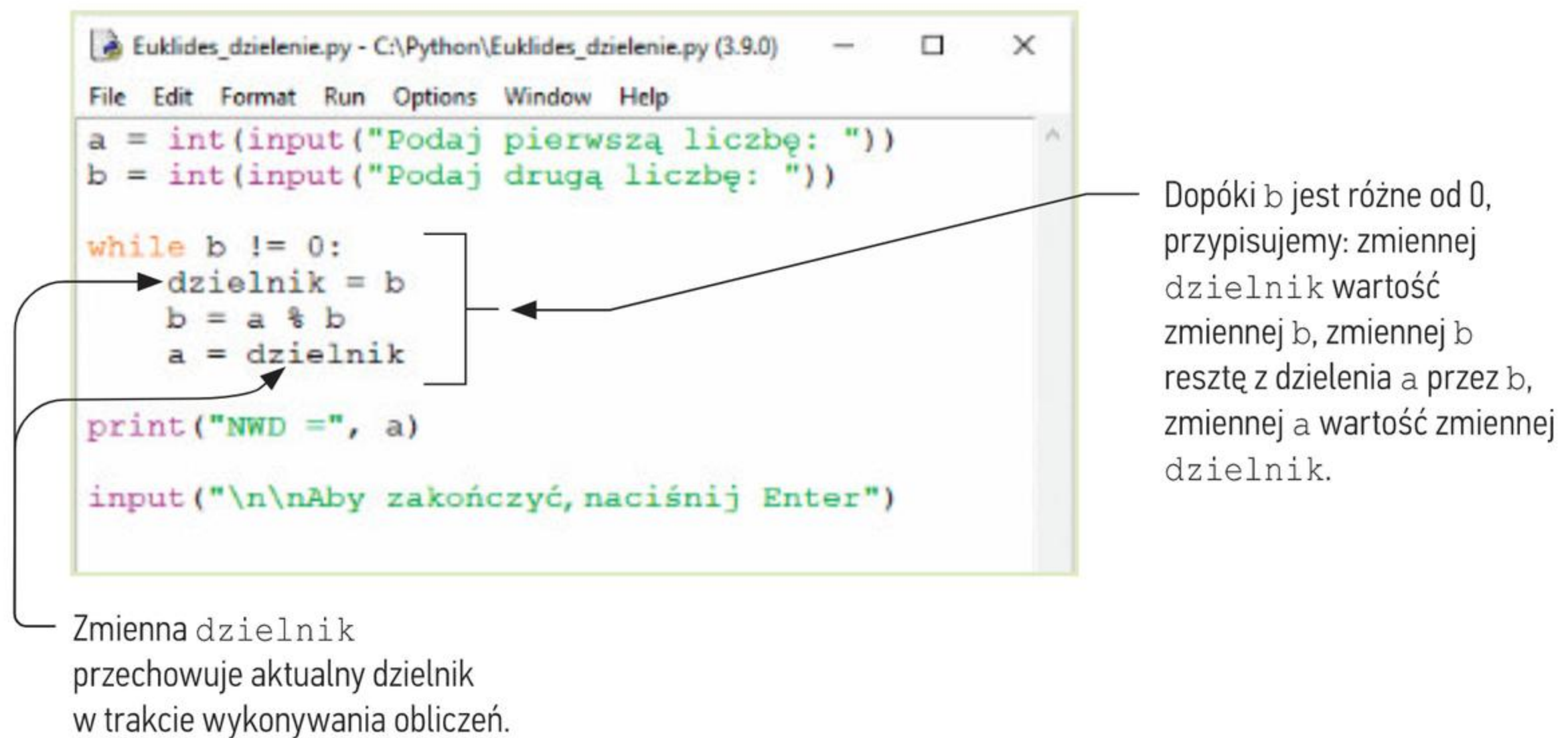
Rys. 8. Program w języku Python realizujący algorytm Euklidesa w wersji z resztą z dzielenia
