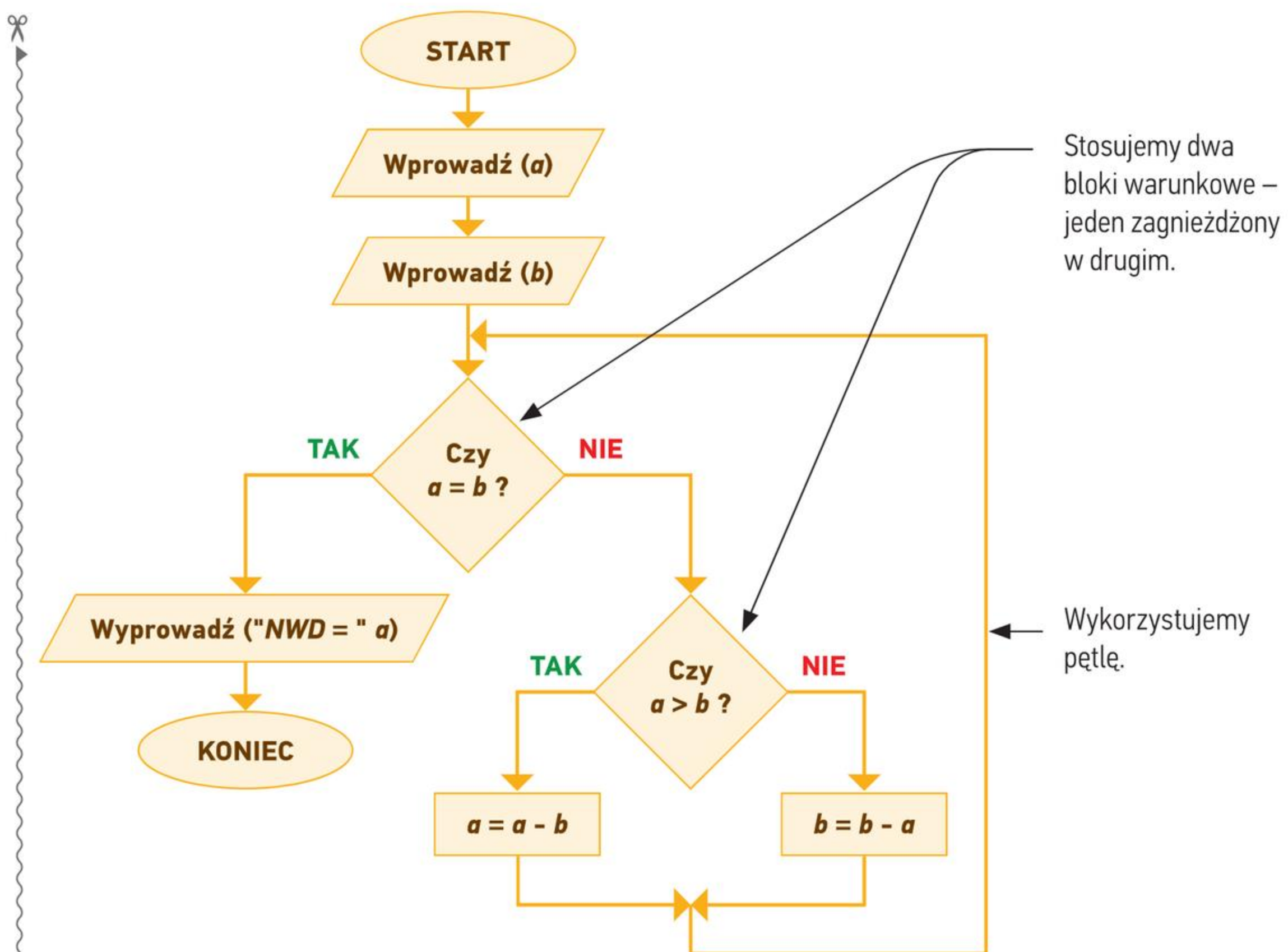
Rys. 5. Schemat blokowy algorytmu Euklidesa w wersji z odejmowaniem
