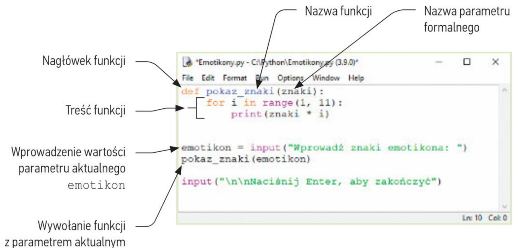
Rys. 11. Program w języku Python, w którym zdefiniowano funkcję niezwracającą wartości z jednym parametrem – ćwiczenie 10.
