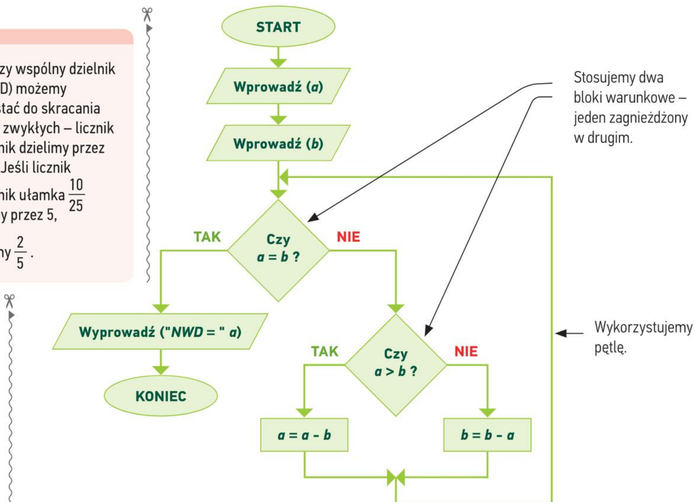
Rys. 5. Schemat blokowy algorytmu Euklidesa w wersji z odejmowaniem
