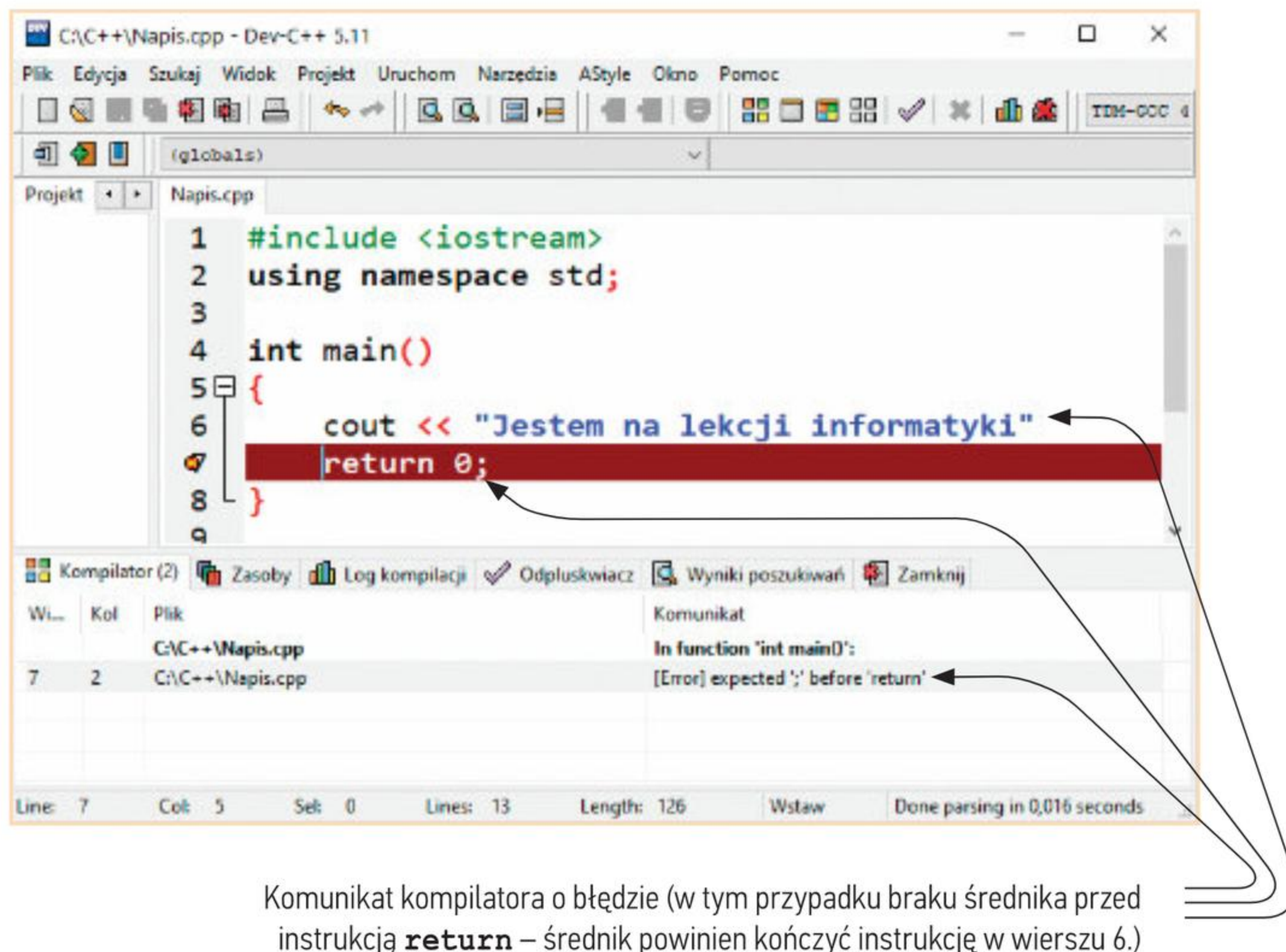
Rys. 9. Okno programu Dev-C++ – kompilator wykrył błąd w programie napisanym w języku C++
