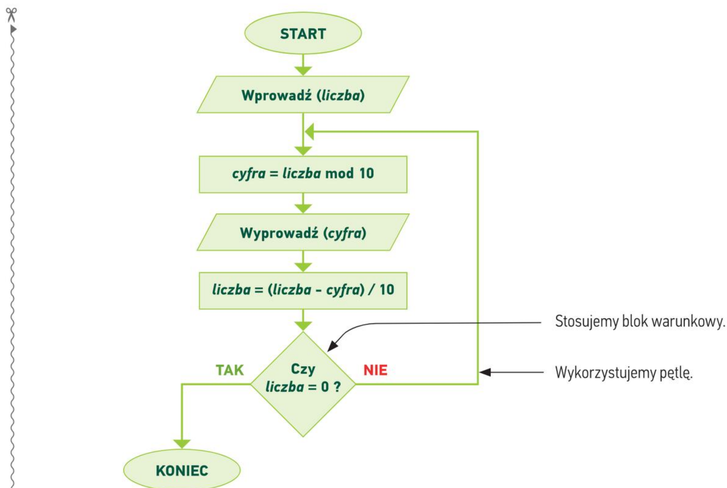
Rys. 9. Schemat blokowy algorytmu wyodrębniania cyfr danej liczby od cyfry jedności
