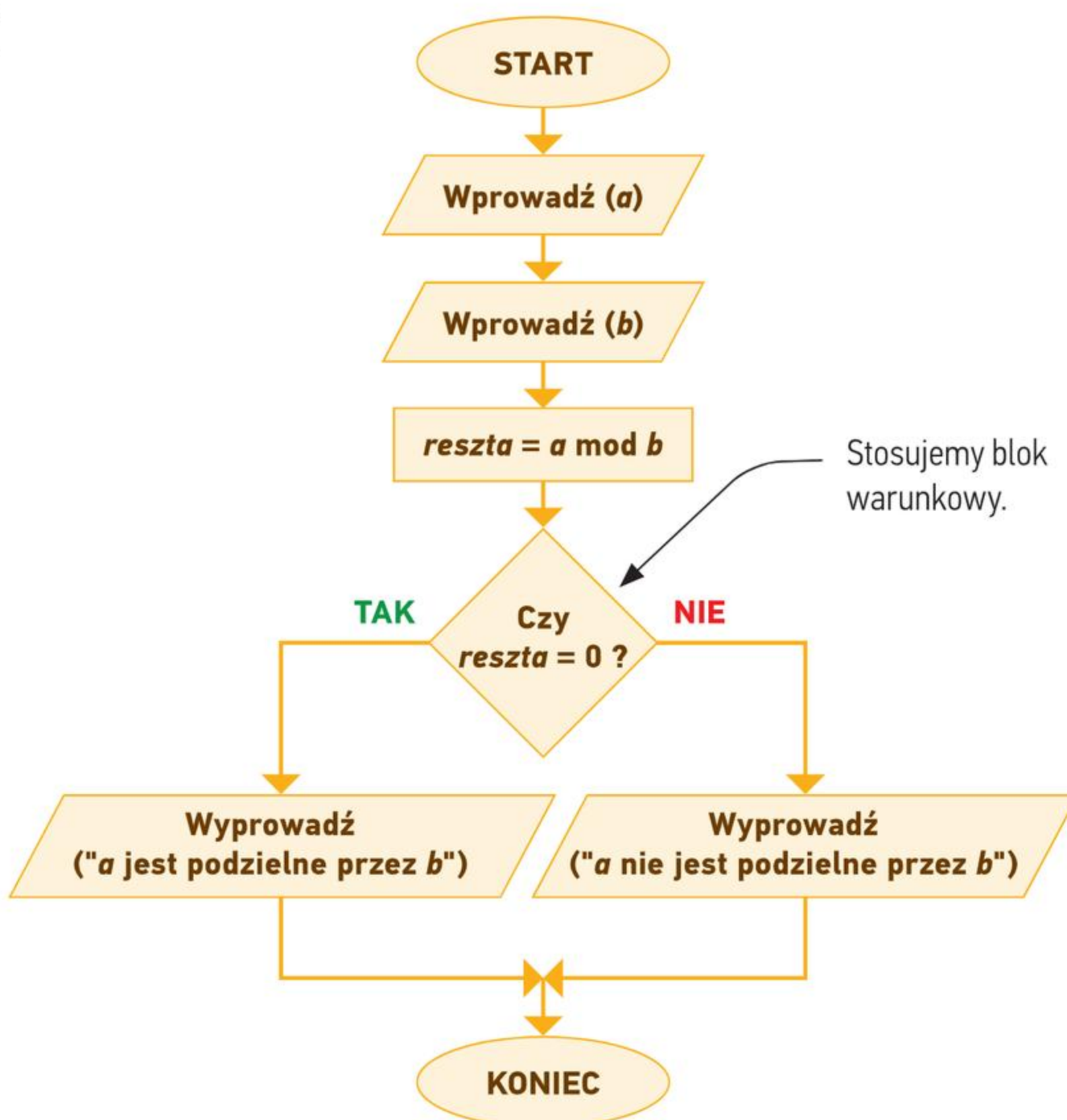
Rys. 2. Schemat blokowy algorytmu badania podzielności liczb
