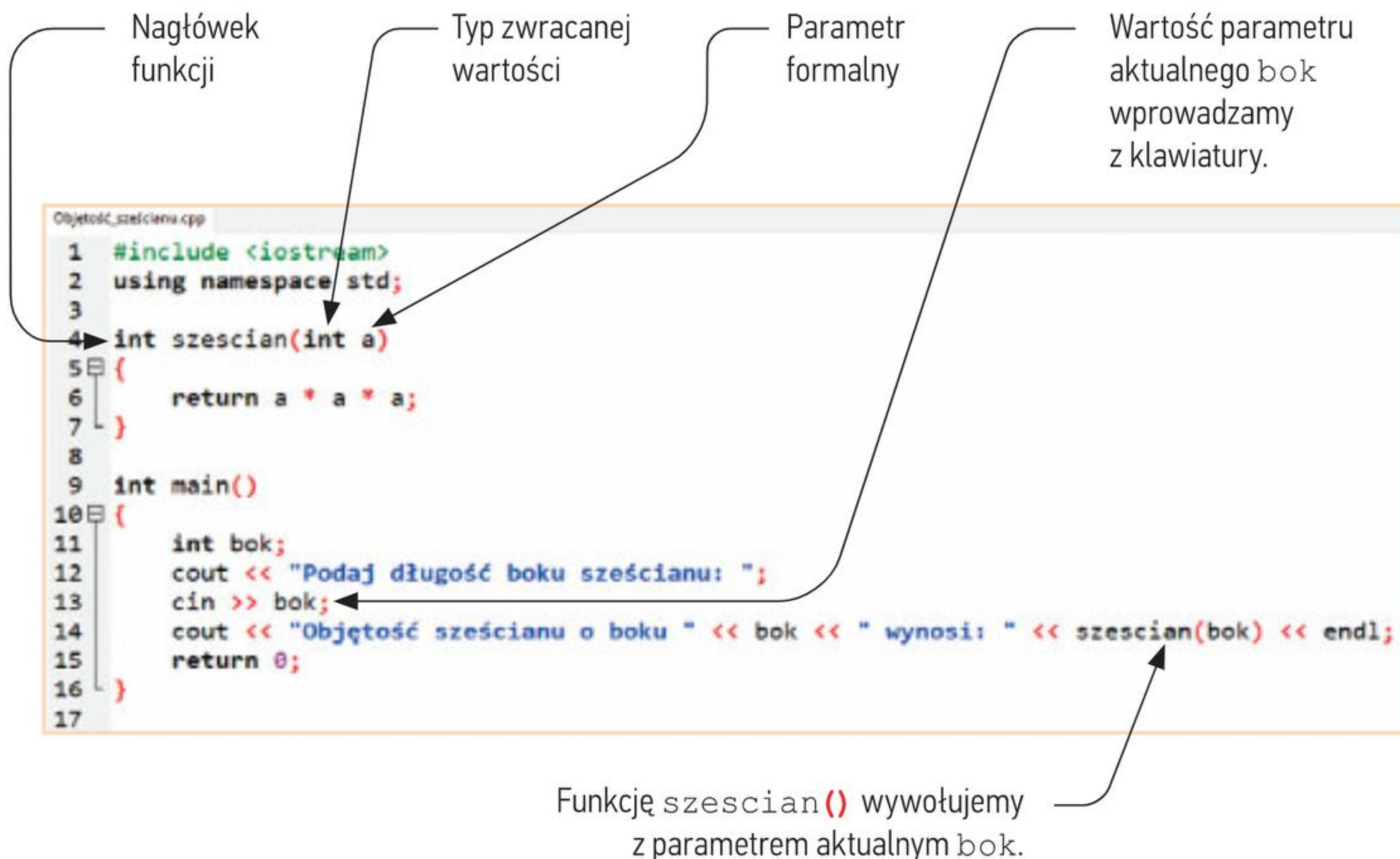
Rys. 12. Definiowanie i wywołanie funkcji zwracającej wartość z jednym parametrem w języku C++ – ćwiczenie 9.
