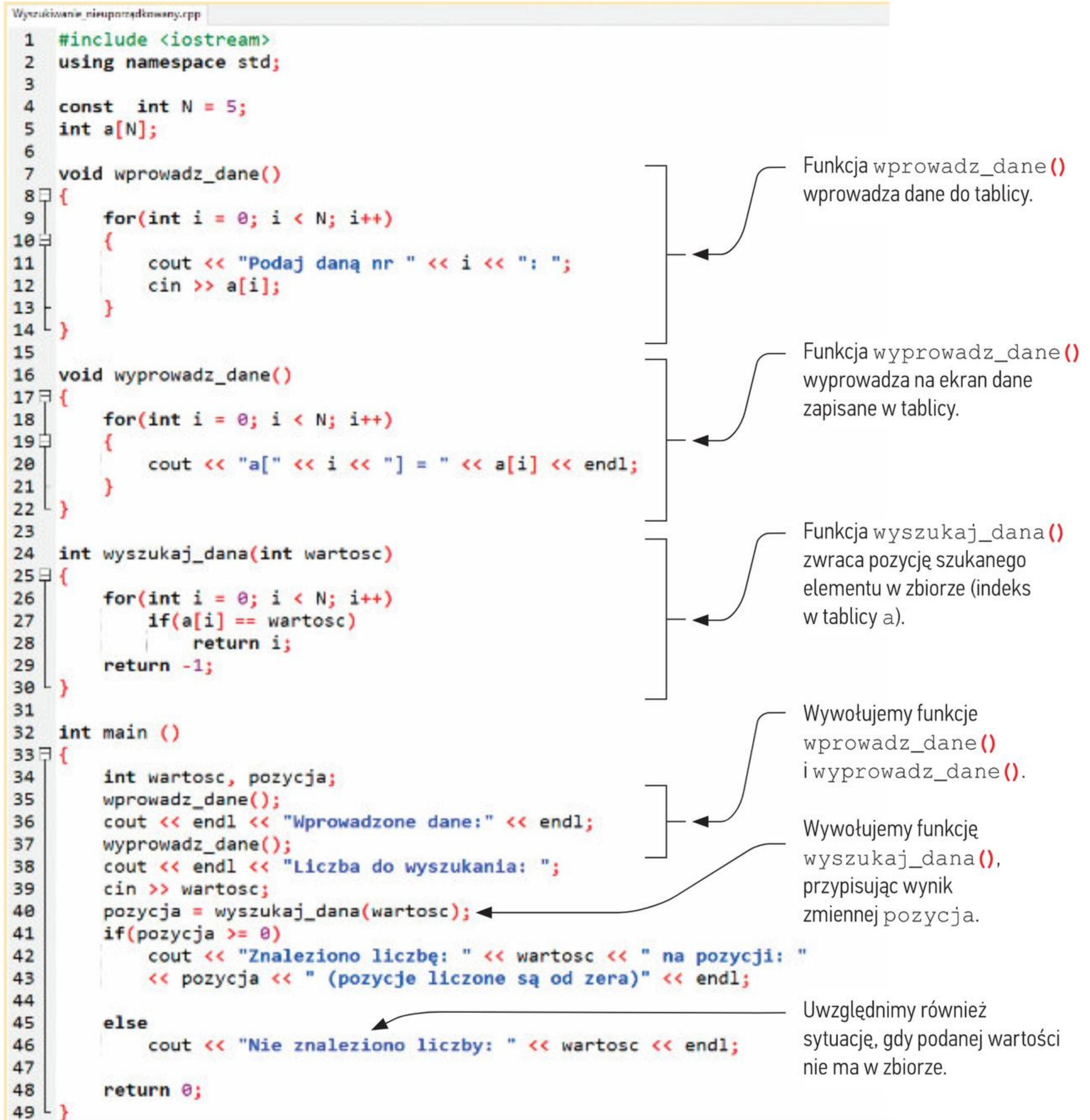
Rys. 4. Program realizujący algorytm wyszukiwania elementu w zbiorze nieuporządkowanym w języku C++ – ćwiczenie 5.
