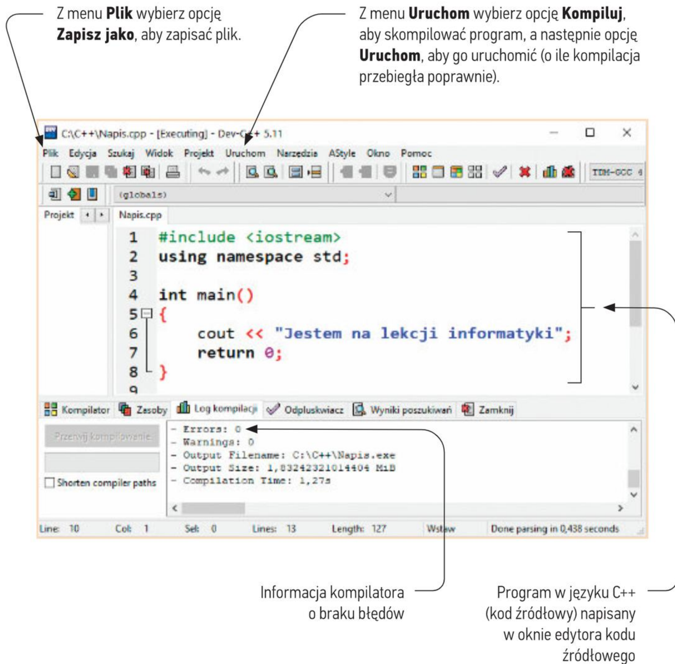
Rys. 7. Okno programu Dev-C++ – kompilacja programu napisanego w języku C++ przebiegła prawidłowo
