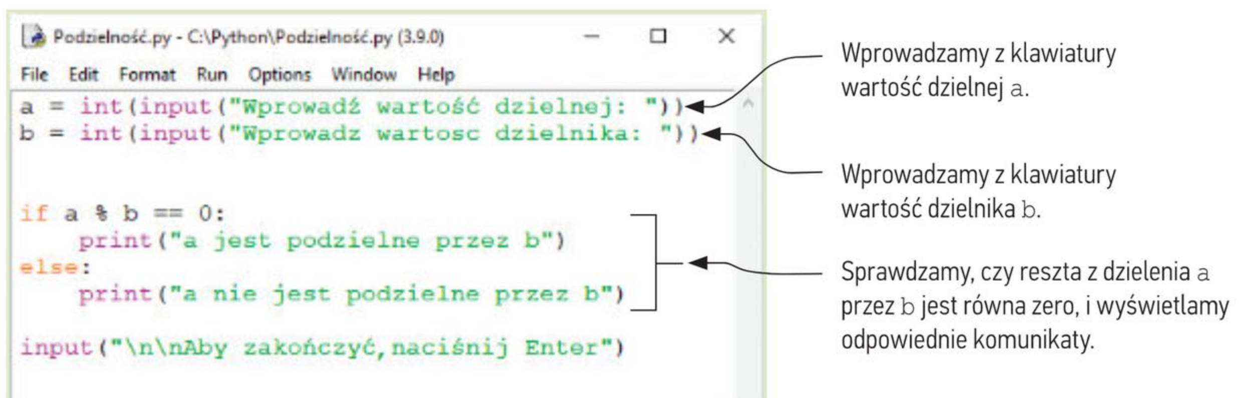
Rys. 3. Program w języku Python realizujący algorytm badania podzielności liczb naturalnych
