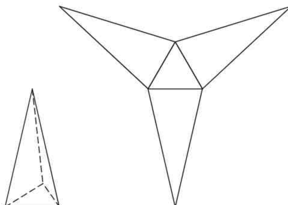
ostrosłup o podstawie w kształcie trójkąta równobocznego
