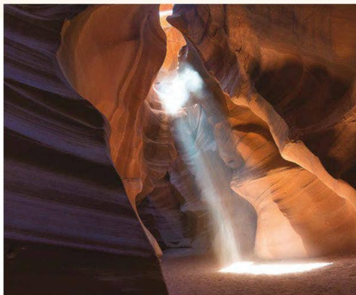
Promień światła wpadający do podziemnego kanału – fotografia wykonana w Kanionie Antylopy w Arizonie (USA)
