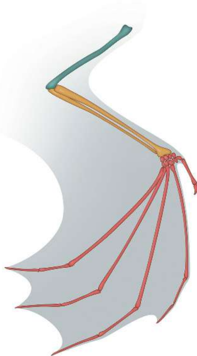
nietoperz
