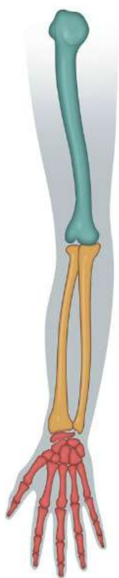
człowiek
