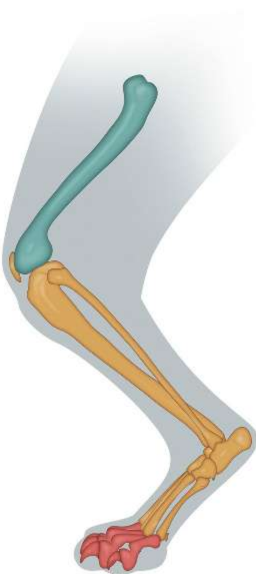
kot
