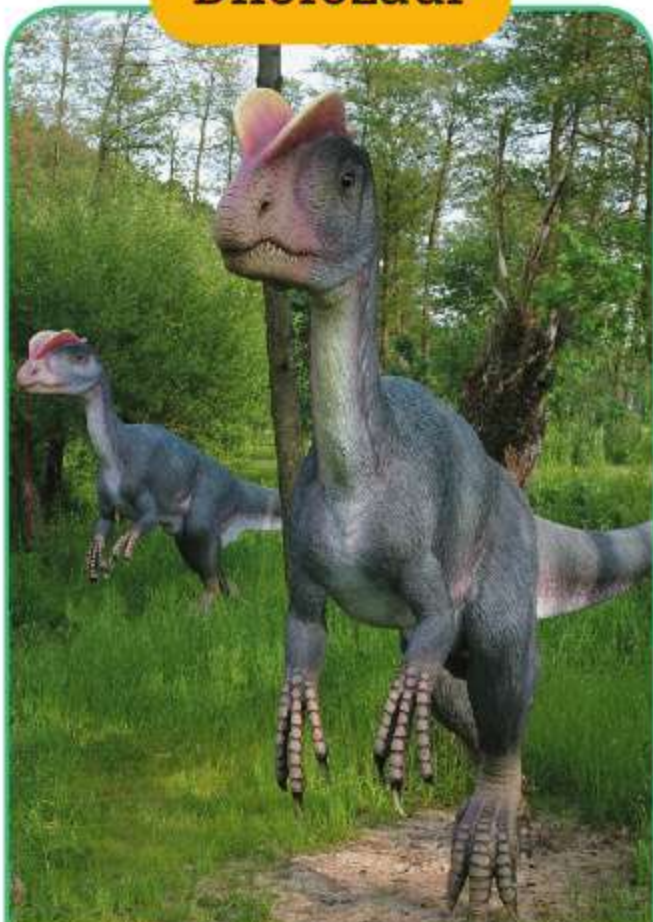
Dilofozaur
