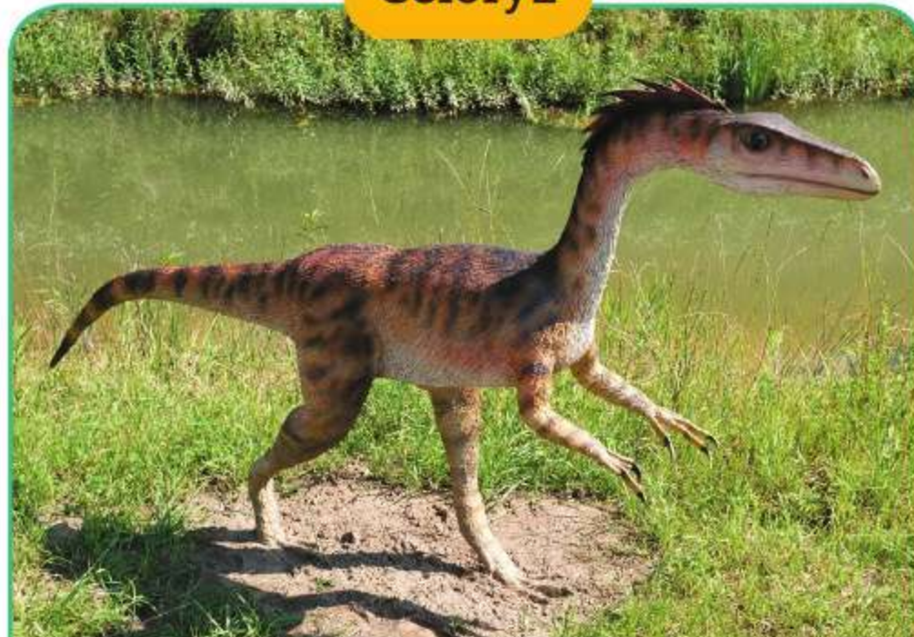
Celofyz
