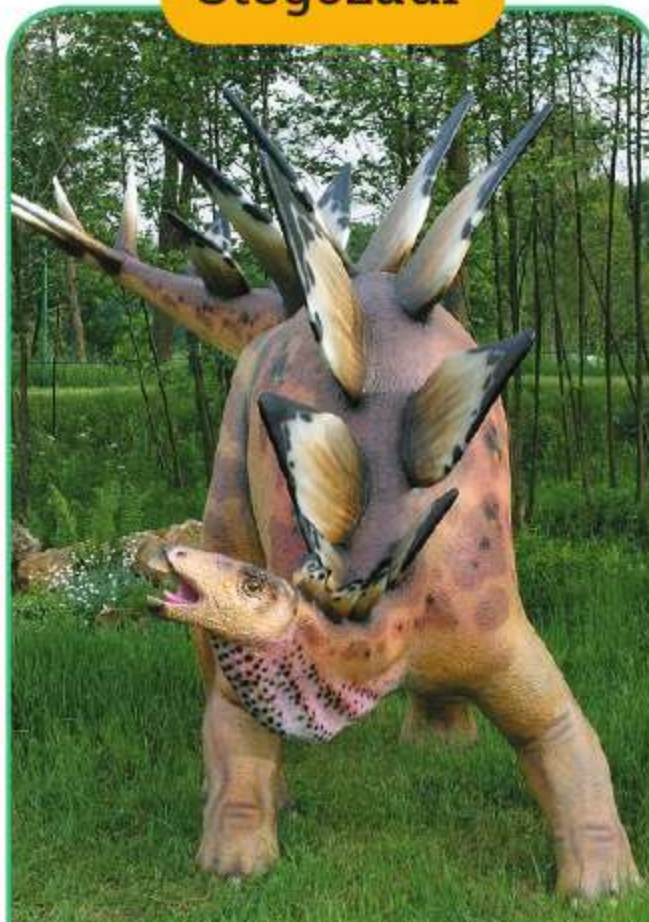
Stegozaur
