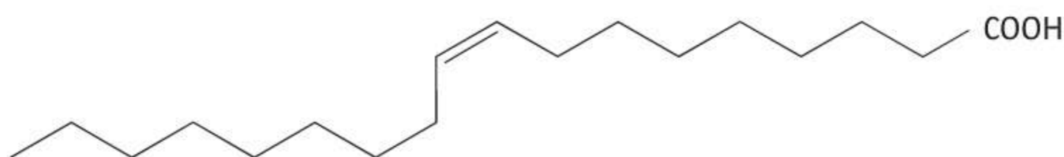
kwas oleinowy
