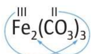
węglan żelaza(III)
