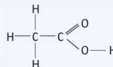
wzór strukturalny
