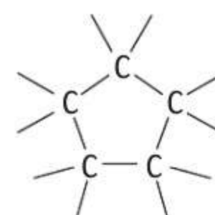
forma pierścieniowa
