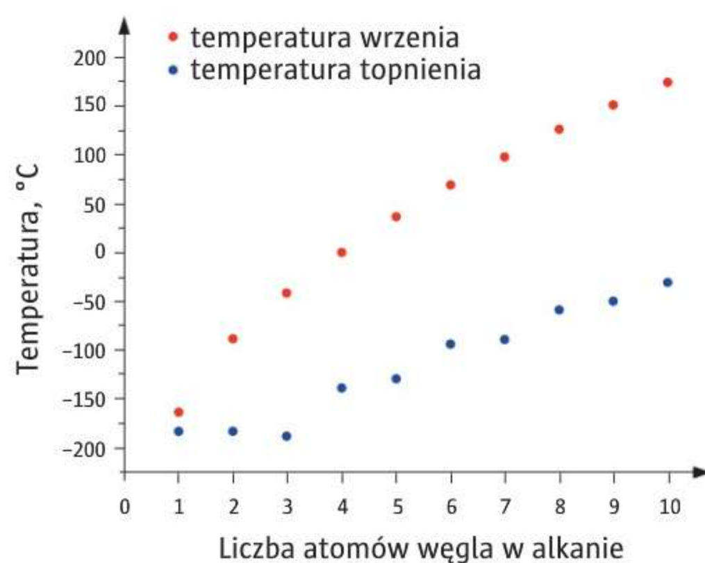
◀ Wykresy przedstawiające zmiany temperatury wrzenia i temperatury topnienia w szeregu homologicznym alkanów
