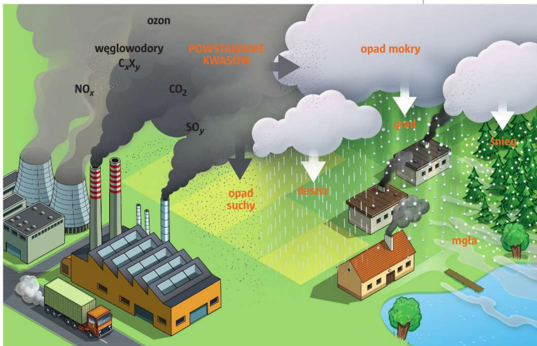
▲ Powstawanie kwaśnych opadów
