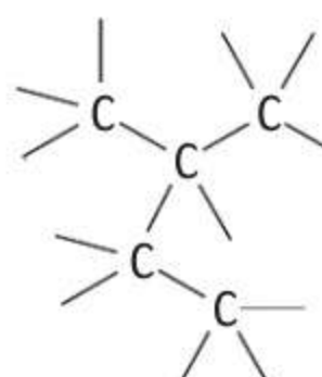
łańcuch rozgałęziony
