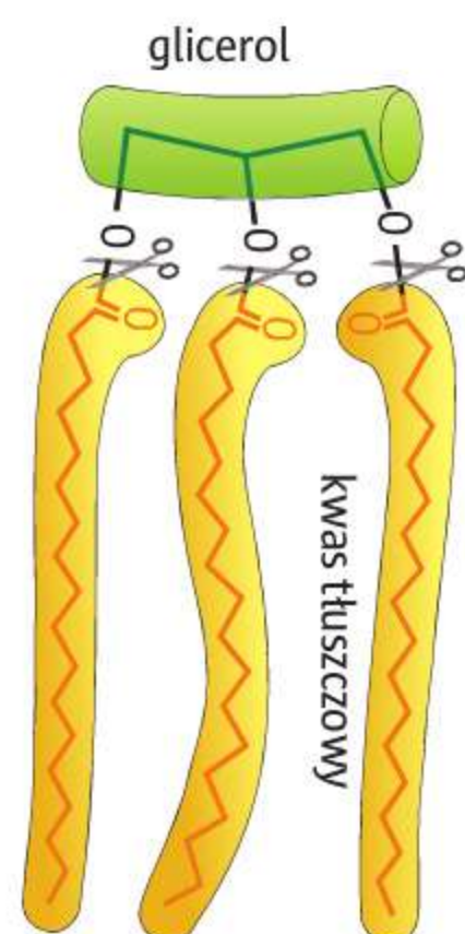
▲ Hydroliza tłuszczu
