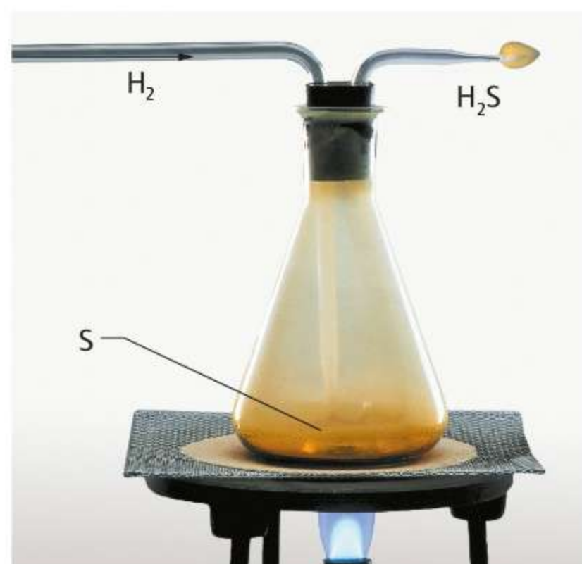
▲ Otrzymywanie siarkowodoru – reakcja spalania wodoru w parach siarki
