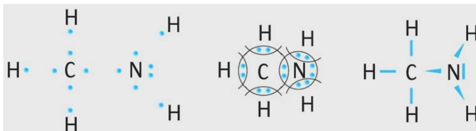
▲ Schemat tworzenia wiązań chemicznych w cząsteczce metyloaminy
