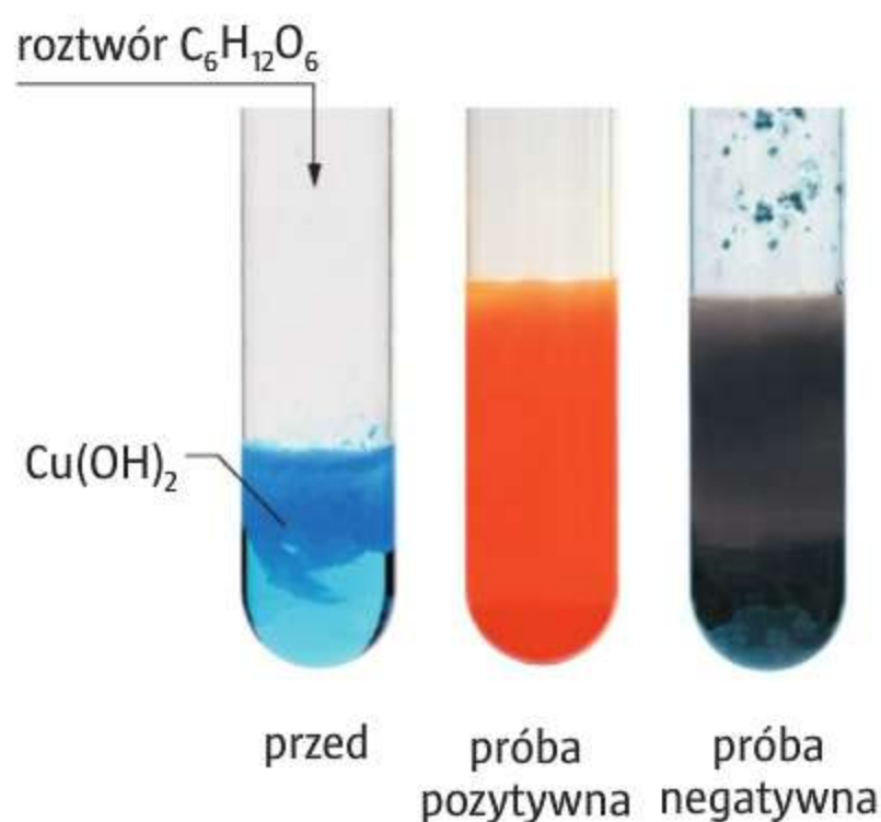
▲ Reakcja charakterystyczna glukozy
