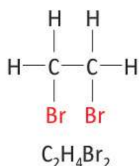
1,2-dibromoetan
