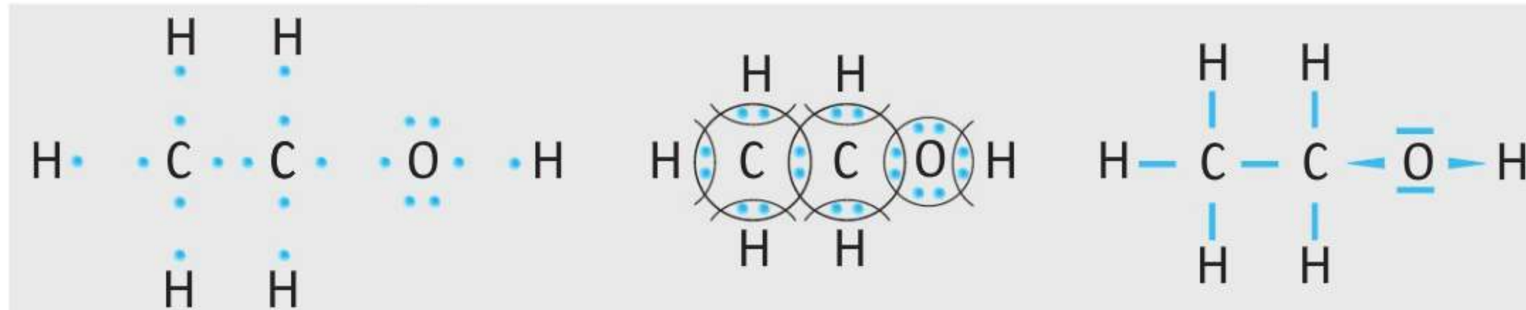
▲ Schemat tworzenia wiązań chemicznych w cząsteczce etanolu
