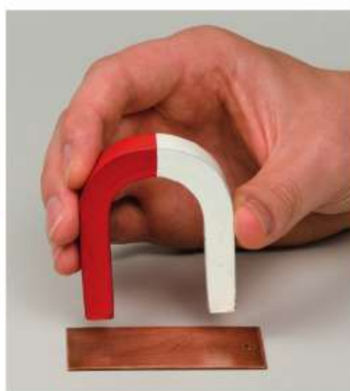
Miedź nie oddziałuje z magnesem.
