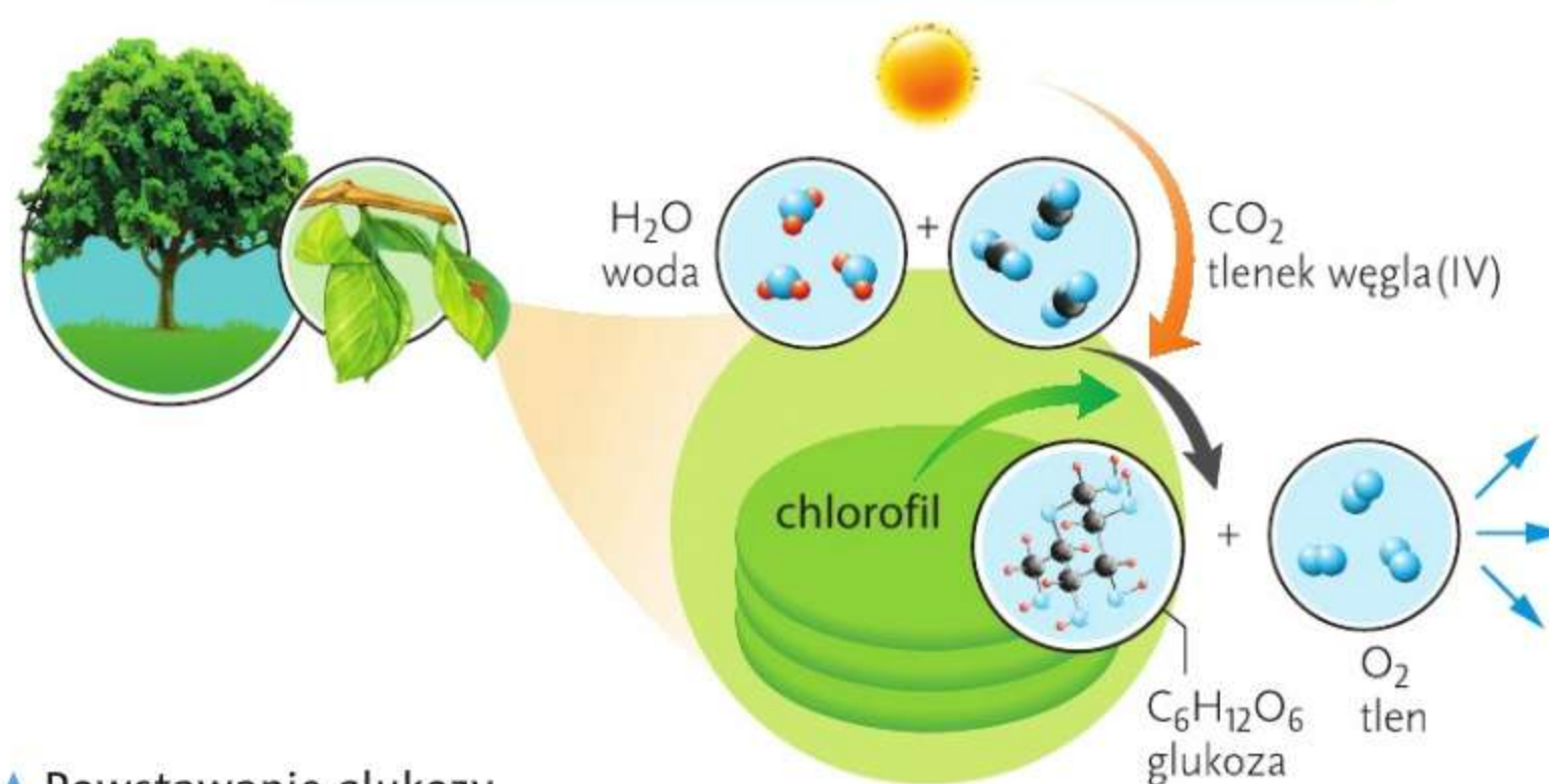
▲ Powstawanie glukozy
