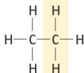
etan C_2H_6
