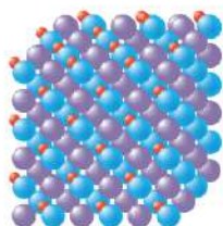
▲ Sieć krystaliczna NaOH
