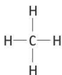
metan CH_4
