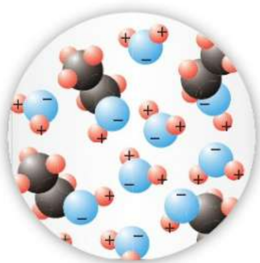
▲ Oddziaływania cząsteczek etanolu z cząsteczkami wody
