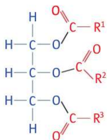
wzór ogólny strukturalny tłuszczów
