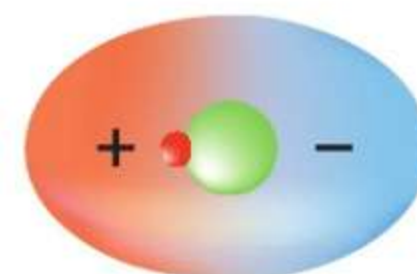
▲ Dipol chlorowodoru
