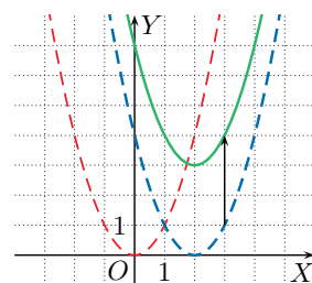
Wykres funkcji y = (x - 2)^2 + 3
