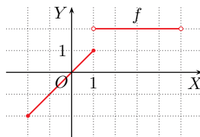
Wykres funkcji f
