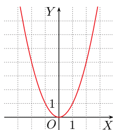
Wykres funkcji y = x^2
