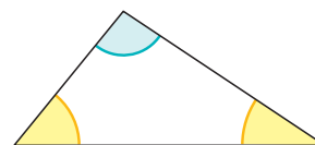
trójkąt rozwartokątny jeden kąt rozwarty
