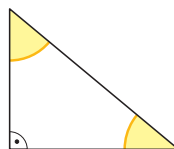
trójkąt prostokątny jeden kąt prosty
