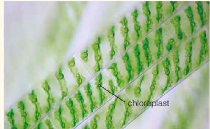
Plechy skrzętnicy.
