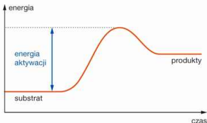
Przebieg reakcji endoergicznej.
