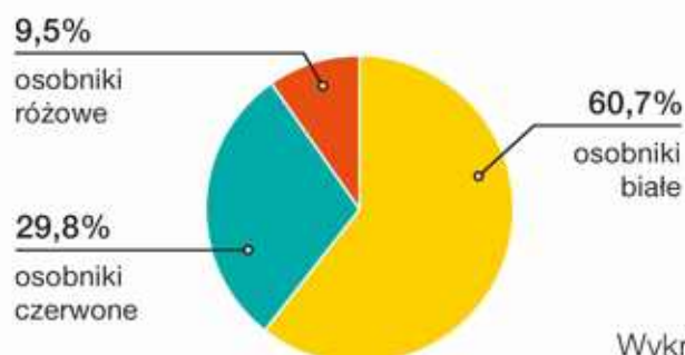
Wykres kołowy.
