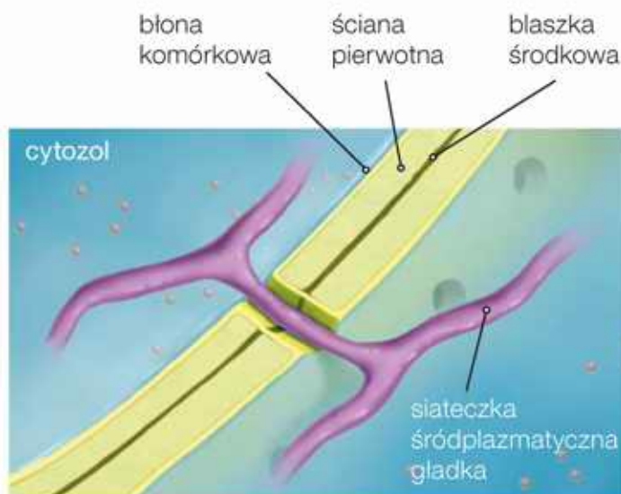
Budowa plazmodesmy.
