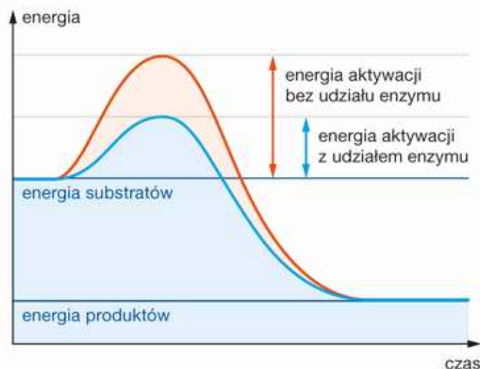
Przebieg reakcji z użyciem katalizatora (enzymu) i bez użycia katalizatora.
