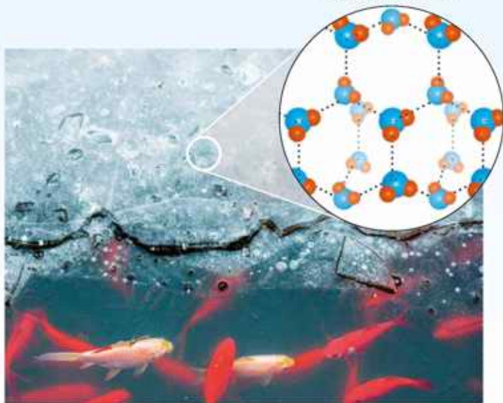
Struktura lodu
