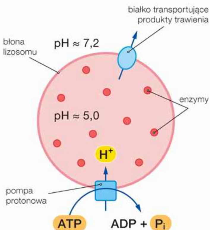
Budowa lizosomu.
