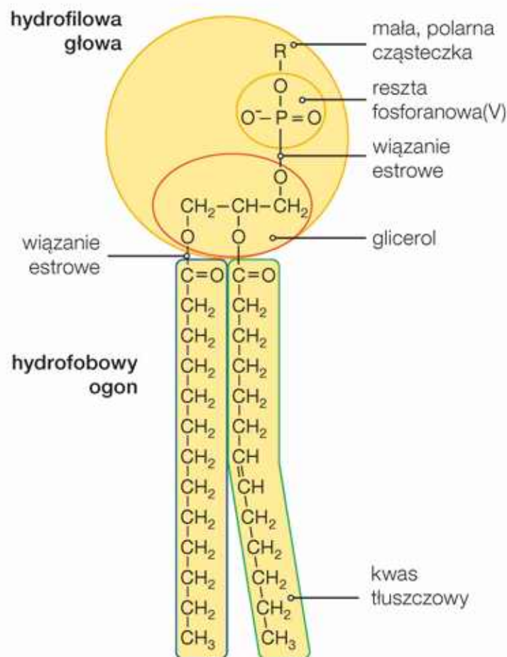
Budowa fosfolipidu.
