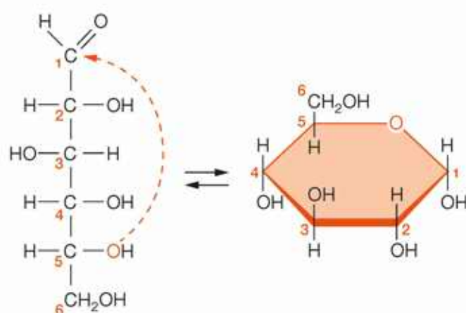
postać łańcuchowa
