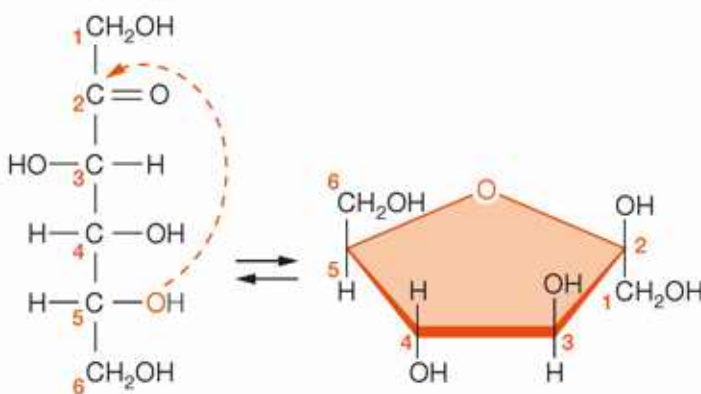
postać łańcuchowa
