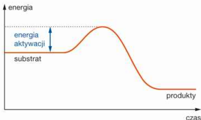
Przebieg reakcji egzoergicznej.
