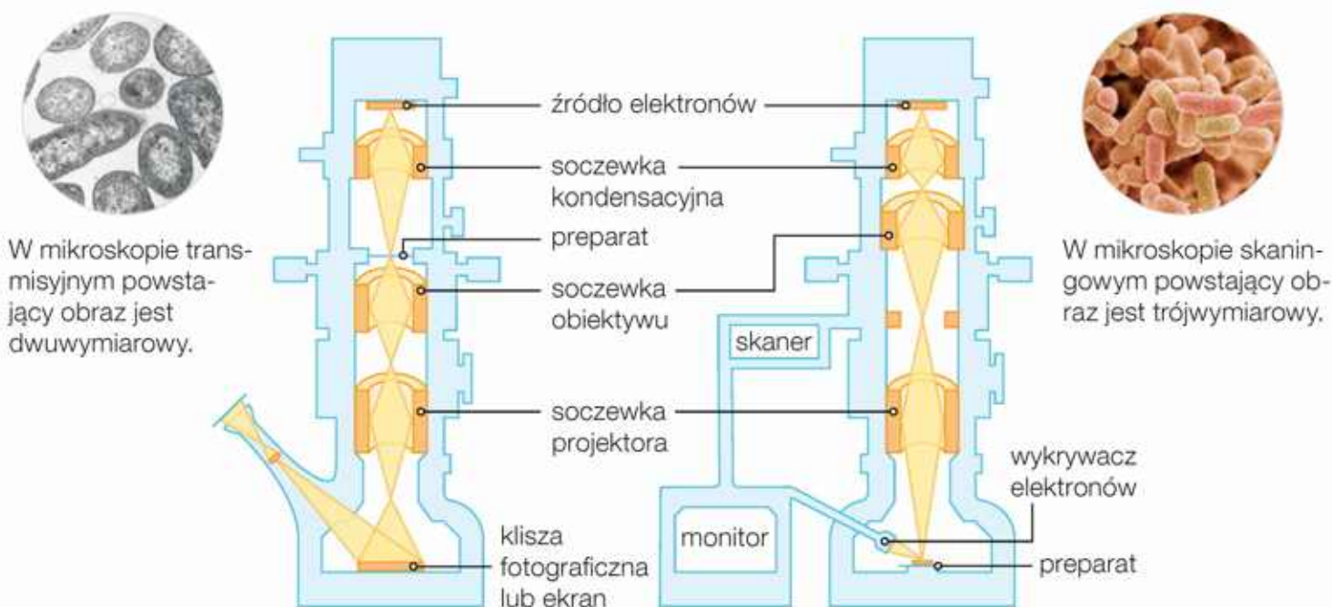
Budowa mikroskopów elektronowych.
