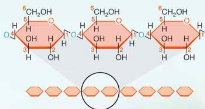
ściana komórkowa
