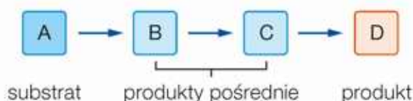
Szlak metaboliczny.
