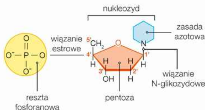
Budowa nukleotydu.
