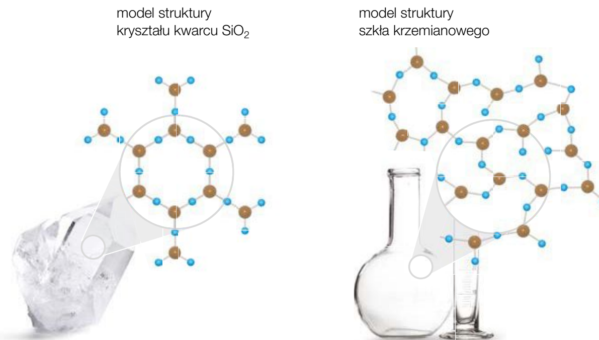
Fot. 35. Tlenek krzemu(IV) jest głównym składnikiem kwarcu i szkła krzemianowego.
