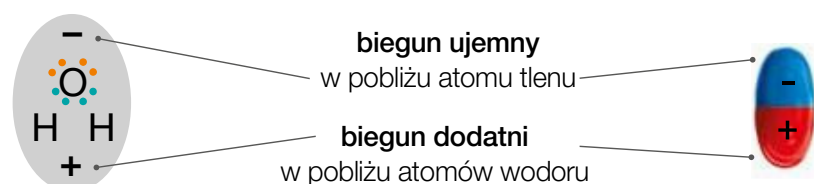
Rys. 8. Cząsteczka wody jest dipolem – ma budowę polarną.
