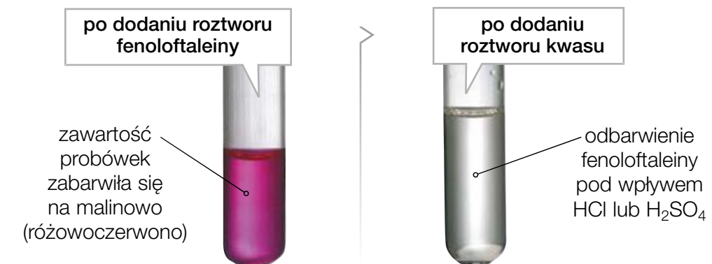
Fot. 82. Otrzymywanie soli.
