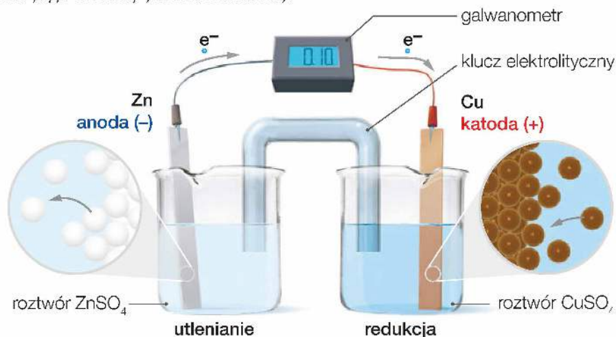
Rys. 48. Ogniw Daniella.
