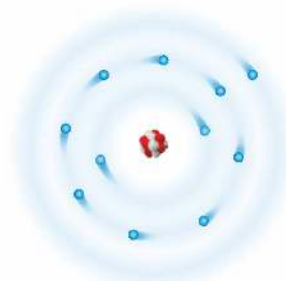
Rys. 14. Poruszające się wokół jądra atomowego elektrony tworzą powłoki elektronowe.
