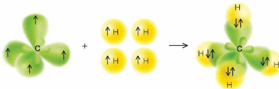
Rys. 39. Model tworzenia się cząsteczki metanu.
