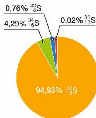
skład procentowy izotopów siarki
