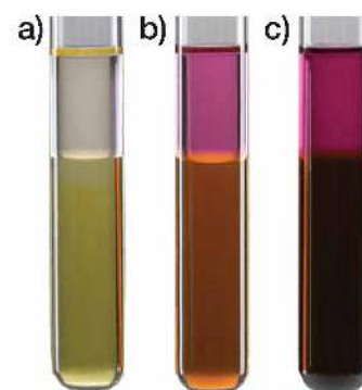
Fot. 167. Badanie aktywności chemicznej fluorowców: a) chloru i bromu, b) chloru i jodu, c) bromu i jodu.
