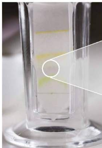
Fot. 81. Rozdzielanie barwników roślinnych metodą chromatografii bibułowej.
