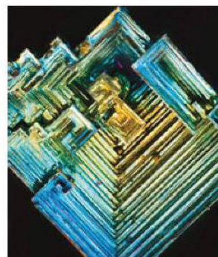
Fot. 151. Bizmut.
