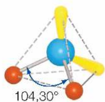
Rys. 43. Przestrzenna budowa cząsteczki wody.
