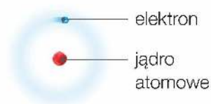
Rys. 17. Model atomu wodoru – dodatni ładunek jądra atomowego i ujemny ładunek elektronów równoważą się.
