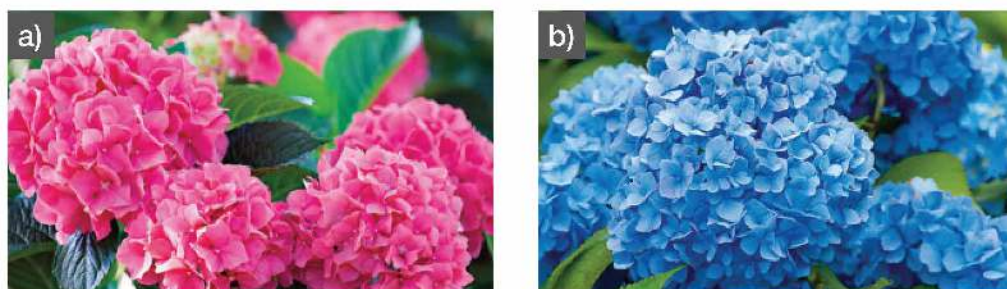
Fot. 127. Płatki kwiatów hortensji mają różną barwę w zależności od odczynu gleby, na której rosną. Barwa hortensji na glebie o odczynie: a) zasadowym, b) kwasowym.
