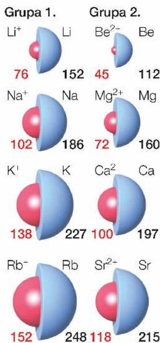
Rys. 28. Porównanie wielkości kationów i atomów (wartości promieni w pm); modele przedstawiają wzajemne proporcje jonów i atomów.
