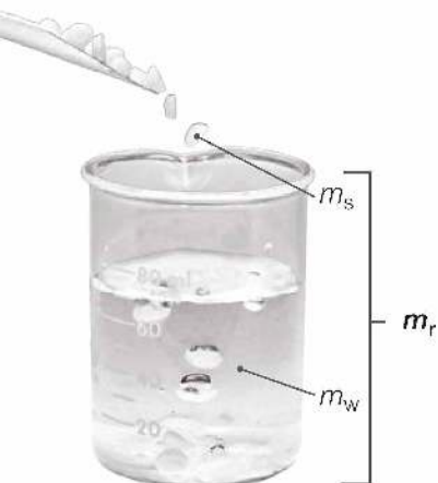
Fot. 94. Roztwór wodorotlenku sodu.
