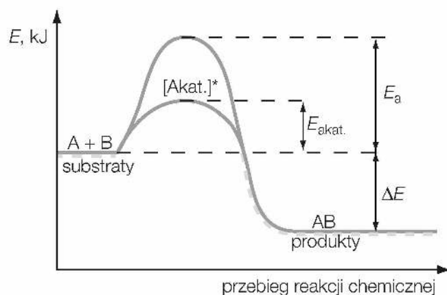
Rys. 57. Wykres zmian energii w reakcji egzotermicznej, gdzie:
