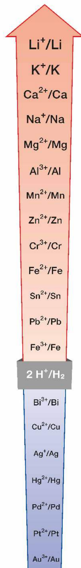
Rys. 46. Szereg aktywności metali.
