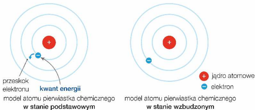
Rys. 8. Model atomu wodoru. W wyniku pochłonięcia kwantu energii atom osiąga stan wzbudzony.
