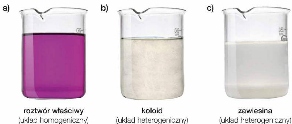
Fot. 80. Manganian(VII) potasu z wodą – a), białko z wodą – b), mąka z wodą – c).
