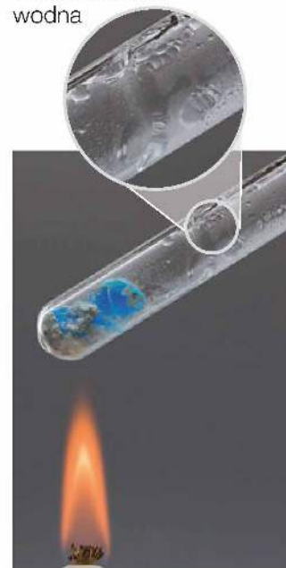
Fot. 49. Ogrzewanie siarczanu(VI) miedzi(II)–woda(1/5).
