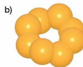
Rys. 63. Cząsteczka siarki \text{S}_8 : a) wzór strukturalny, b) model czaszowy.
