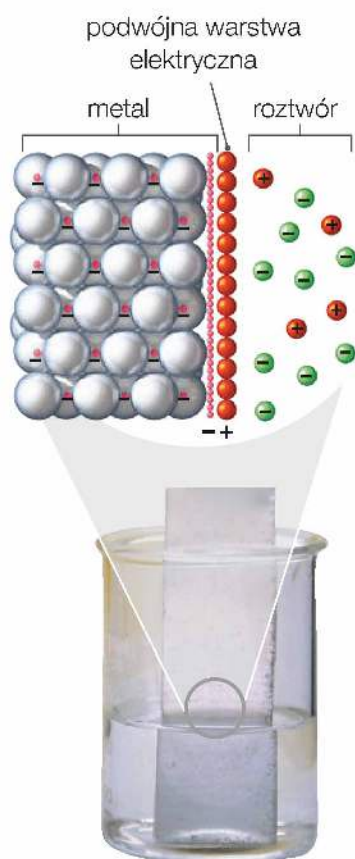
Fot. 74. Na granicy faz od strony metalu występuje nadmiar elektronów, a od strony roztworu – nadmiar kationów.
