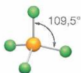
Rys. 37. Wiązania chemiczne w cząsteczce metanu.
