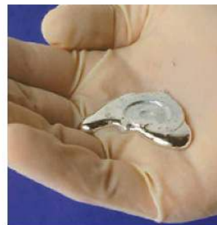
Fot. 145. Temperatura topnienia galu wynosi 29,8^{\circ}C , dlatego ten metal topi się w dłoni.
