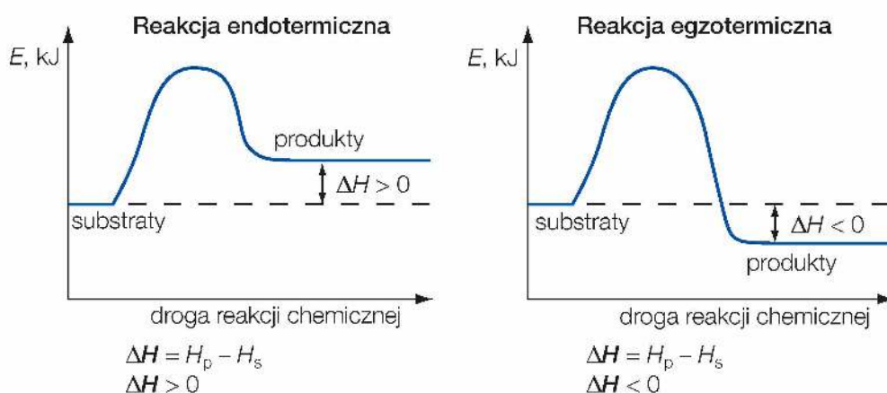
Rys. 54. Wykres zmian energii substratów i produktów.
