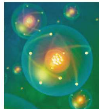
Rys. 27. Model cząsteczki wody – atomy wodoru i tlenu łączą się za pomocą wiązań chemicznych.
