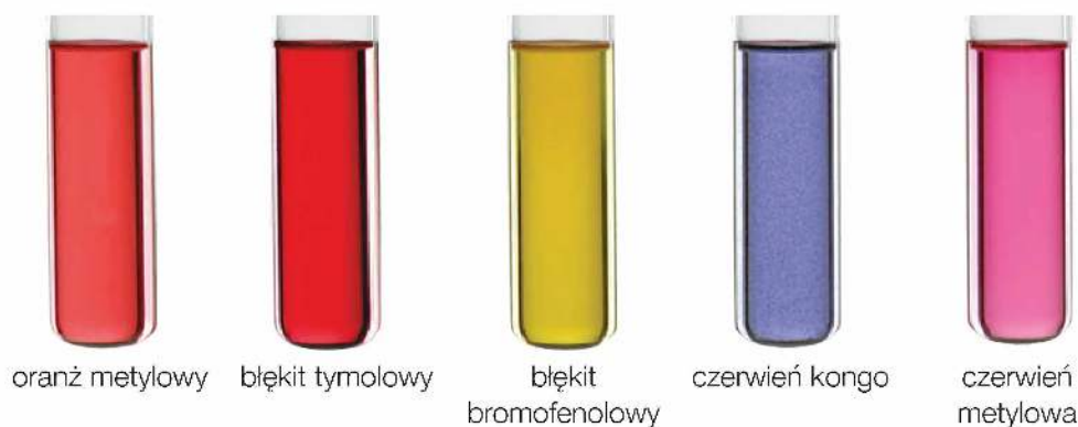
Fot. 45. Barwy wskaźników w roztworze zawierającym jony oksoniowe \text{H}_3\text{O}^+ .
