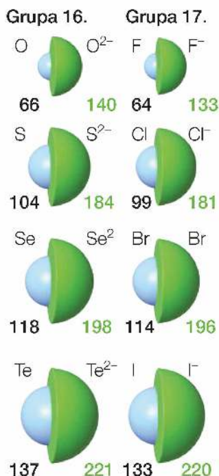
Rys. 29. Porównanie wielkości atomów i anionów (wartości promieni w pm); modele przedstawiają wzajemne proporcje atomów i jonów.
