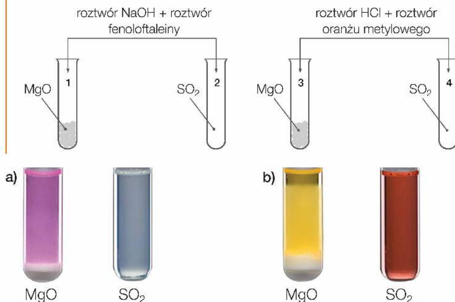
Fot. 28. Barwa fenoloftaleiny w probówkach zawierających NaOH oraz tlenki magnezu i siarki – a). Barwa oranżu metylowego w probówkach zawierających HCl oraz tlenki magnezu i siarki – b).
