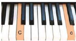
Fot. 11. Właściwości pierwiastków ułożonych wg zwiększających się mas atomowych powtarzają się co 8, jak dźwięki w oktawie muzycznej.
