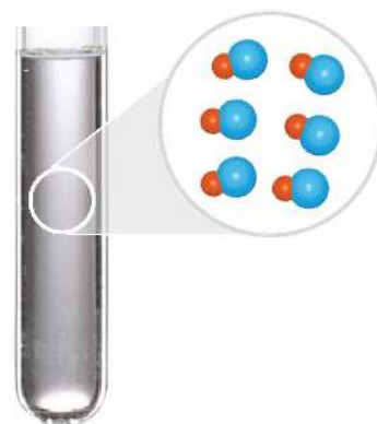
Fot. 122. W roztworach zasad znajdują się jony \text{OH}^- .
