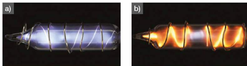
Fot. 170. Barwy światła emitowanego przez: a) argon, b) neon.
