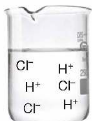
Fot. 123. W roztworach mocnych elektrolitów znajdują się tylko jony.
