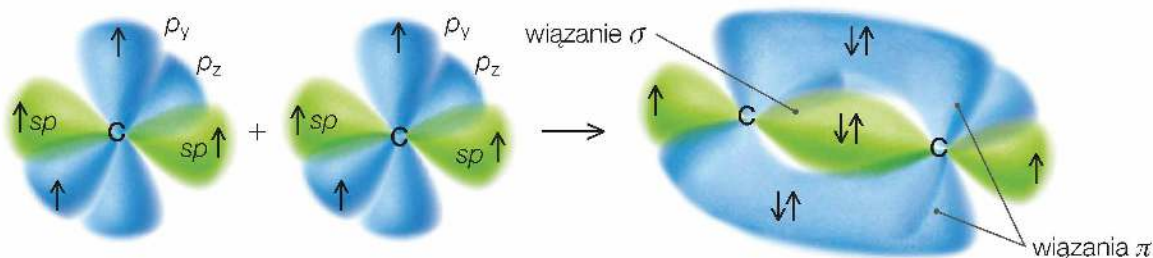
Rys. 41. Model tworzenia się wiązania C\equiv C .
