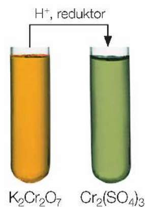
Fot. 175. Z pomarańczowego dichromianu(VI) potasu powstaje zielony roztwór siarczanu(VI) chromu(III).
