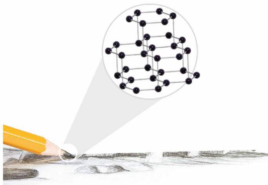
Rys. 33. Słabe siły van der Waalsa umożliwiają przesuwanie się warstw grafitu względem siebie, dlatego grafit ściera się, pozostawiając ślady.
