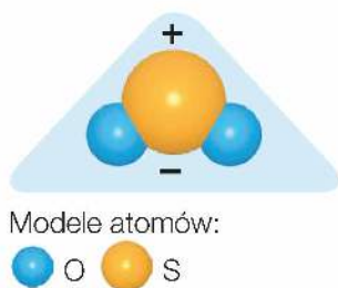
Rys. 42. Model cząsteczki polarnej \text{SO}_2 .
