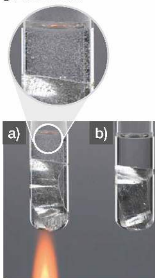
Fot. 108. Reakcja chemiczna glinu z kwasem chlorowodorowym: a) w wysokiej temperaturze, b) w temperaturze pokojowej.
