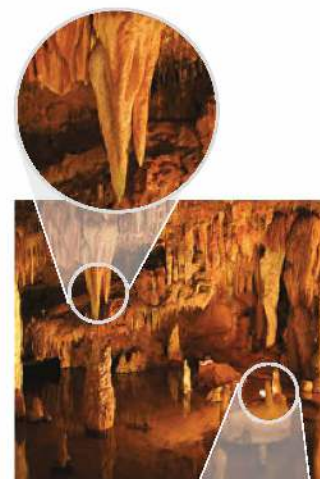
Fot. 55. Stalagmity i stalaktyty.
