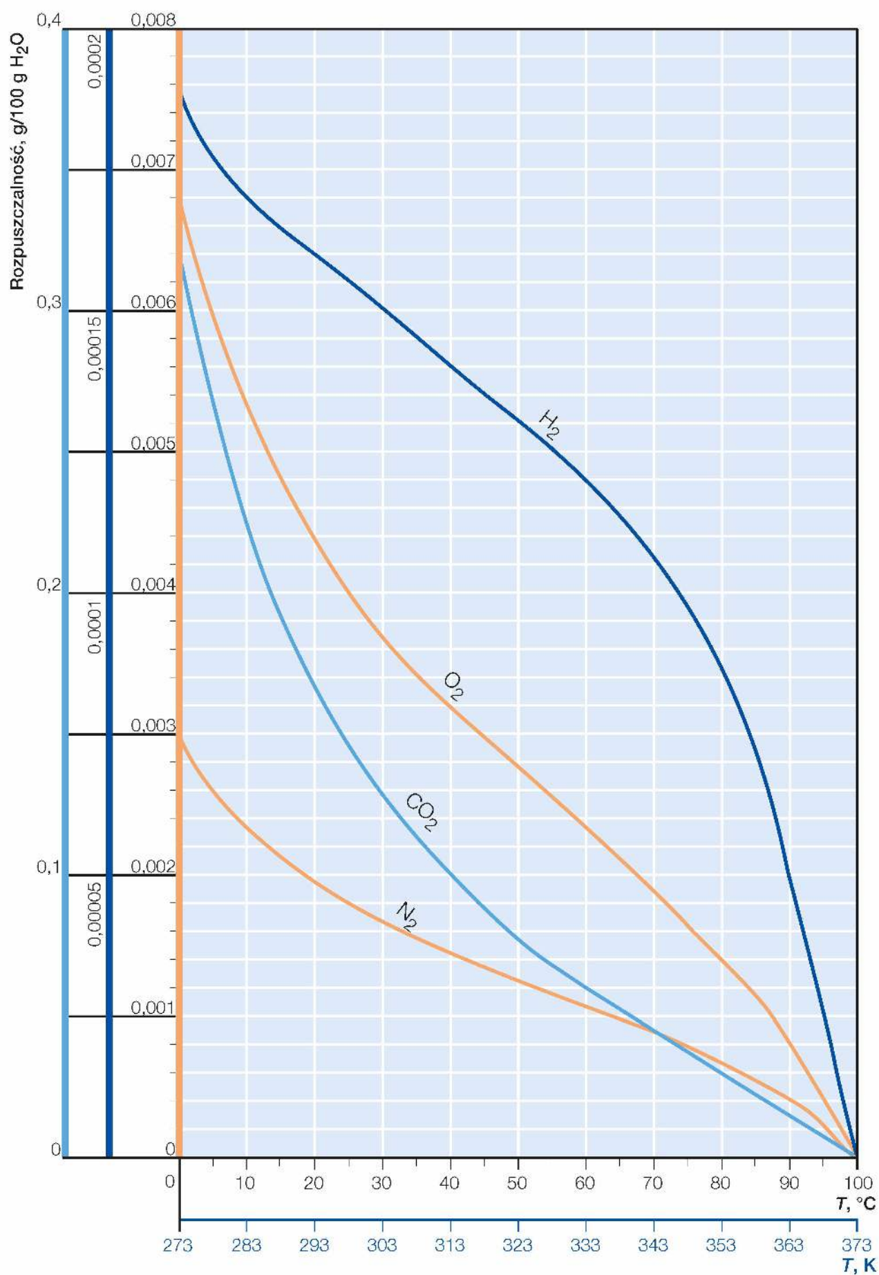
Rys. 53. Krzywe rozpuszczalności przedstawiają zależność rozpuszczalności gazów w wodzie od temperatury.
