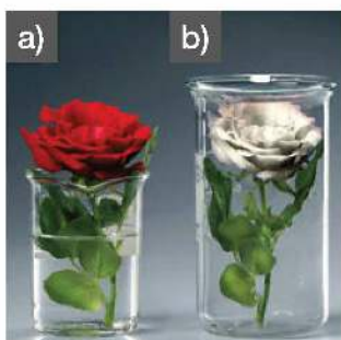
Fot. 162. Czerwona róża (a) w naczyniu z SO 2 po kilku minutach całkowicie traci swój kolor (b).
