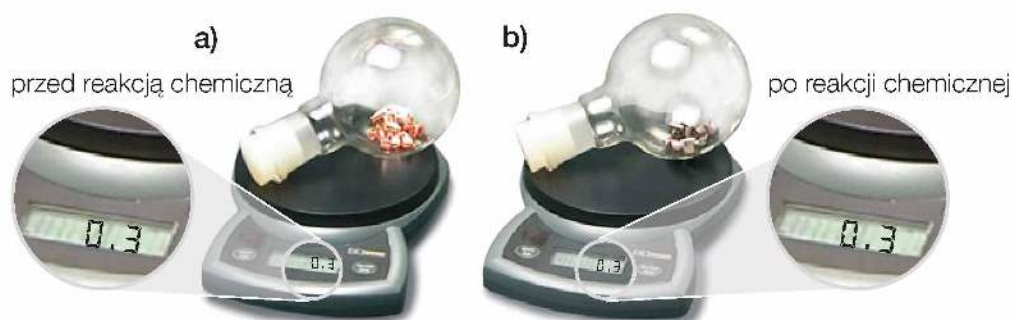
Fot. 23. Masa miedzi i tlenu (a) jest równa masie tlenku miedzi(II) (b).
