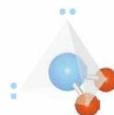
Rys. 36. Model cząsteczki wody.
