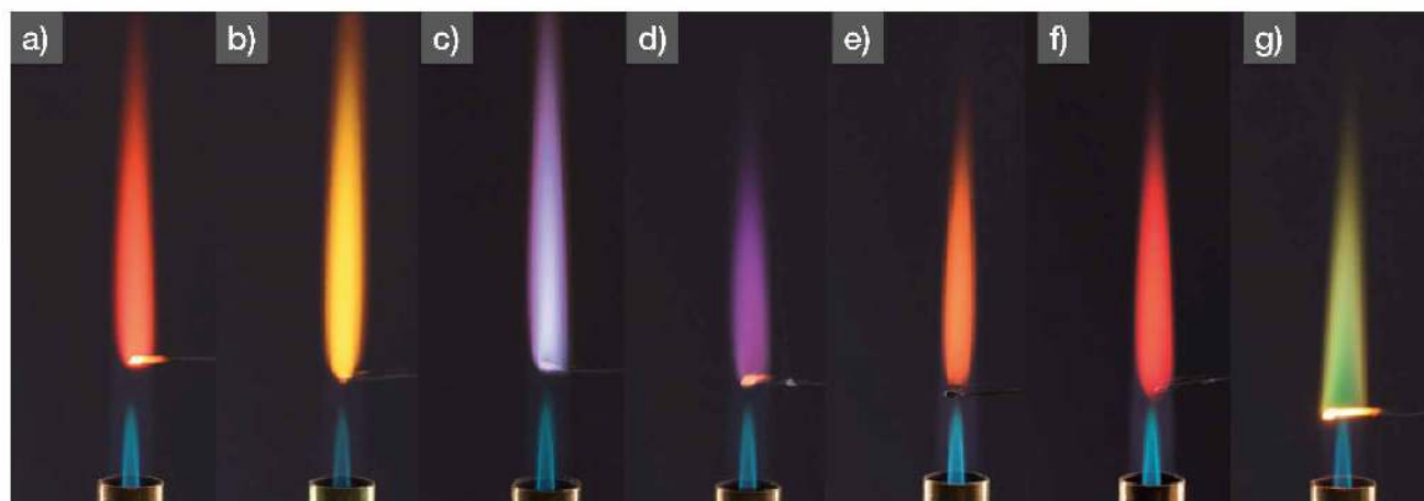
Fot. 144. Barwy płomieni kationów: a) litu, b) sodu, c) potasu, d) cezu, e) wapnia, f) strontu, g) baru.
