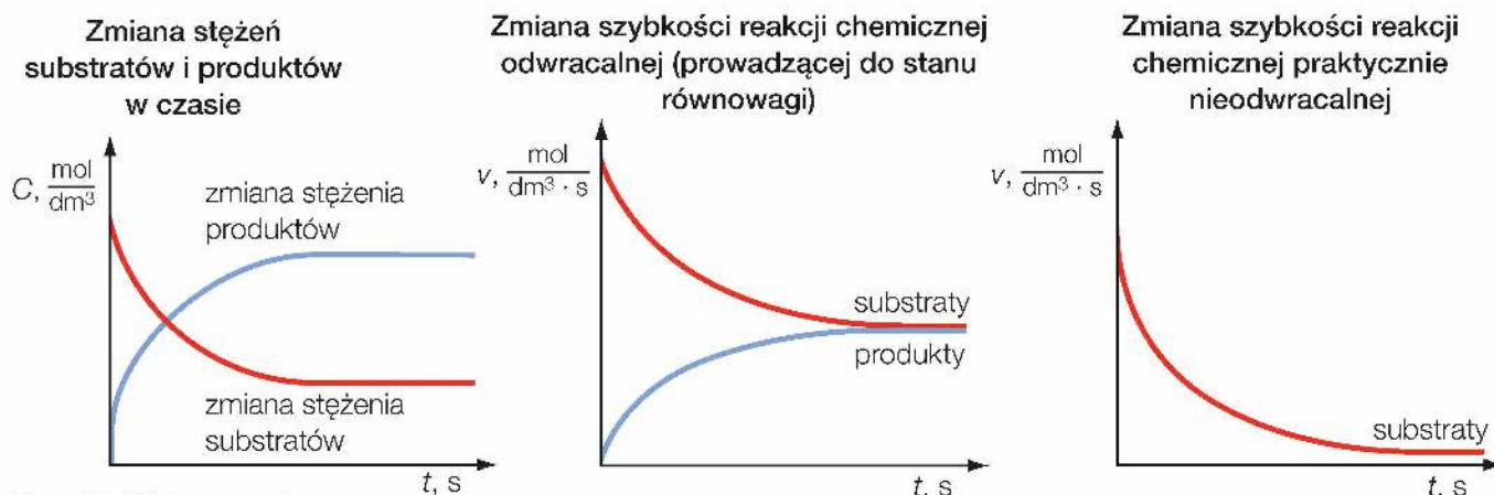
Rys. 55. Wykresy zmian stężenia lub szybkości reakcji chemicznej w czasie.
