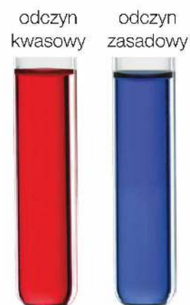
Fot. 137. Barwa wskaźnika – błękitu tymolowego – w roztworach kwasów i zasad.
