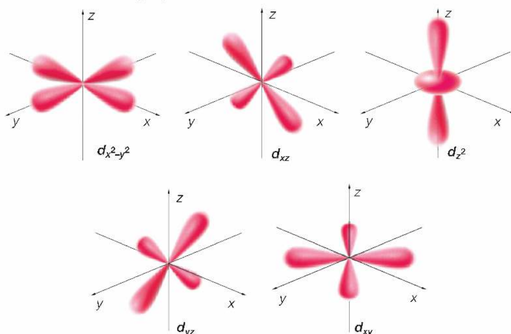
Rys. 11. Modele kształtów orbitali atomowych typu d .
