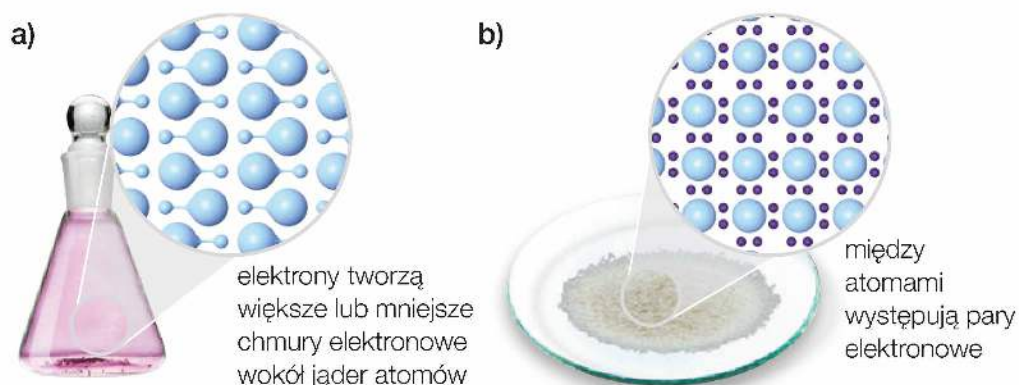
Fot. 18. Model struktury kryształów: a) cząsteczkowych, b) kowalencyjnych.
