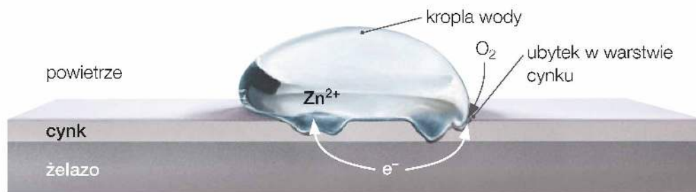
Rys. 50. Anoda tworzy się na warstwie cynkowej. Jony cynku przechodzą do kropli wody, jednak nie zostają dalej utlenione. Gdy w powłoce cynkowej powstaną ubytki, tlen pochodzący z powietrza może dotrzeć do warstwy żelaznej, na której wytworzy się katoda. Dzięki elektronom swobodnie przepływającym z anody zachodzi redukcja tlenu.
