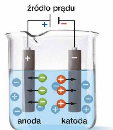
Rys. 51. Elektrody – podstawowe elementy elektrolizera – są zanurzone w wodnym roztworze elektrolitu lub stopionym elektrolicie.
