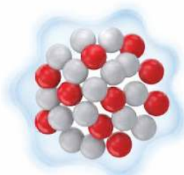
jądro z nadmiarem energii
