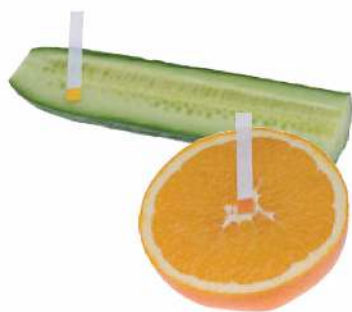
Fot. 129. Sok z ogórka ma odczyn obojętny (żółta barwa uniwersalnego papierka wskaźnikowego), a sok z pomarańczy – kwasowy (pomarańczowa barwa uniwersalnego papierka wskaźnikowego).
