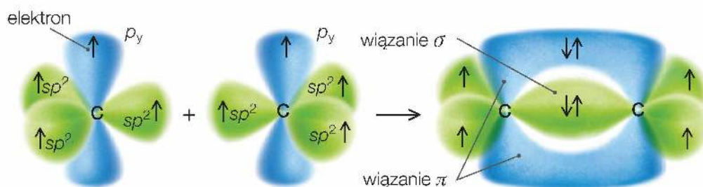
Rys. 40. Model tworzenia się wiązania \text{C}=\text{C} .
