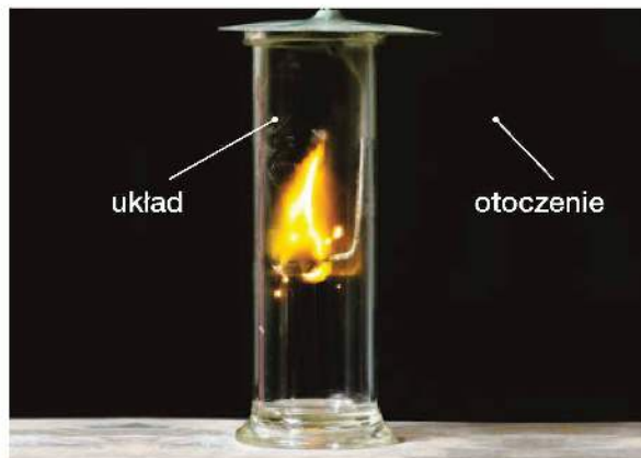
Fot. 102. Spalanie substancji w tlenie.
