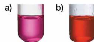
Fot. 32. Malinowa barwa fenoloftaleiny świadczy o odczynie zasadowym – a), natomiast czerwona barwa oranżu metylowego o odczynie kwasowym – b).
