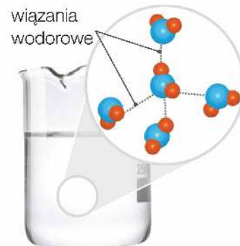
Fot. 15. Cząsteczki wody są połączone wiązaniami wodorowymi.
