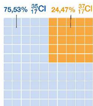
Rys. 19. Skład procentowy chloru.
