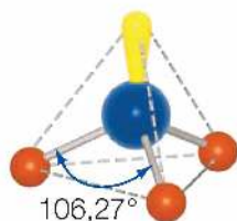
Rys. 44. Przestrzenna budowa cząsteczki amoniaku.
