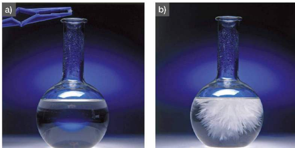
Fot. 92. Dodanie niewielkiego kryształka octanu sodu (zarodka krystalizacji) do jego przesyconego roztworu (a) powoduje błyskawiczną krystalizację nadmiaru soli (b).
