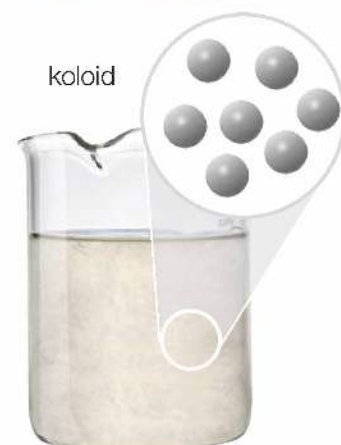
Fot. 83. Roztwory właściwe i koloidy różnią się wielkością cząstek substancji rozpuszczonej.
