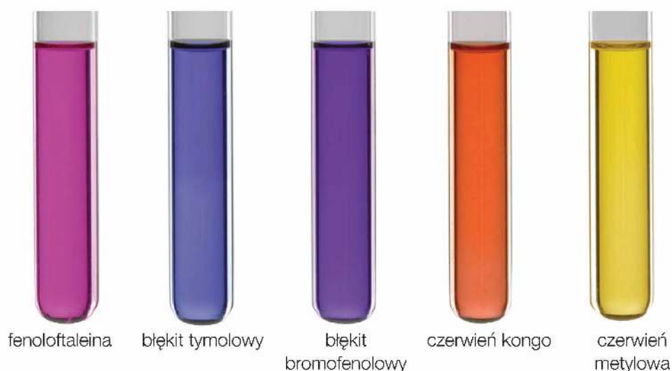
Fot. 38. Barwy różnych wskaźników kwasowo-zasadowych w roztworach o odczynie zasadowym.
