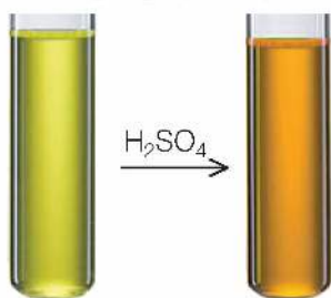
Fot. 174. Powstanie jonów dichromianowych.
