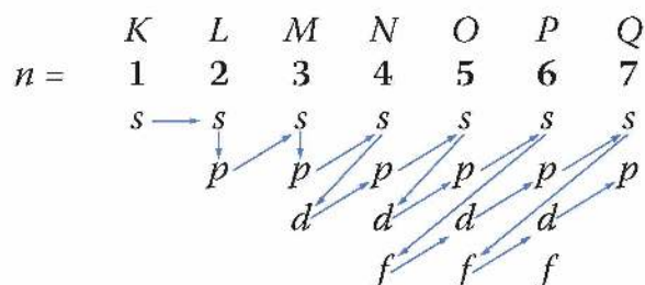
Rys. 15. Kolejność wypełniania podpowłok elektronowych przez elektrony – zgodnie ze wzrostem energii.
