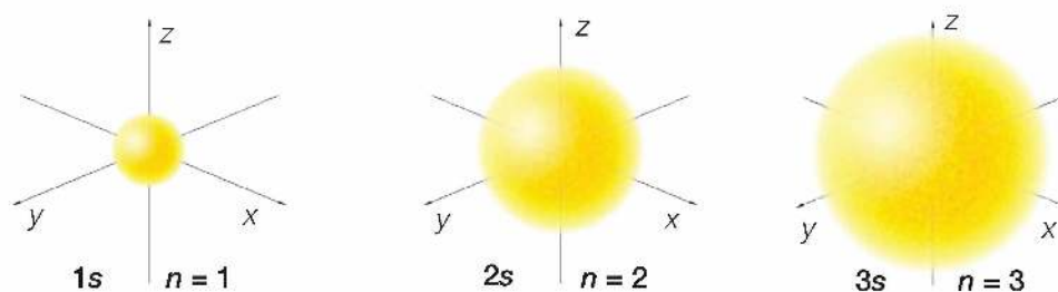
Rys. 12. Orbitale s mają kształt kuli, a ich promień są tym większe, im większa jest wartość n .
