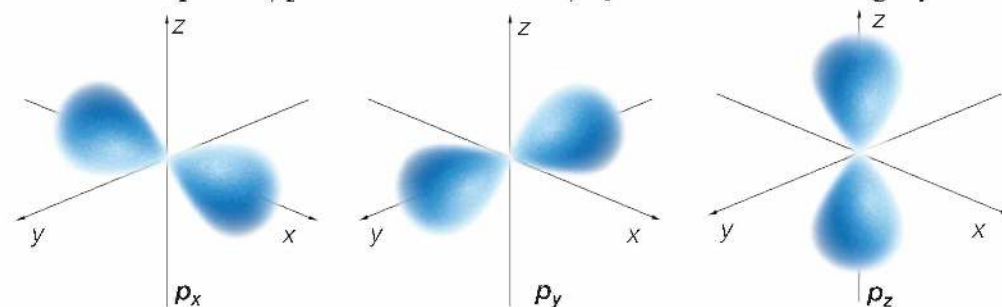
Rys. 10. Modele kształtów orbitali atomowych typu p .
