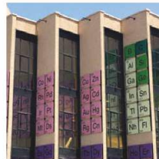
Fot. 10. Układ okresowy na budynku Uniwersytetu w Murcji.
