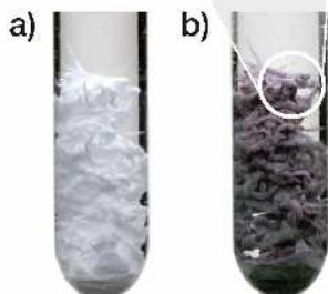
Fot. 136. Praktycznie nierozpuszczalny w wodzie biały chlorek srebra(I) (a) pod wpływem światła ciemnieje (b).
