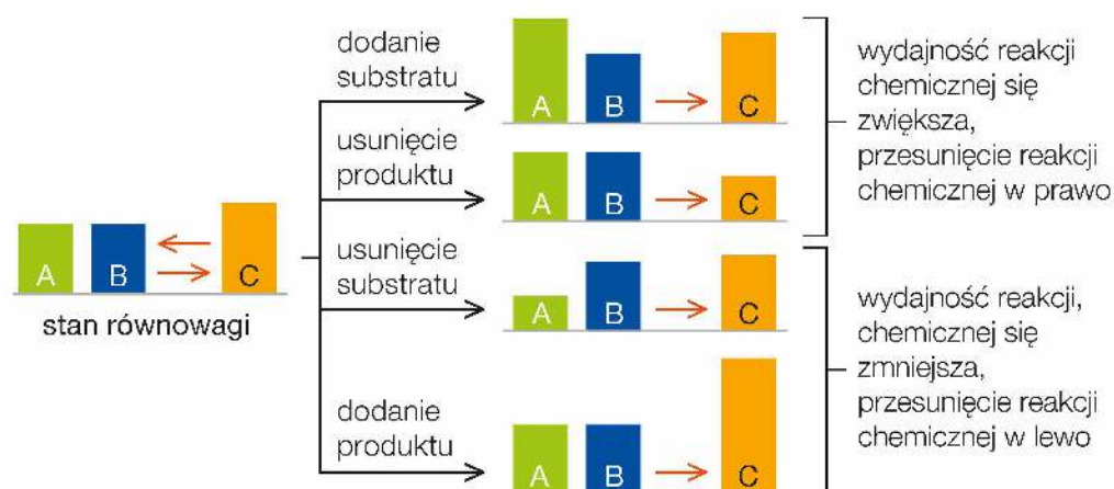
Rys. 59. Wpływ zmiany stężenia substratów lub produktów na stan równowagi chemicznej.
