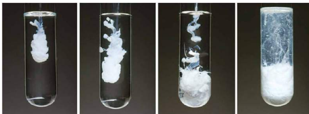
Fot. 117. Reakcja strącania chlorku srebra(I).
