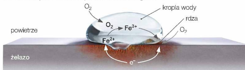
Rys. 49. Powstające na anodzie kationy \text{Fe}^{2+} zostają utlenione w kropli wody do jonów \text{Fe}^{3+} , następnie tworzy się z nich rdza (m.in. \text{Fe}_2\text{O}_3 ). Jednocześnie uwolnione elektrony swobodnie przepływają przez metal do katody, gdzie dzięki nim zachodzi redukcja tlenu pochodzącego z powietrza.
