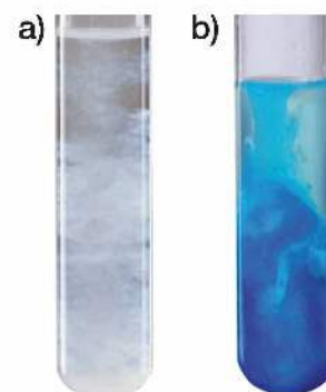
Fot. 135. Osady wodorotlenku glinu (a) oraz wodorotlenku miedzi(II) (b) powstają w reakcji zasad z odpowiednimi solami.
