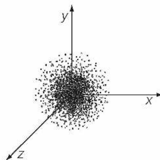
Rys. 7. Chmura elektronowa nie ma wyraźnej granicy zewnętrznej. Jednak im dalej od jądra atomowego, tym mniejsze jest prawdopodobieństwo znalezienia tam elektronu.
