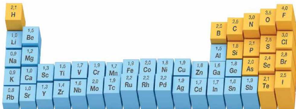
Rys. 25. Elektroujemność pierwiastków chemicznych wg skali Paulinga jest wielkością bezwymiarową (bez jednostki). Elektroujemności gazów szlachetnych nie podaje się ze względu na ich bierność chemiczną.
