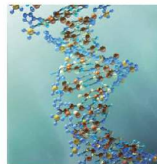
Rys. 32. DNA składa się z dwóch łańcuchów nukleotydów połączonych wiązaniami wodorowymi.
