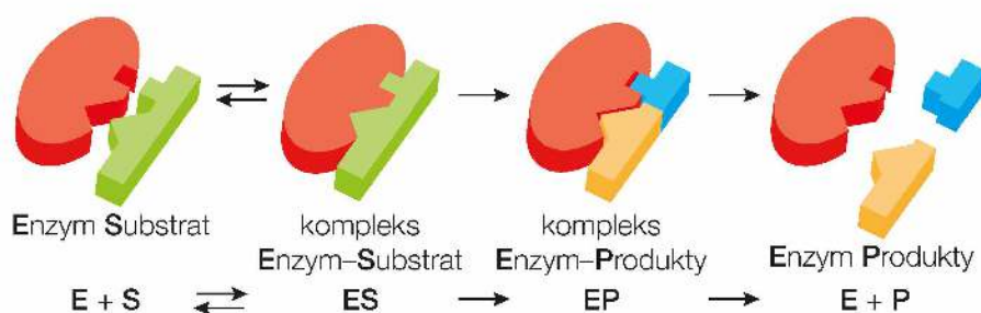
Rys. 58. Centrum aktywne enzymu odpowiada kształtem substratowi i sprawia, że może on szybciej przekształcić się w produkty.
