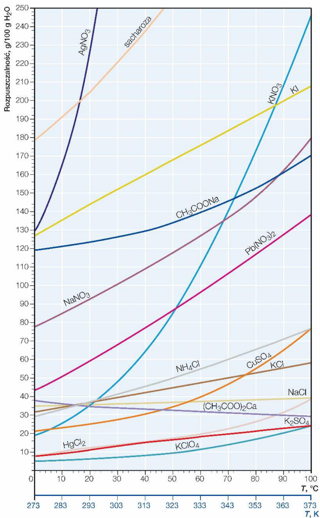
Rys. 52. Krzywe rozpuszczalności – zależność rozpuszczalności substancji stałych w wodzie od temperatury: \text{AgNO}_3 – azotan(V) srebra(I); KI – jodek potasu; \text{NaNO}_3 – azotan(V) sodu; \text{KNO}_3 – azotan(V) potasu; \text{Pb}(\text{NO}_3)_2 – azotan(V) ołowiu(II); \text{NH}_4\text{Cl} – chlorek amonu; \text{CuSO}_4 – siarczan(VI) miedzi(II); \text{K}_2\text{SO}_4 – siarczan(VI) potasu; KCl – chlorek potasu; NaCl – chlorek sodu; (\text{CH}_3\text{COO})_2\text{Ca} – etanian wapnia; \text{CH}_3\text{COONa} – etanian sodu; \text{HgCl}_2 – chlorek rtęci(II); \text{KClO}_4 – chloran(VII) potasu; sacharoza – \text{C}_{12}\text{H}_{22}\text{O}_{11} .
