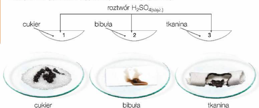
Fot. 163. Wpływ stężonego roztworu kwasu siarkowego(VI) na cukier, bibułę i tkaninę.
