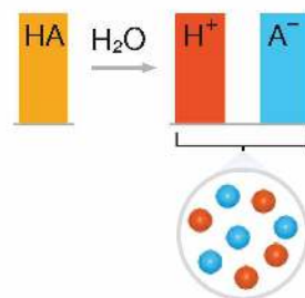
Rys. 60. Dysocjacja mocnego kwasu jednoprotowego.
