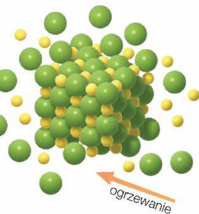
Rys. 35. Model stapiania NaCl – pod wpływem ogrzewania jony \text{Na}^+ i \text{Cl}^- są uwalniane z sieci krystalicznej soli.
