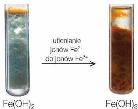
Fot. 180. Powstawanie czerwono-brunatnego osadu wodorotlenku żelaza(III).
