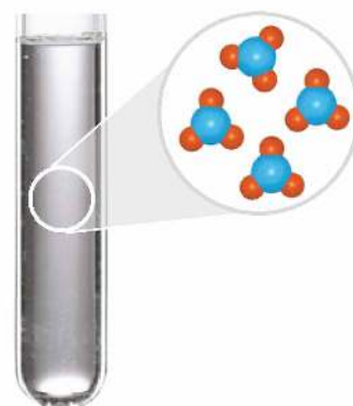
Fot. 121. W roztworach kwasów znajdują się jony \text{H}_3\text{O}^+ .
