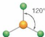
Rys. 38. Wiązania chemiczne w cząsteczce fluorku boru.
