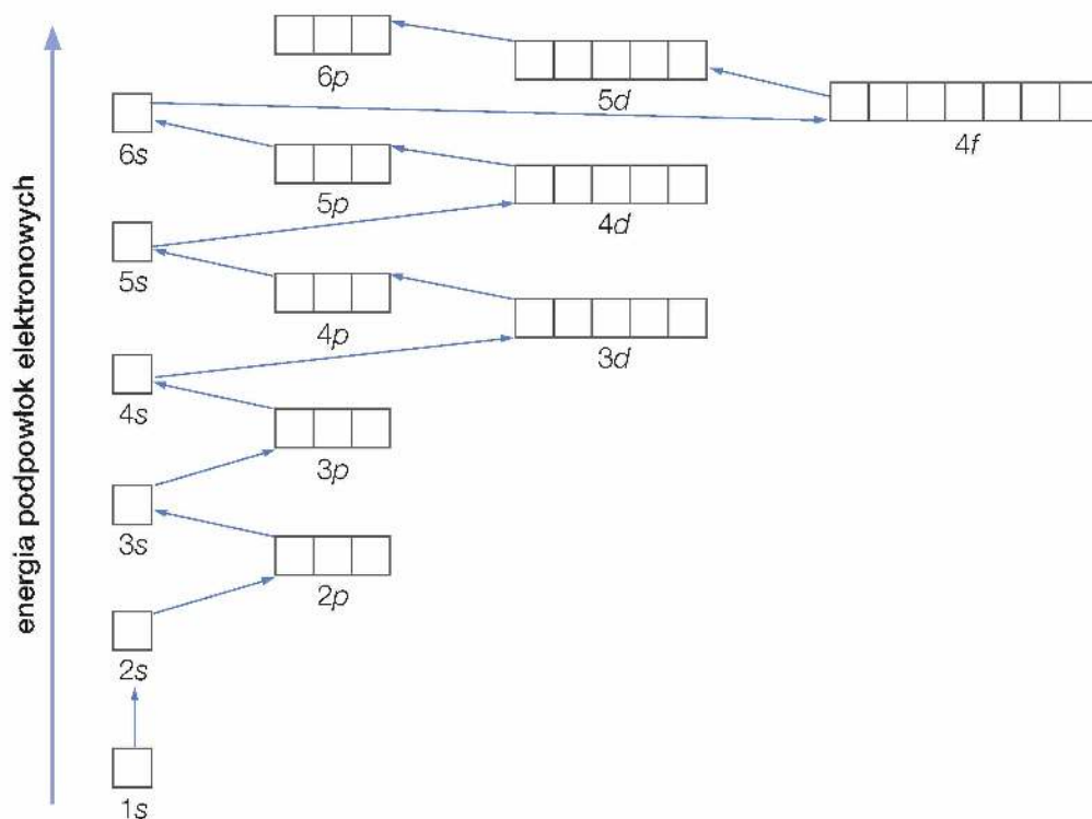
Rys. 16. Podpowłoki elektronowe są zapełniane przez elektrony w takiej kolejności, w jakiej wzrasta ich energia.
