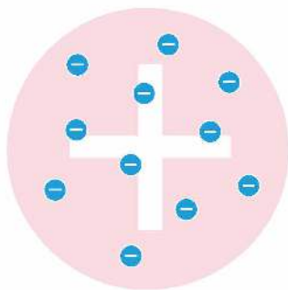
Rys. 2. Model atomu Thomsona.
