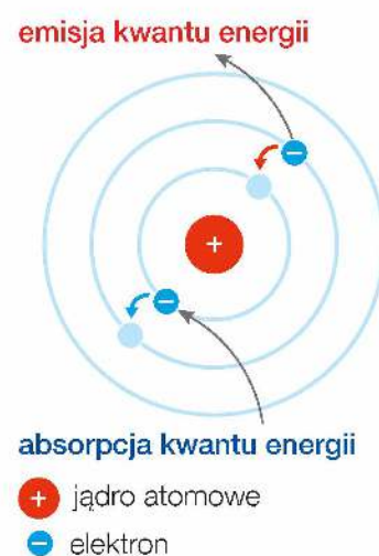
Rys. 4. Model atomu Bohra.
