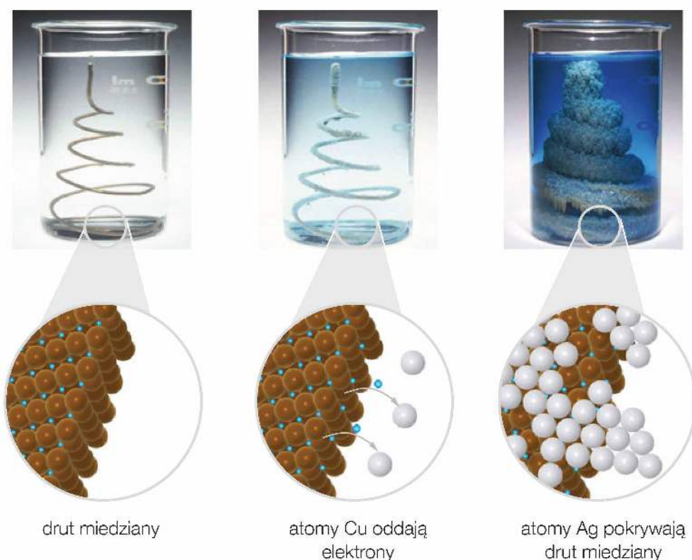
Fot. 71. Reakcja miedzi z azotanem(V) srebra(I).
