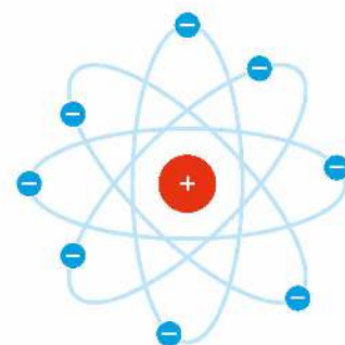
Rys. 3. Planetarny model atomu – model Rutherforda.
