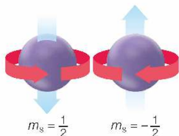
Rys. 13. Model spinu elektronu, który można sobie wyobrazić jako wirowanie elektronu wokół własnej osi.
