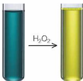
Fot. 173. Utlennianie jonów chromu(III) do jonów chromu(VI).
