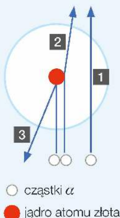
Rys. 5. Schemat przedstawiający eksperyment Rutherforda.
