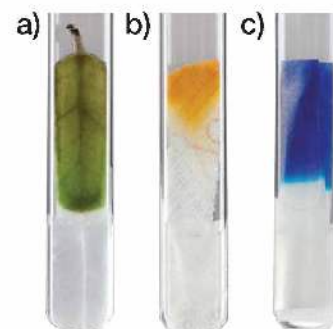
Fot. 168. Wpływ wody chlorowej na barwniki w: a) liściu, b) tkaninie, c) atramencie.
