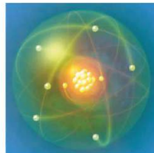
Rys. 6. Modelowe wyobrażenie atomu tlenu – elektrony poruszają się wokół jądra atomowego i nie można im przyporządkować stałego położenia.
