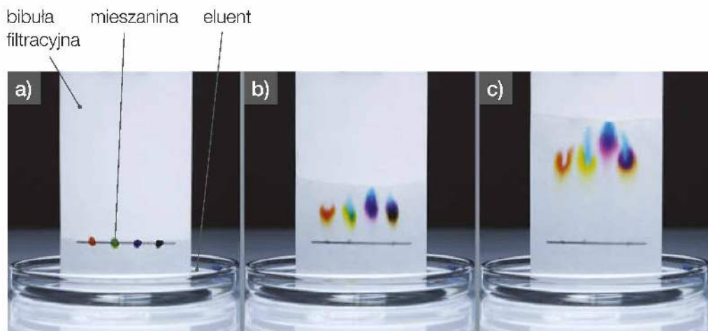
Fot. 12. Mieszaninę substancji rozdzielanych nanosi się na bibułę filtracyjną, którą następnie umieszcza się w zlewce z eluentem – a). Eluent rozpuszcza poszczególne składniki mieszaniny, a wędrując wzdłuż fazy stacjonarnej, powoduje ich przesuwanie się – b). Poszczególne składniki mieszaniny zatrzymują się na różnej wysokości bibuły filtracyjnej – c).
