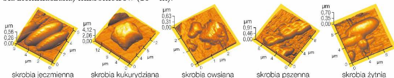
Rys. 62. Przykłady ziaren skrobi pochodzących z różnych roślin, zobrazone metodą mikroskopii sił atomowych (AFM).
