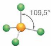
Rys. 4. Wiązania chemiczne w cząsteczce metanu.
