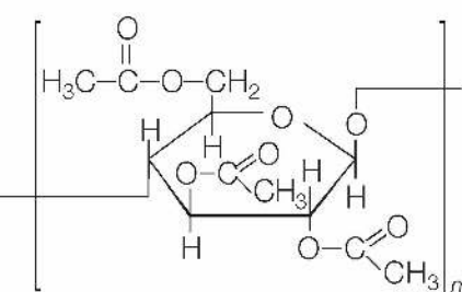
wzór półstrukturalny trioctanu celulozy
