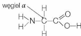
wzór kwasu aminoetanowego
