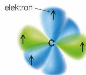
Rys. 12. Model hybrydyzacji sp orbitali atomowych węgla.
