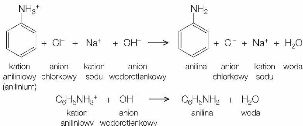
Fot. 126. Produktem reakcji chemicznej jest oleista ciecz.
