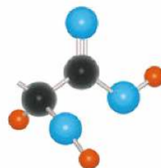
Rys. 55. Model fragmentu cząsteczki hydroksykwasu.
