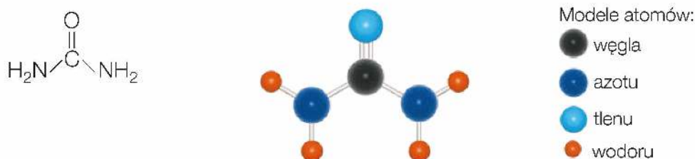
Fot. 133. Kryształy mocznika.
