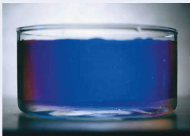
Barwa światła spolaryzowanego odchylonego o kąt 75° .
