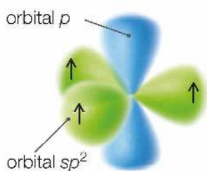
Rys. 17. Model hybrydyzacji sp^2 orbitali atomowych węgla.
