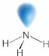
Rys. 52. Rozmieszczenie wiązań N–H w amoniaku i aminach odpowiada hybrydyzacji sp^3 atomu azotu.
