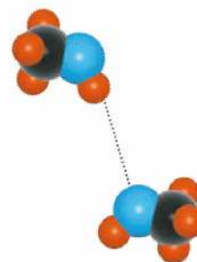
Rys. 35. Model wiązania wodorowego między polarnymi cząsteczkami metanolu.
