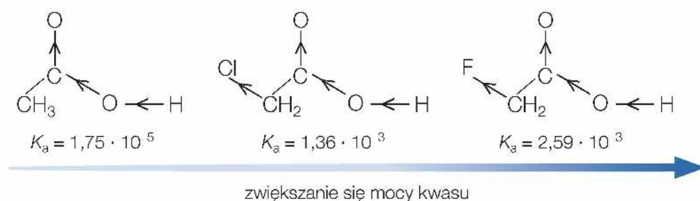
Rys. 42. Kierunek przemieszczania się elektronów w cząsteczkach kwasów: etanowego, chloroetanowego oraz fluoroetanowego.
