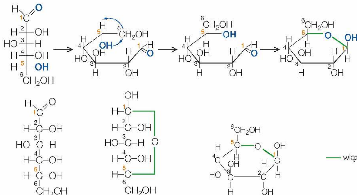
wzór liniowy D-glukozy wzór pierścieniowy D-glukozy wzór taflowy D-glukozy
