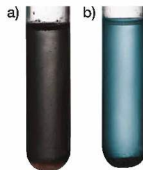
Fot. 92. Pod wpływem ogrzewania kwasu etanowego z tlenkiem miedzi(II) (a) powstaje roztwór o barwie niebieskiej (b).
