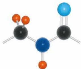
Rys. 58. W cząsteczkach białek występują wiązania peptydowe.
