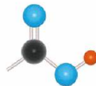
Rys. 41. Model grupy karboksylowej.
