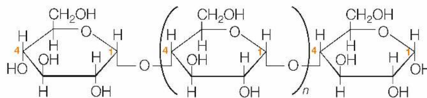
fragment cząsteczki amylozy
