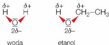
Rys. 34. Porównanie budowy cząsteczek wody i etanolu.
