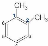
1,2-dimetylobenzen ortoksylen o -ksylen
