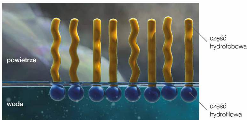
Rys. 47. Ustawienie cząsteczek substancji powierzchniowo czynnej na granicy faz woda–powietrze.
