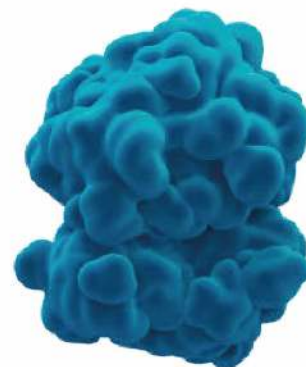
Rys. 59. Model rybosomu. W rybosomach aminokwasy łączą się wiązaniem peptydowym.
