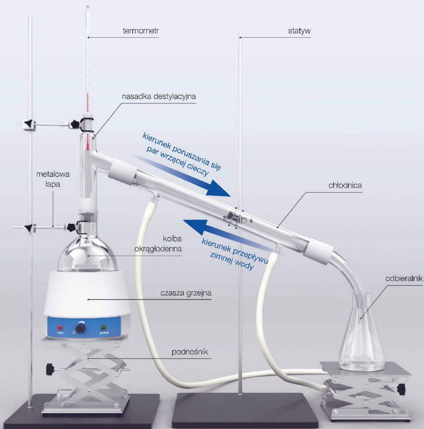
zestaw do destylacji
