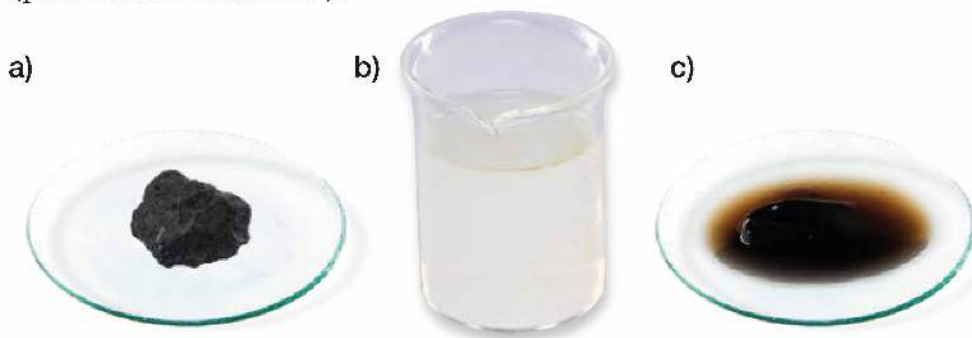
Fot. 48. Produkty pirolizy węgla kamiennego: a) koks, b) woda pogazowa, c) smoła węglowa.
