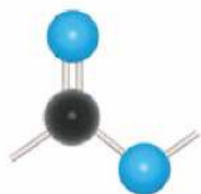
Rys. 48. Model grupy estrowej.
