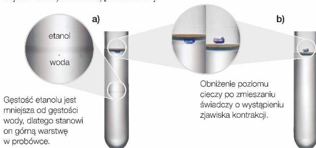
Fot. 62. Mieszanie etanolu z wodą: a) objętość przed wymieszaniem; b) zmniejszenie objętości po wymieszaniu.
