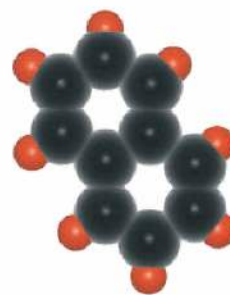
Rys. 22. Model cząsteczki naftalenu.
