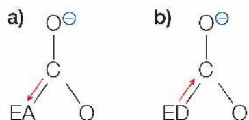
Rys. 43. Kierunek przemieszczania się elektronów w anionie karboksylanowym podstawionym: a) stabilizującą grupą elektronoakceptorową, b) destabilizującą grupą elektronodonorową.
