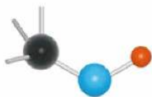
Rys. 33. Model grupy hydroksylowej, która jest grupą funkcyjną alkoholi.
