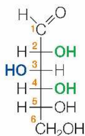
D-glukoza wzór Fischera
