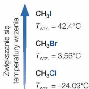
Rys. 27. Zmiana temperatury wrzenia pochodnych metanu wraz ze zwiększaniem się masy atomowej fluorowca w cząsteczce.
