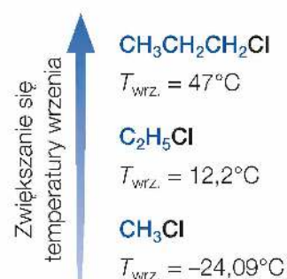
Rys. 28. Zmiana temperatury wrzenia chloroalkanów.
