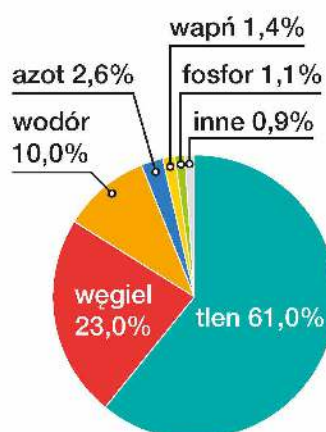
Rys. 1. Pierwiastki chemiczne, których zawartość w organizmie człowieka jest mniejsza niż 1% masy, to m.in.: S, Na, K, Cl, Mg, Si.
