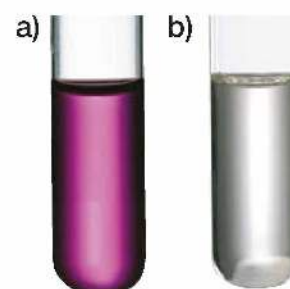
Fot. 93. Reakcja kwasu etanowego z wodorotlenkiem sodu: a) fenoloftaleina w roztworze zasady sodowej ma barwę malinową, b) pod wpływem kwasu etanowego roztwór odbarwia się.
