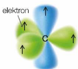
Rys. 8. Model hybrydyzacji sp^2 orbitali atomowych węgla.
