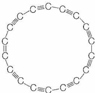
Rys. 2. Wzór strukturalny cząsteczki cyklokarbonu.
