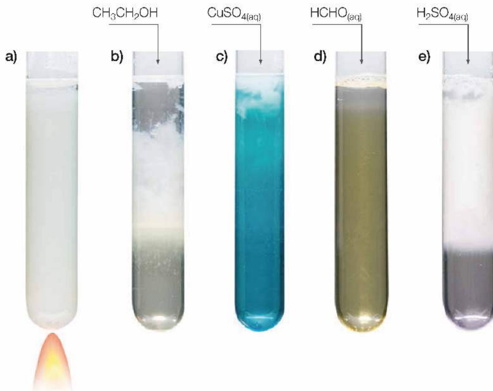
Fot. 153. Wpływ na białko: a) podwyższonej temperatury, b) roztworu \text{CH}_3\text{CH}_2\text{OH} , c) roztworu \text{CuSO}_4 , d) roztworu \text{HCHO} , e) stężonego roztworu \text{H}_2\text{SO}_4 .
