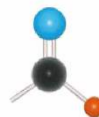
Rys. 39. Model grupy aldehydowej, która jest grupą funkcyjną aldehydów.
