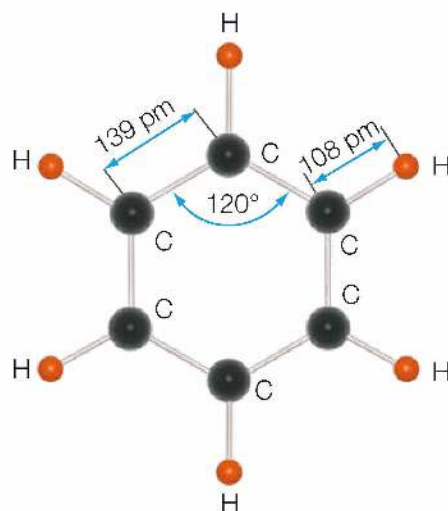
Rys. 16. Model budowy cząsteczki benzenu.
