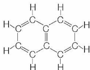
wzór strukturalny naftalenu
