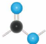
Rys. 49. Model grupy estrowej.
