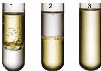
Fot. 115. Badanie rozpuszczalności oleju roślinnego w wodzie, etanolu i benzynie.
