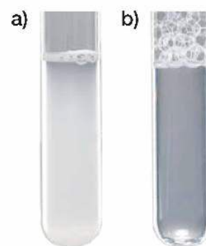
Fot. 98. Zachowanie mydła w wodzie: a) twardej, b) miękkiej.
