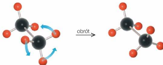
Rys. 23. Konformacje etanu.
