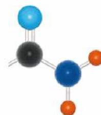
Rys. 53. Model fragmentu cząsteczki amidu.
