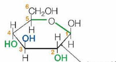
D-glukoza wzór Hawortha
