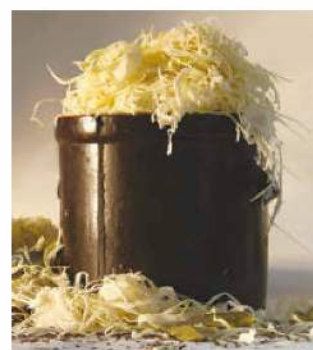
Fot. 142. Kwas D-(–)-mlekowy jest produktem fermentacji mlekowej sacharydów, m.in. w procesach kiszenia kapusty, ogórków czy mleka. Kwas L-(+)-mlekowy powstaje podczas pracy mięśni, powodując tzw. zakwasy.
