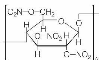
wzór półstrukturalny triazotanu(V) celulozy
