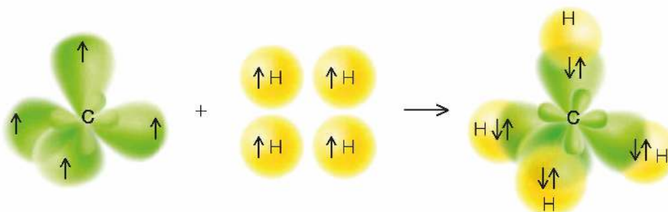
Rys. 5. Model tworzenia się cząsteczki metanu.
