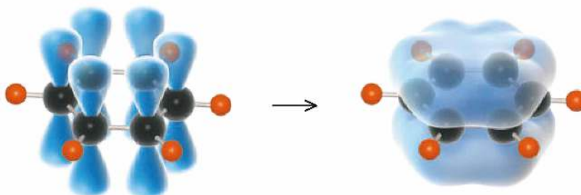
Rys. 18. Model tworzenia zdelokalizowanych orbitali typu \pi (zdelokalizowane wiązanie typu \pi ).
