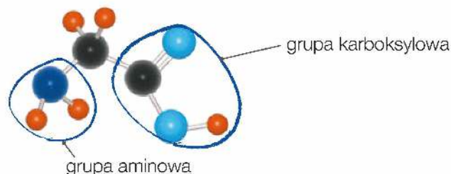
model cząsteczki kwasu aminoetanowego
