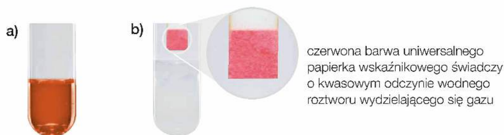
Fot. 75. Woda bromowa: a) przed reakcją chemiczną, b) po dodaniu fenolu.
