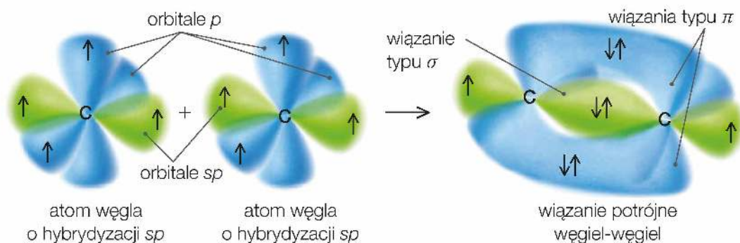
Rys. 13. Model tworzenia się wiązań typu \sigma i typu \pi między atomami węgla wchodzącymi w skład cząsteczki alkinu.
