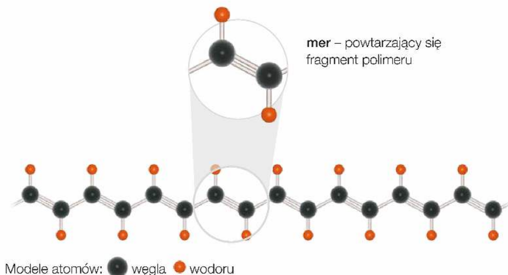
Rys. 14. Model fragmentu cząsteczki poliacetyleny.
