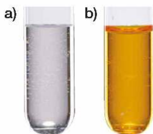
Fot. 149. Reakcja kwasu aminoetanowego: a) z roztworem NaOH i fenoloftaleiny, b) z roztworem HCl i oranżu metylowego.
