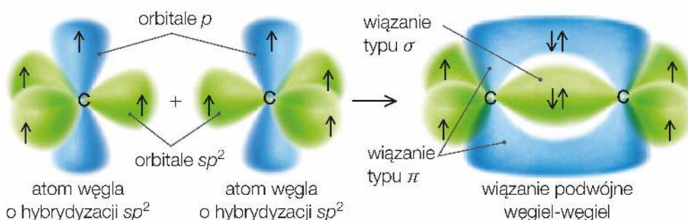
Rys. 9. Model tworzenia wiązań typu \sigma i typu \pi między atomami węgla wchodzącymi w skład cząsteczki alkeny.
