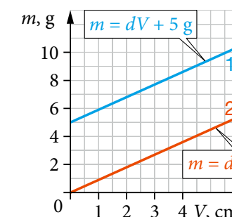
Rys. 1.19. Wykres zależności masy oleju od jego objętości z uwzględnieniem naczynia (1) lub bez naczynia (2)
