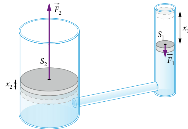
Rys. 6.8. Małe przesunięcie dużego tłoka otrzymujemy przez duże przesunięcie małego tłoka
