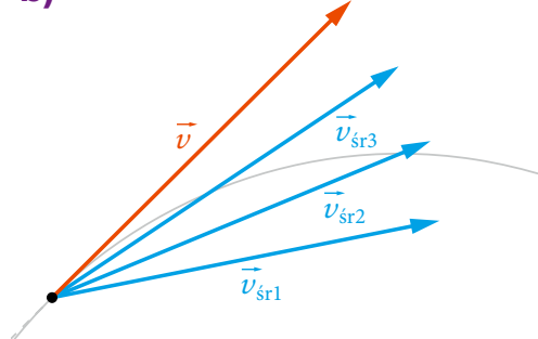
Rys. 3.2. Wektory przemieszczenia \Delta \vec{r} (a) odpowiadają coraz krótszym przedziałom czasu, a wektory prędkości średniej \vec{v}_{sr} (b) są skierowane tak samo jak odpowiadające im wektory przemieszczenia
