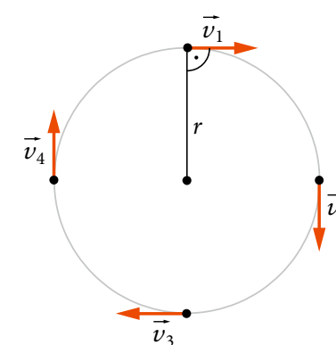
Rys. 3.18. Wektor prędkości w ruchu po okręgu jest styczny do okręgu
