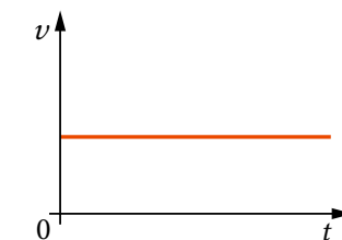
Rys. 2.13. Wykres zależności v(t) dla ruchu jednostajnego prostoliniowego
