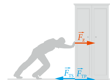
Rys. 4.16. Podłoga działa na szafę siłą tarcia \vec{F}_{TS} , która równoważy przyłożoną do szafy siłę zewnętrzną \vec{F}_z . Szafa także działa na podłogę siłą tarcia \vec{F}_{TP}
