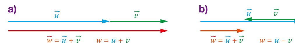
Rys. 1.29. Dodawanie i odejmowanie wektorów o jednakowych kierunkach: a) jednakowe zwroty – wartości się dodaje, b) przeciwnie zwroty – wartości się odejmują
