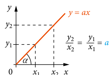
Rys. 1.16. Wykres proporcjonalności prostej y = ax
