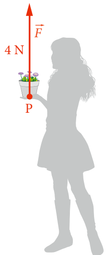
Rys. 1.25. Dziewczyna działa na doniczkę siłą skierowaną do góry
