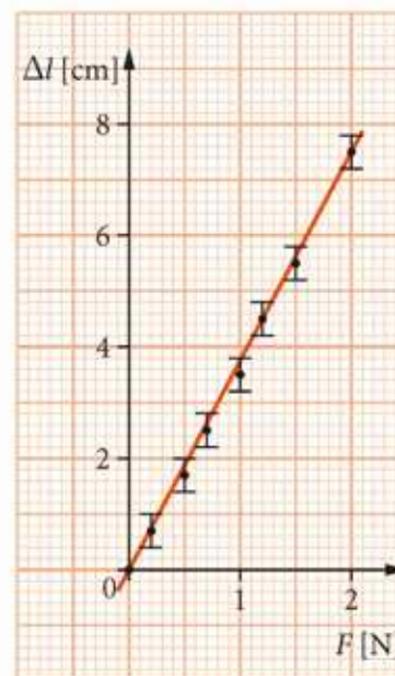
▲ Wykres zależności wydłużenia sprężyny od siły rozciągającej
