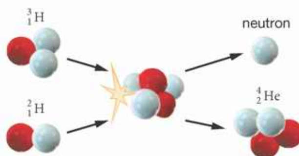
▲ Reakcja syntezy jąder trytu i deuteru
