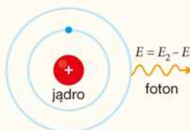
▲ Atom po emisji fotonu
