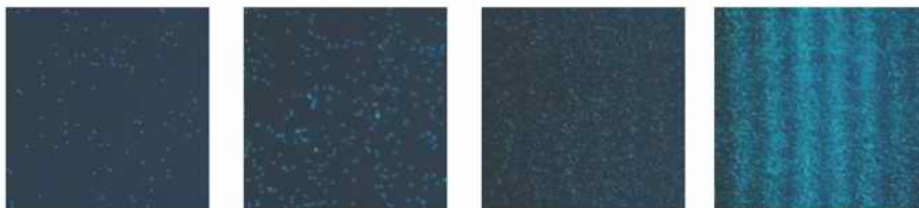
▲ Tworzenie obrazu interferencyjnego przez elektrony. Kolejne zdjęcia powstawały w miarę upływu czasu, po uderzeniu coraz większej liczby elektronów
