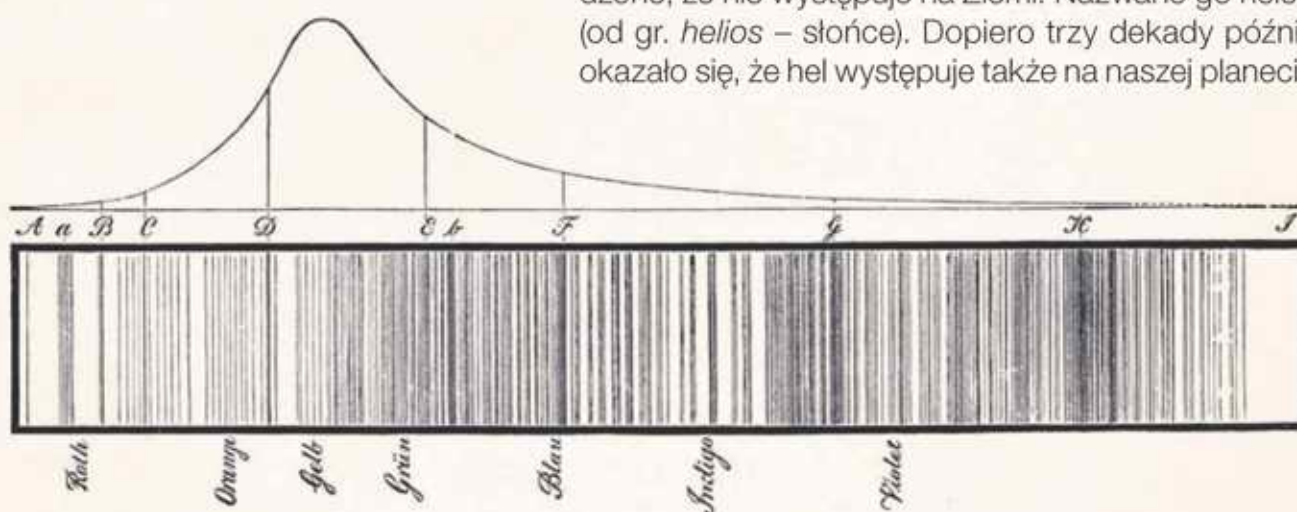
▲ Rysunek sporządzony przez Fraunhofera przedstawiający widmo słoneczne
