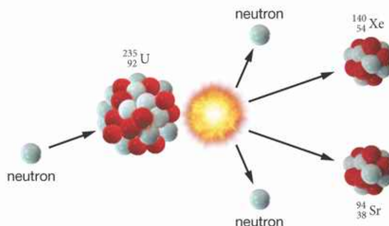
▲ Rozszczepienie jądra uranu
