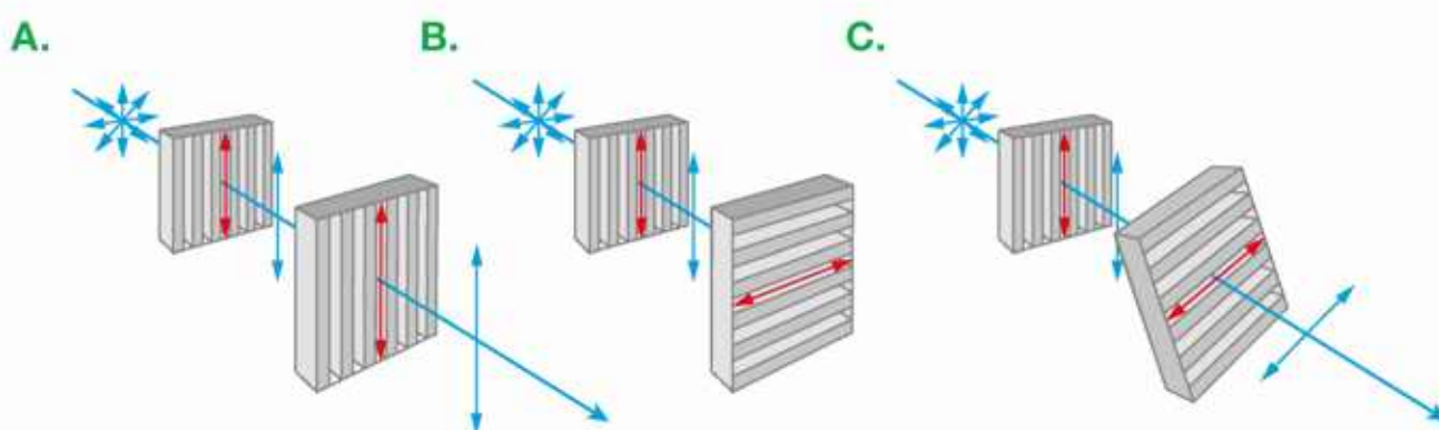
▲ Przejście światła przez dwa kolejne polaryzatory
