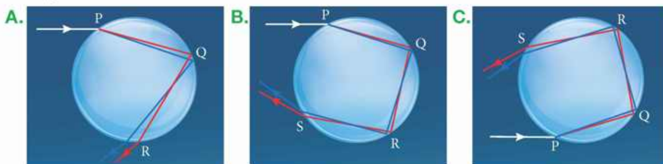
▲ Powstawanie drugiej (zewnętrznej) tęczy
