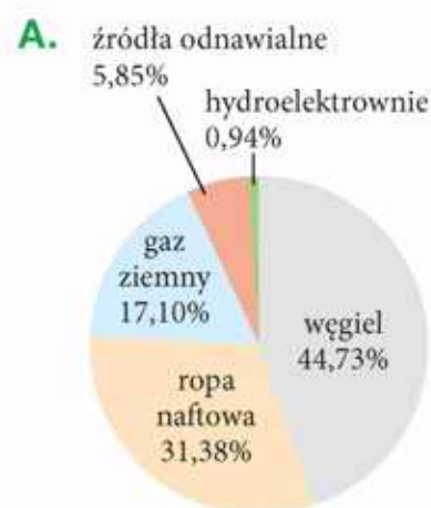
▲ Źródła energii w Polsce w 2019 r.
