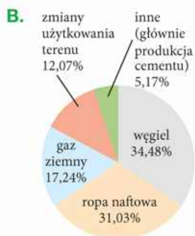
▲ Roczna emisja \text{CO}_2 spowodowana przez działalność człowieka (średnio na świecie)
