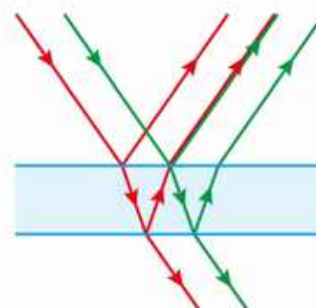
▲ Interferencja na błonie bańki mydlanej; kolory promieni służą tylko ich rozróżnieniu na rysunku, w rzeczywistości są to promienie światła białego
