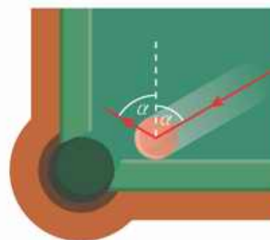
▲ Prawo odbicia dla kul bilardowych
