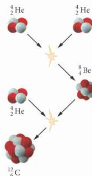
▲ Schemat reakcji przemiany helu w węgiel
