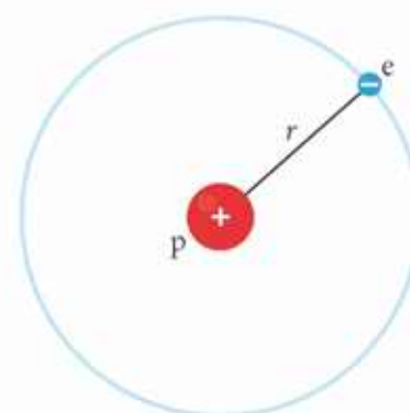
▲ Atom wodoru według Bohra
