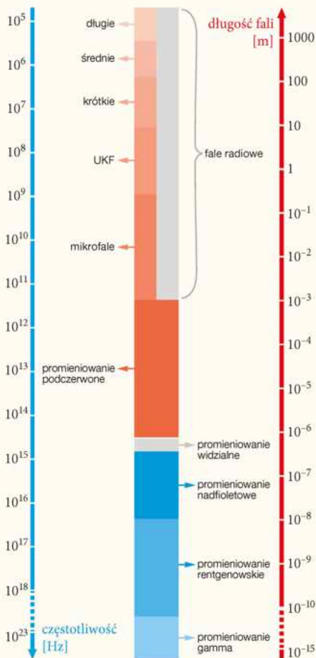
▲ Widmo fal elektromagnetycznych
