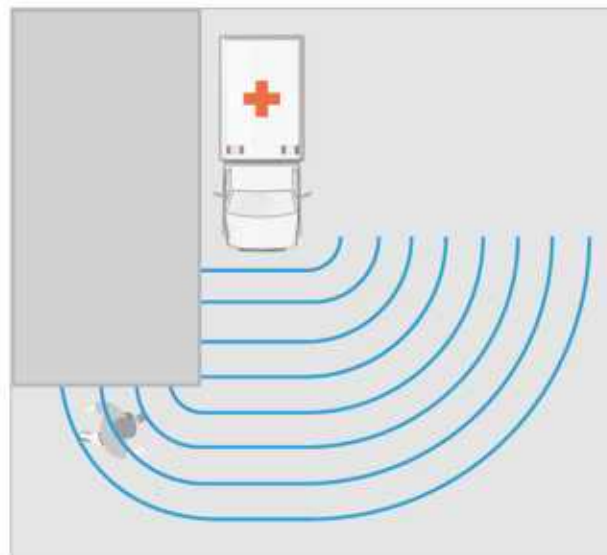
▲ Ugięcie fal dźwiękowych na krawędzi budynku
