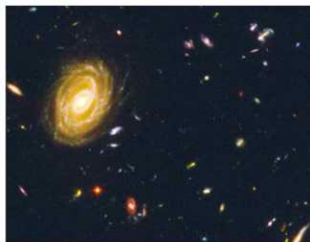
▲ Dzięki efektowi Dopplera został odkryty ruch galaktyk we Wszechświecie
