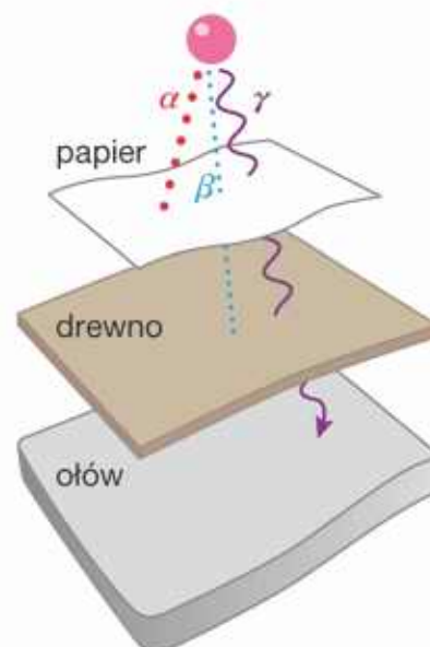
▲ Zasięg promieniowania alfa, beta i gamma
