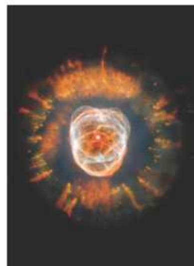
▲ Mglawica planetarna. Tak będzie wyglądać Słońce za ponad 7 mld lat
