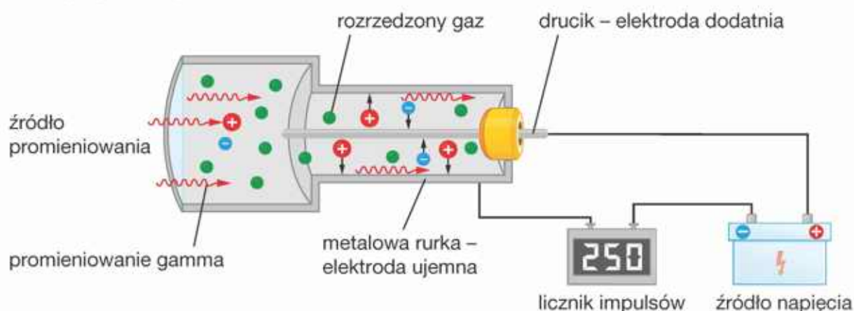
▲ Schemat licznika Geigera–Müllera
