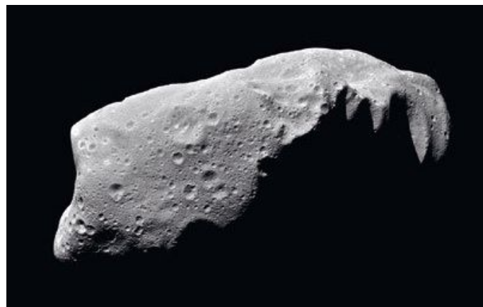
Planetoidy mają najczęściej nieregularny kształt. Jedną z nich jest Ida, która krąży w pasie głównym planetoid.
