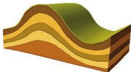
Fałd stojący.
