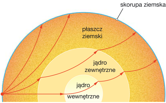
Analiza rozchodzenia się fal sejsmicznych dostarcza wielu informacji. Pozwala np. stwierdzić, gdzie znajdują się powierzchnie nieciągłości.
