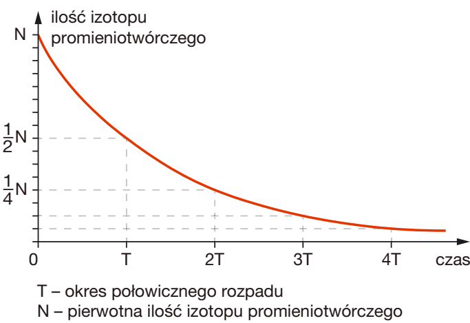
Za każdym razem, gdy upłynie okres połowicznego rozpadu, pierwiastka promieniotwórczego pozostaje dwa razy mniej.
