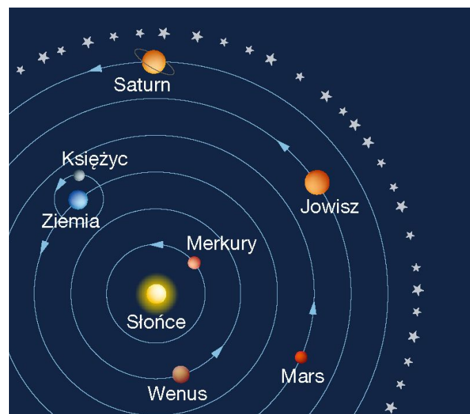
Heliocentryczny model wszechświata.
