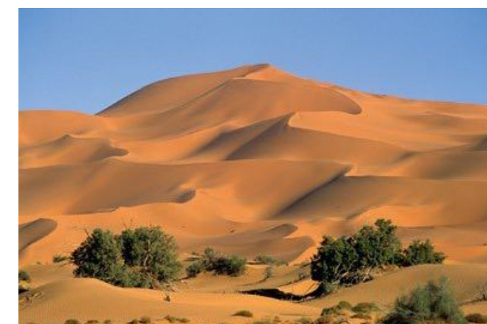
Wydmy na Saharze, we wschodniej Algierii, mają 5 km długości i ponad 450 m wysokości. To najwyższe wydmy w Afryce.
