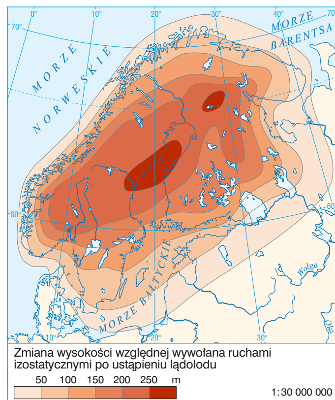
Ruchy izostatyczne na Półwyspie Skandynawskim po ustąpieniu lądolodu.
