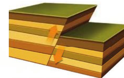
Uskok odwrócony.
