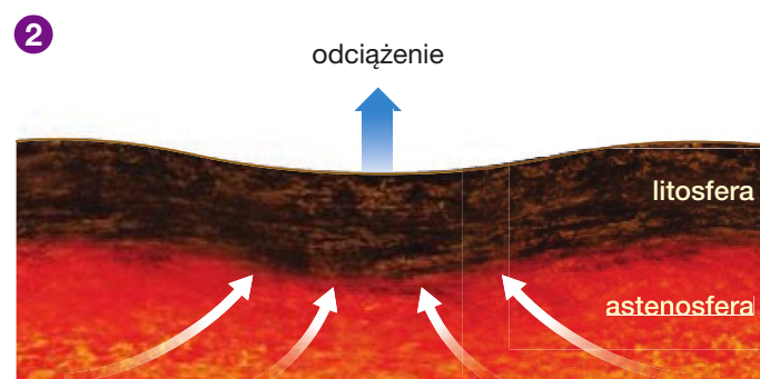
Ruchy izostatyczne związane z powstaniem i zanikiem lądolodu.
