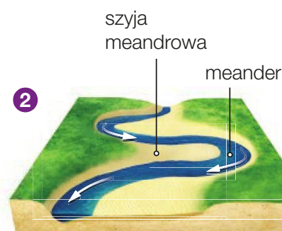
Ruch wody w korycie meandrowym.
