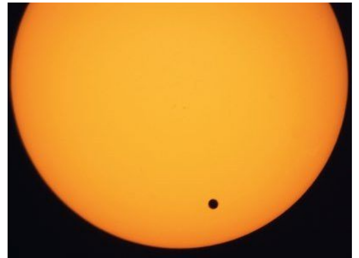
Tranzyt Wenus występuje wtedy, gdy znajduje się ona na tle tarczy Słońca. To zjawisko można zaobserwować, jeśli Słońce, Wenus i Ziemia ustawią się w jednej linii.
