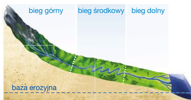
Profil podłużny rzeki.
