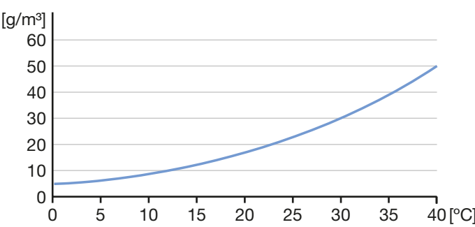
Zawartość pary wodnej w powietrzu w zależności od temperatury powietrza.
