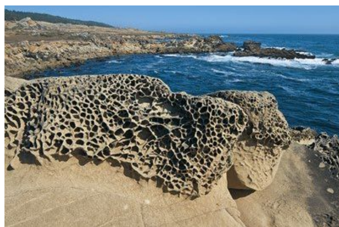
Na skutek wietrzenia chemicznego mogą powstawać tafoni – zagłębienia przypominające plastry miodu. Występują one np. na wybrzeżu Kalifornii.
