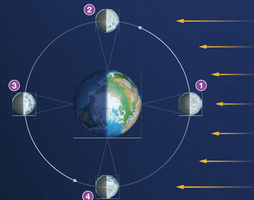
Położenie Księżyca względem Słońca i Ziemi
