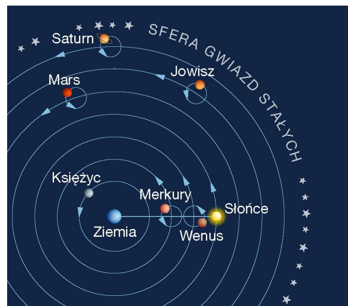
Geocentryczny model wszechświata.
