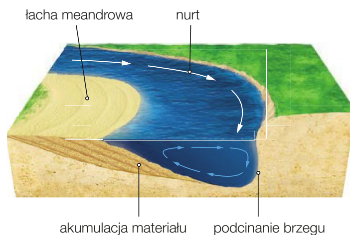
Ruch wody w korycie meandrowym.
