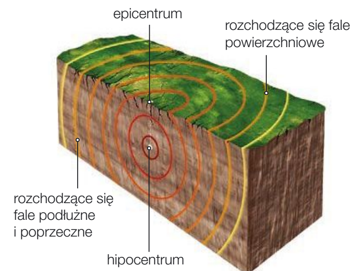
Rozchodzenie się fal sejsmicznych.
