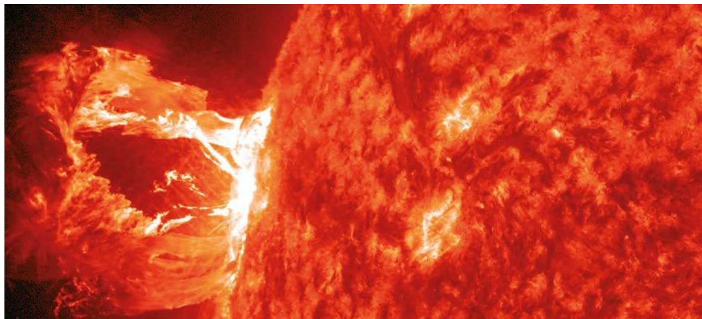
Przejawem aktywności Słońca są rozbłyski słoneczne, czyli wyrzuty ogromnej ilości energii w przestrzeń kosmiczną. Po raz pierwszy zaobserwowano je już w 1859 r.
