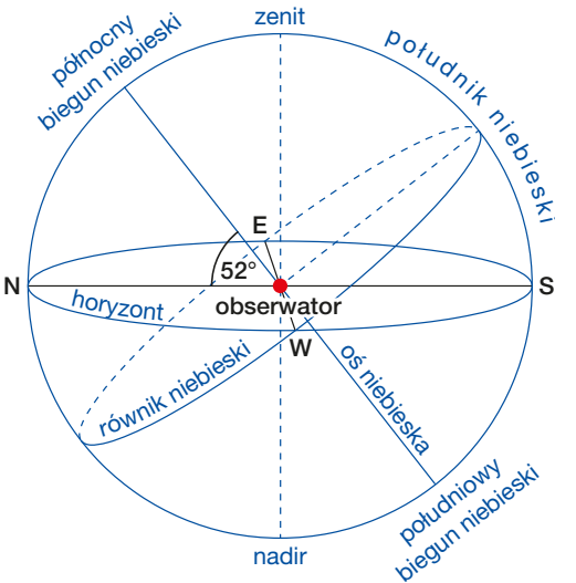
Układ horyzontalny dla szerokości geograficznej Warszawy.
