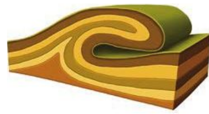
Fałd leżący.
