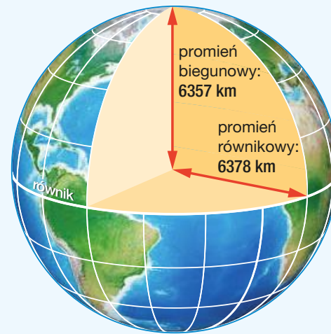
1 Spłaszczenie biegunowe Ziemi.
