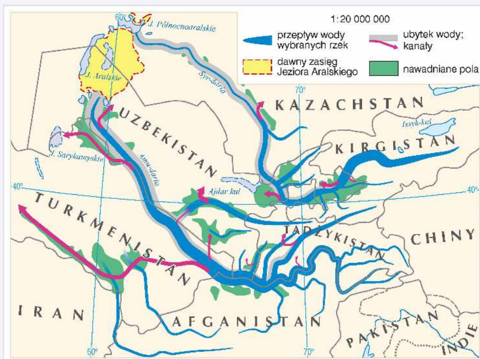
Obecnie w miejscu Jeziora Aralskiego znajduje się kilka mniejszych zbiorników.
