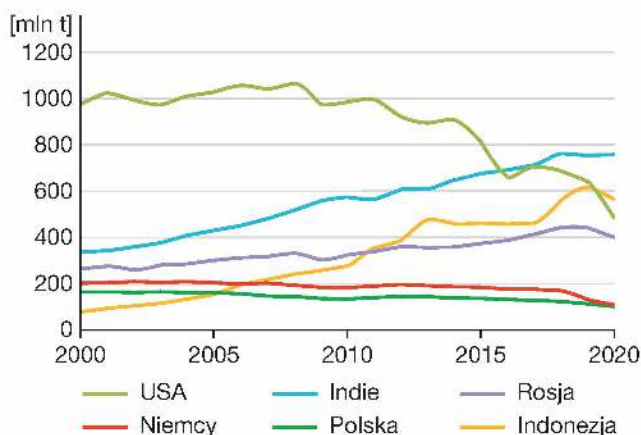
Wydobycie węgla w wybranych krajach w latach 2000–2020.
