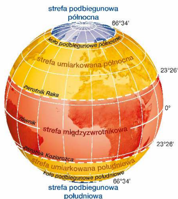
Strefy oświetlenia Ziemi.
