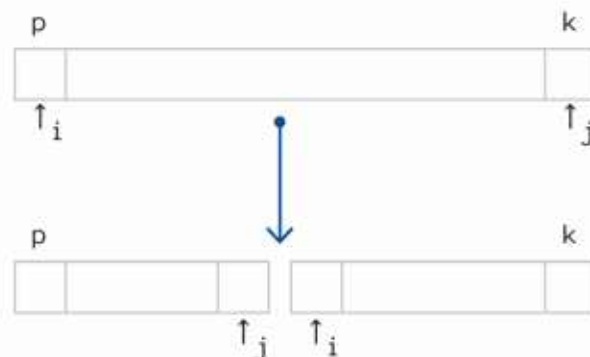
Rys. 20.4. Położenie indeksów i oraz j przed podziałem tablicy i po nim
