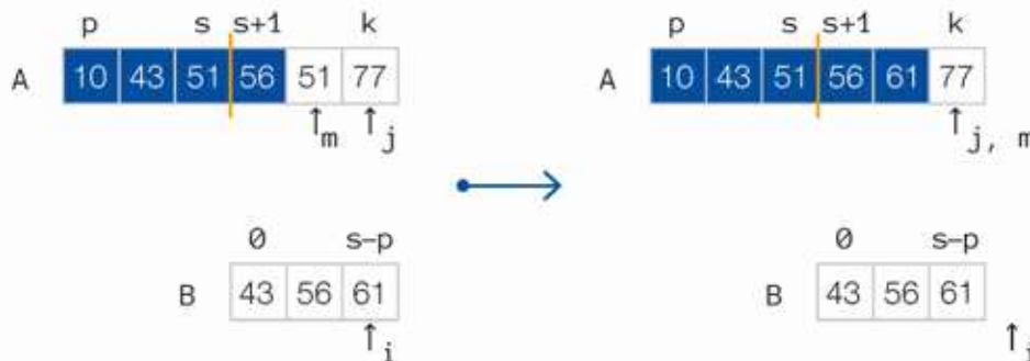
Rys. 20.9. Wybór przedostatniego elementu tablicy A
