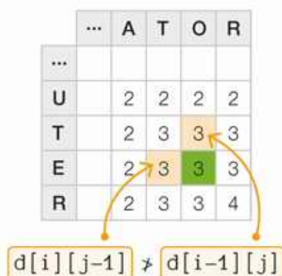
Rys. 19.14. Wybór pola przy wyznaczaniu wspólnego podciagu – analiza dwóch przypadków
