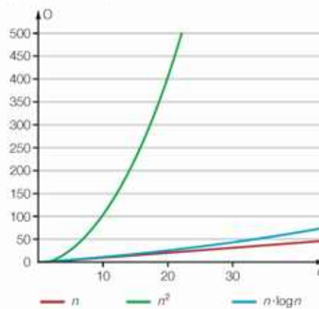
Rys. 11.1. Porównanie wykresów funkcji reprezentujących wybrane złożoności obliczeniowe
