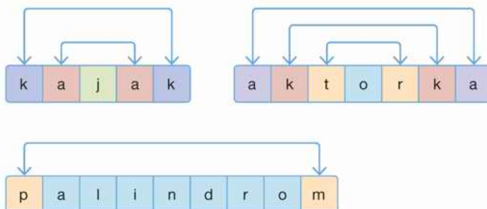
Rys. 4.1. Sprawdzenie, czy podane wyrazy są palindromami
