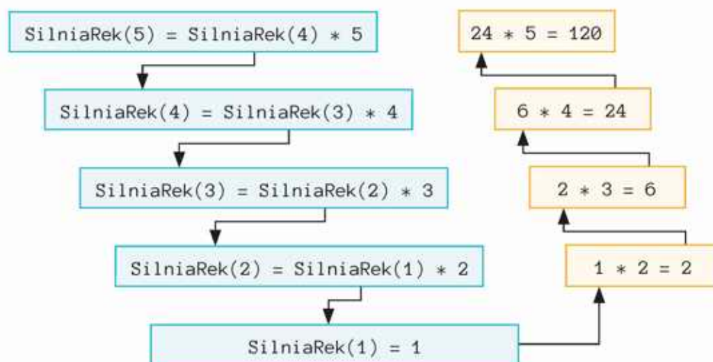
Rys. 17.2. Graficzna interpretacja obliczania wartości 5! z wykorzystaniem funkcji rekurencyjnej
