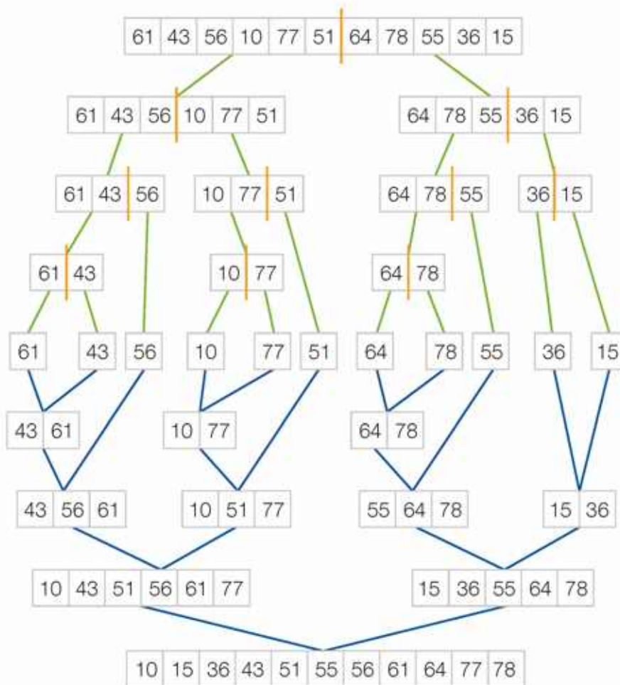
Rys. 20.5. Działanie algorytmu sortowania przez scalanie
