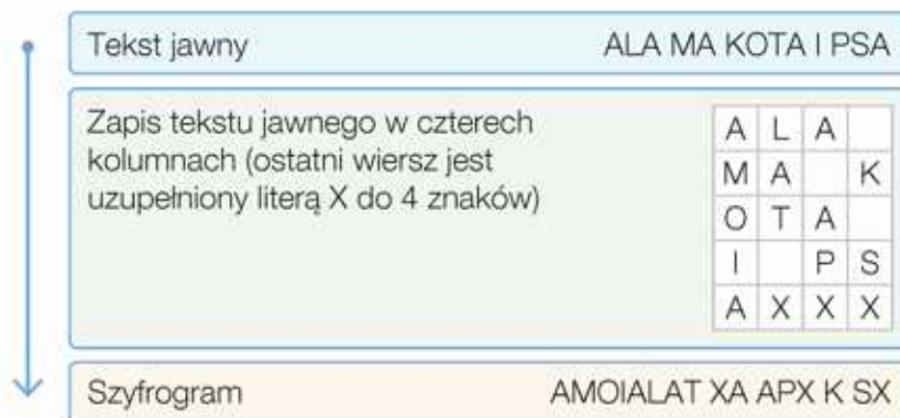
Rys. 13.1. Przykład szyfrowania informacji szyfrem kolumnowym z kluczem 4
