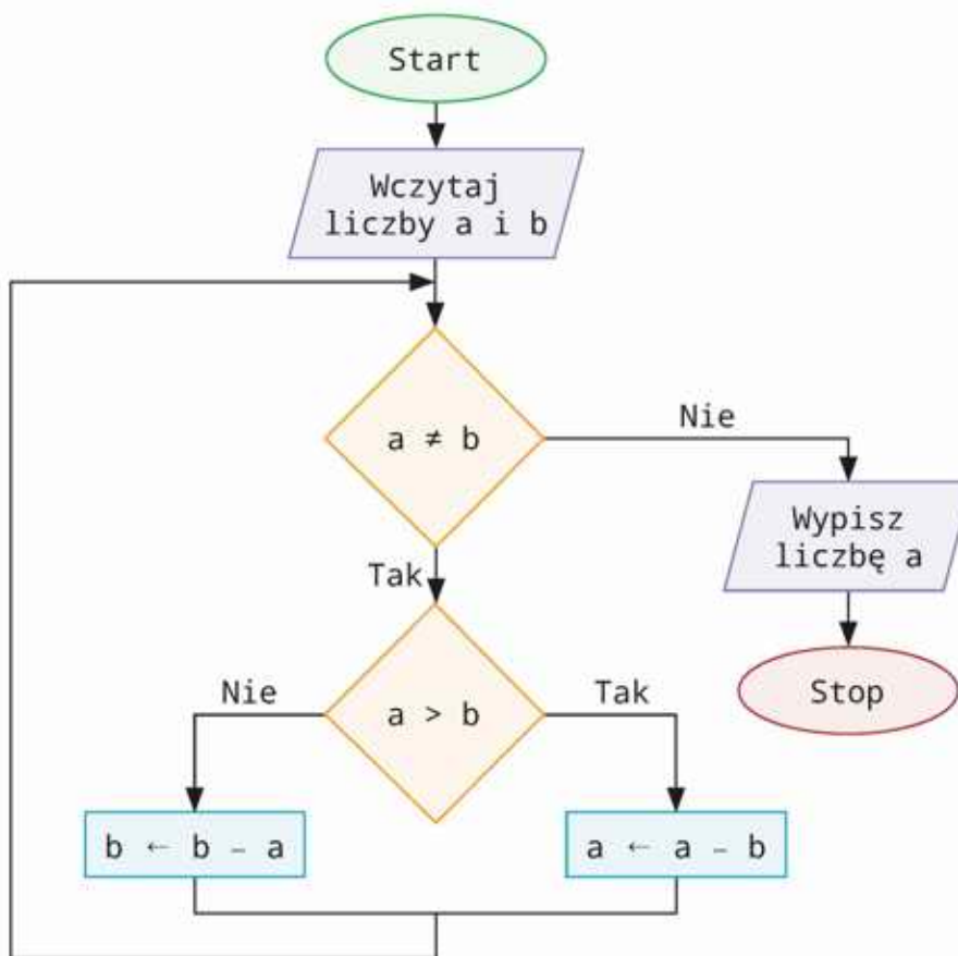
Rys. 7.2. Schemat blokowy algorytmu Euklidesa z wykorzystaniem odejmowania
