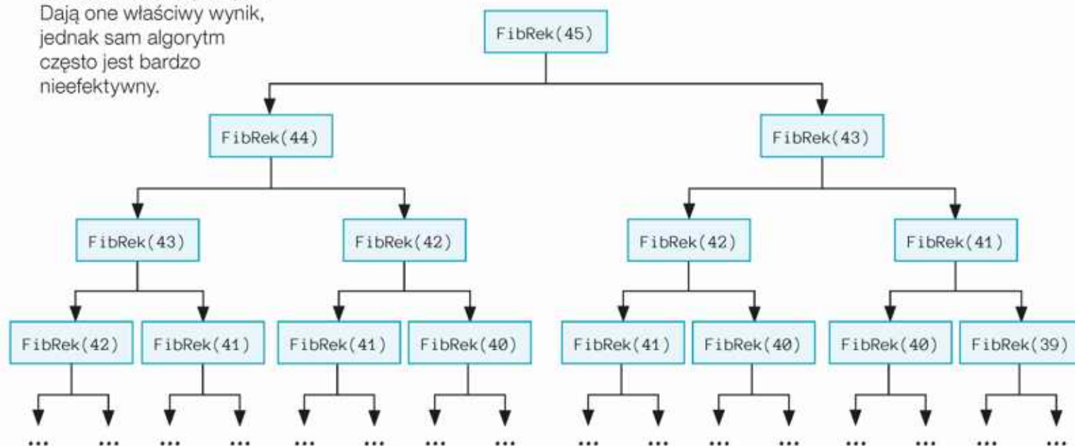
Rys. 17.7. Schemat wywołań funkcji FibRek dla n = 45
