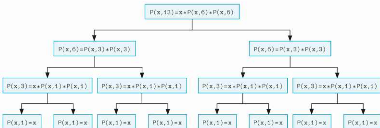
Rys. 17.4. Schemat rekurencyjnego wywoływania funkcji P, obliczającej potęgę liczby x o wykładniku 13
