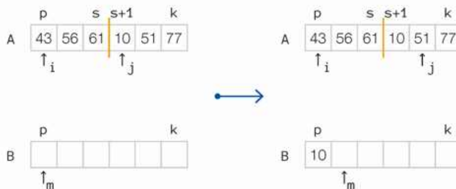
Rys. 20.6. Pierwszy krok scalania fragmentów danych – porównanie pierwszych elementów fragmentów i skopiowanie mniejszego
