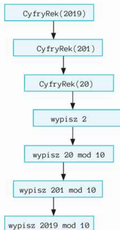
Rys. 17.3. Funkcja wypisująca cyfry od najbardziej znaczących
