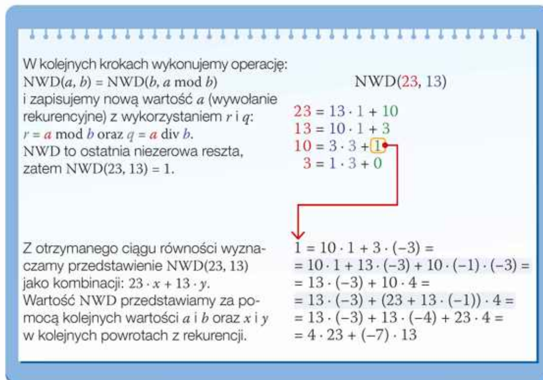
Rys. 17.8. Schemat postępowania przy obliczaniu \text{NWD}(23, 13)
