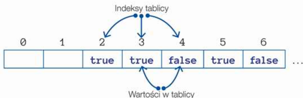
Rys. 14.1. Fragment tablicy Pierwsze z zaznaczeniem liczb pierwszych i złożonych
