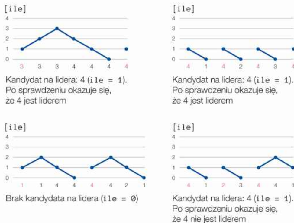
Rys. 16.1. Schematy objaśniające, jak się zlicza wystąpienia kandydatów na lidera w zbiorze
