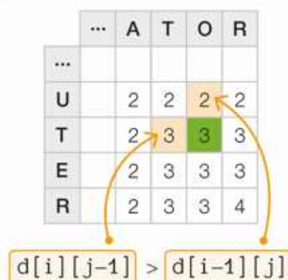
Rys. 19.14. Wybór pola przy wyznaczaniu wspólnego podciagu – analiza dwóch przypadków
