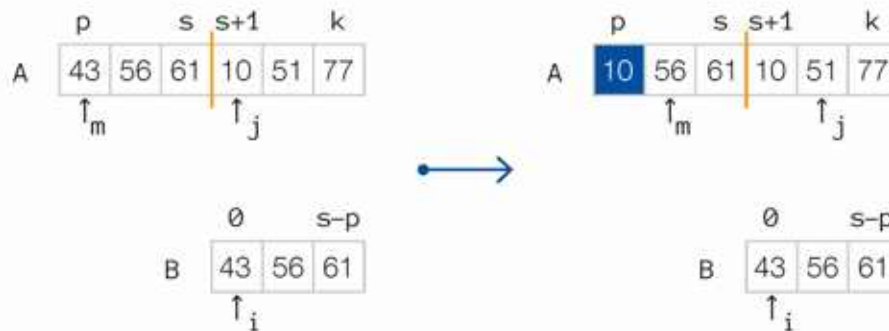
Rys. 20.8. Pierwszy krok scalania – porównanie pierwszych elementów scalanych fragmentów i skopiowanie mniejszego
