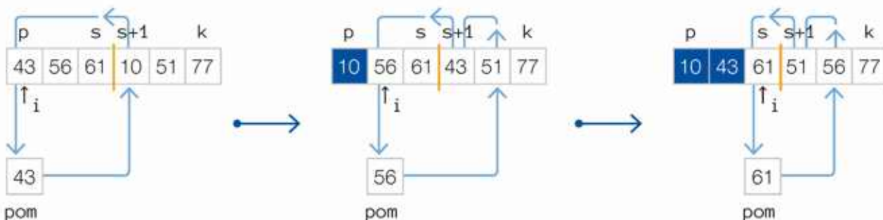
Rys. 20.10. Kolejne kroki scalania fragmentów danych metodą in situ
