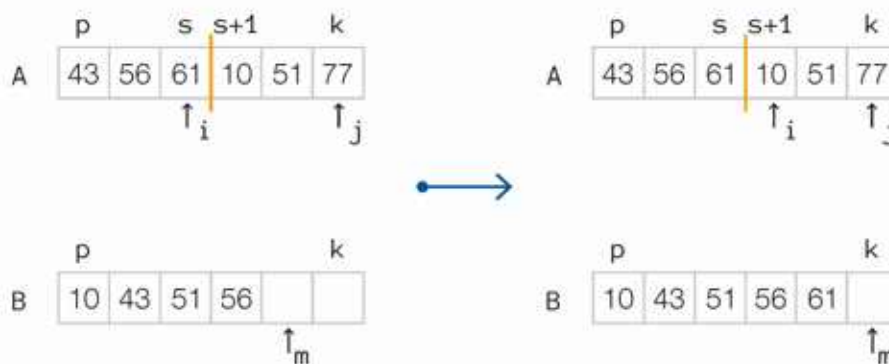
Rys. 20.7. Porównanie ostatnich elementów pierwszego i drugiego fragmentu
