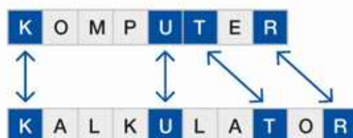
Rys. 19.12. Najdłuższy wspólny podciąg słów KOMPUTER i KALKULATOR
