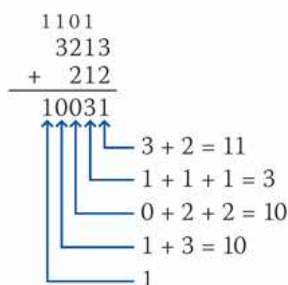
Rys. 6.1. Przykład dodawania liczb w systemie czwórkowym
