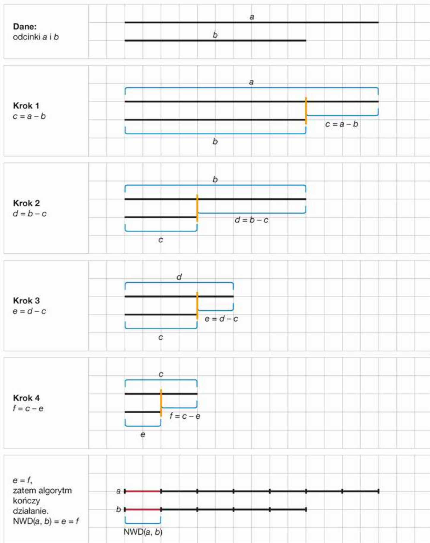
Rys. 7.1. Graficzne przedstawienie algorytmu Euklidesa z wykorzystaniem odejmowania
