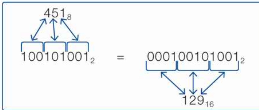
Rys. 2.1. Zamiana zapisu liczby pomiędzy systemami ósemkowym i szesnastkowym
