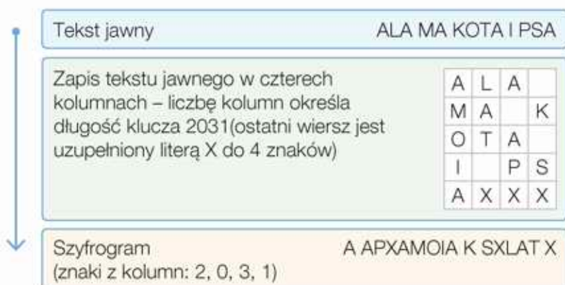
Rys. 13.2. Przykład szyfrowania informacji szyfrem kolumnowym z kluczem 2031
