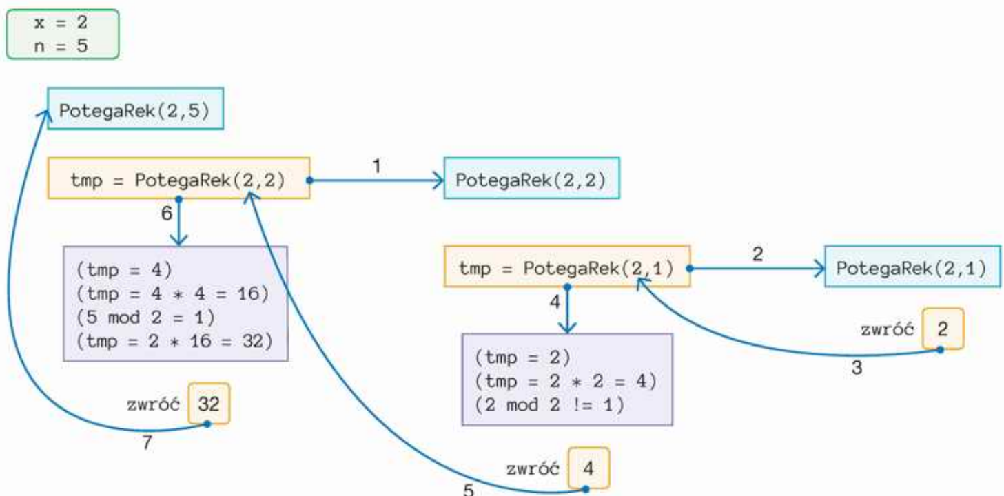
Rys. 17.5. Schemat kolejnych wywołań rekurencyjnych funkcji PotegaRek
