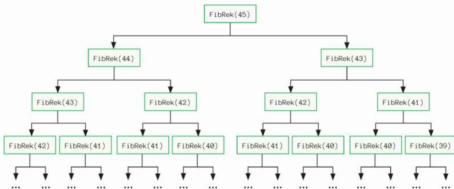
Rys. 5.11. Schemat wywołań rekurencyjnych funkcji FibRek dla n = 45
