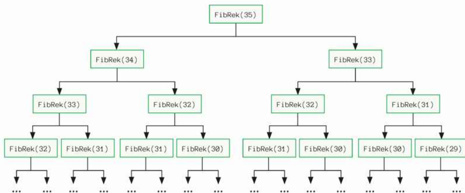
Rys. 10.11. Schemat wywołań rekurencyjnych funkcji FibRek dla n = 35
