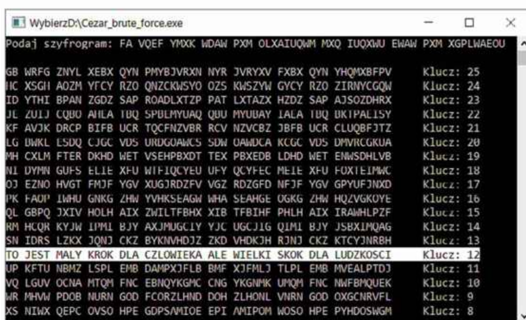
Rys. 2.10. Zastosowanie ataku siłowego do łamania szyfru Cezara
