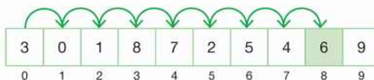
Rys. 8.5. Wyszukiwanie sekwencyjne
