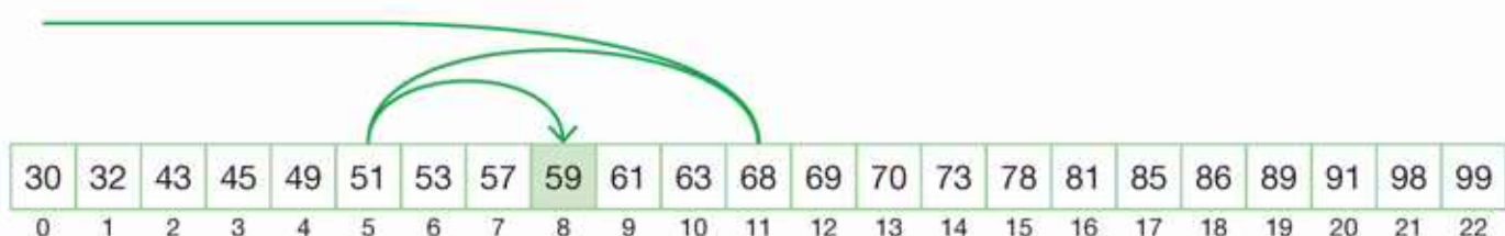
Rys. 3.6. Wyszukiwanie binarne
