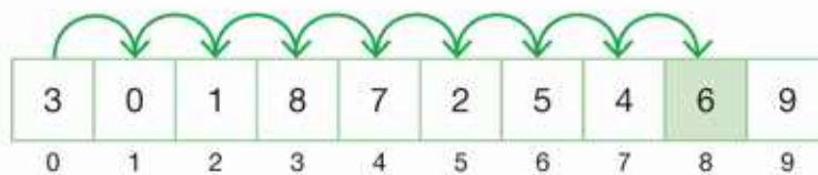
Rys. 3.5. Wyszukiwanie sekwencyjne
