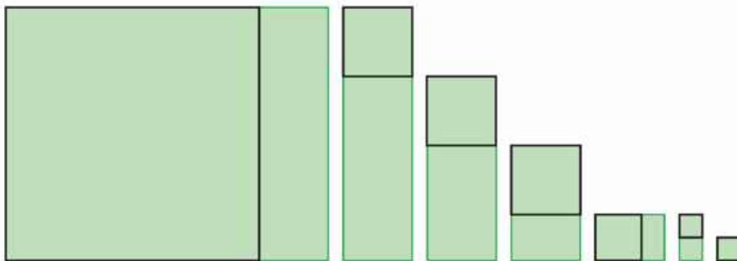
Rys. 4.1. Kolejne etapy wycinanki Euklidesa
