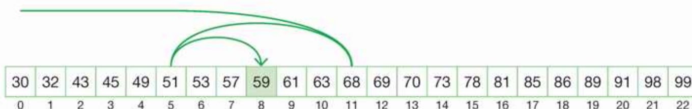
Rys. 8.6. Wyszukiwanie binarne
