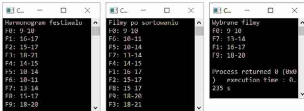
Rys. 4.8. Przykładowe wywołanie programu problem_kinomana.exe
