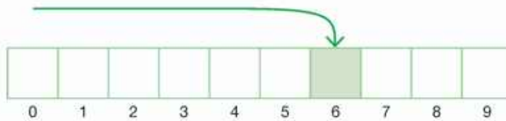
Rys. 3.4. Dostęp bezpośredni
