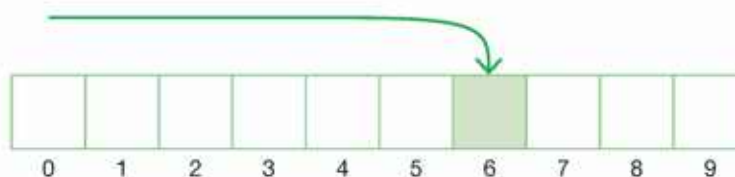
Rys. 8.4. Dostęp bezpośredni
