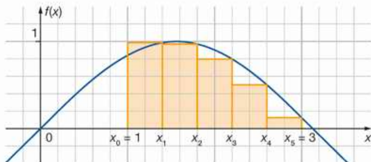
Rys. 8.5. Szukanie metodą prostokątów przybliżenia pola obszaru ograniczonego funkcją f(x) = \sin x i osią OX w przedziale [1; 3] dla n = 5
