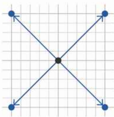
Rys. 8.12. Możliwe położenia cząstki po wykonaniu ruchu w jednostce czasu zgodnie z przedstawionym modelem
