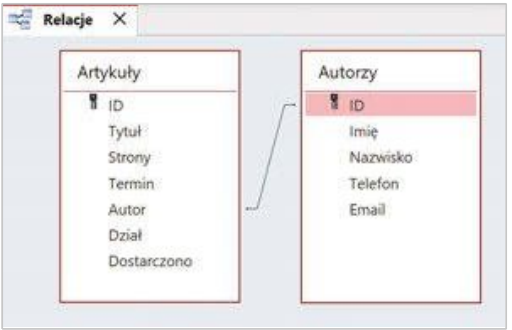
Rys. 5.7. Relacja między tabelami Artykuły i Autorzy
