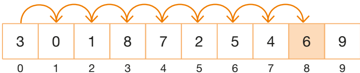
Rys. 9.8. Wyszukiwanie sekwencyjne
