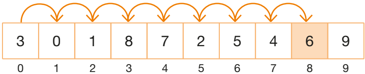
Rys. 13.8. Wyszukiwanie sekwencyjne
