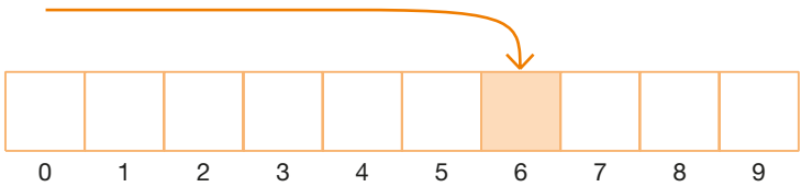
Rys. 13.7. Dostęp bezpośredni
