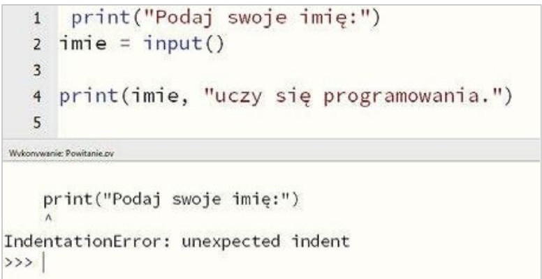
Rys. 6.5. Błąd składniowy w kodzie źródłowym programu
