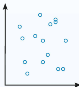
korelacja zerowa, r = 0
