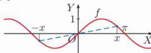
Funkcja f(x) = \sin x , określona dla x \in \mathbf{R} , jest nieparzysta.
