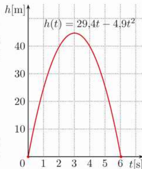
Wykres funkcji h opisującej wysokość, na której znajdowała się kula w chwili t .
