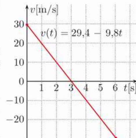
Wykres funkcji v opisującej prędkość, z którą poruszała się kula w chwili t .
