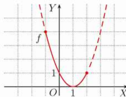
Wykres funkcji f: \langle -1; 2 \rangle \rightarrow \mathbf{R} danej wzorem f(x) = (x - 1)^2
