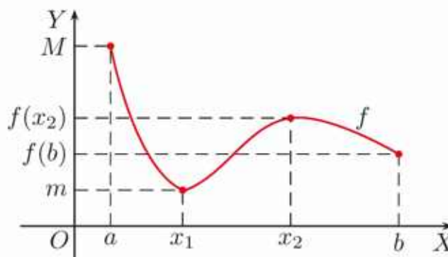
Wartość najmniejsza m = f(x_1) , wartość największa M = f(a)
