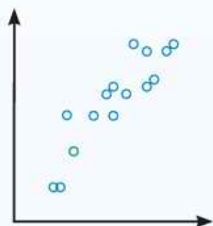
silna korelacja dodatnia, r = 0,9
