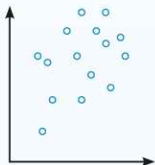
słaba korelacja dodatnia, r = 0,4
