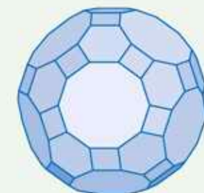
dwudziesto- -dwunastościan rombów wielki
