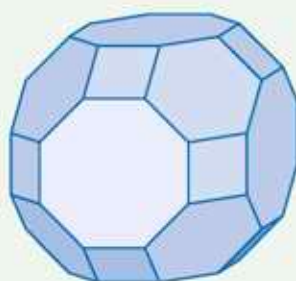
sześćcio-ośmiościan rombów wielki
