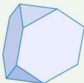
czworościan ścięty
