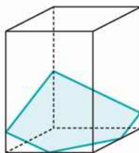
pięciokąt
