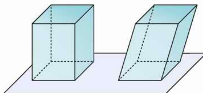
równoległoscian prosty
