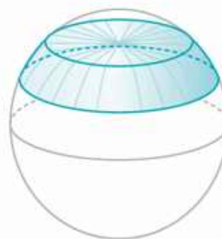
warstwa kuli
