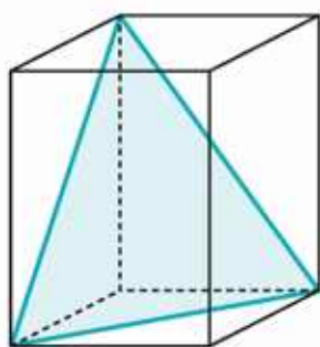
trójkąt
