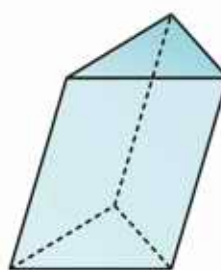
graniastosłup trójkątny
