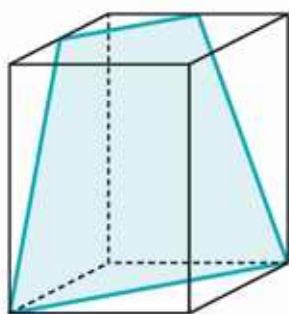
czworokąt (trapez)
