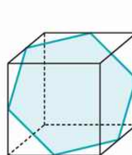
sześciokąt
