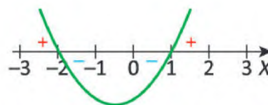
Szkic wykresu funkcji y = (x+2)(x-1)
