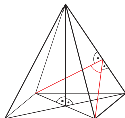
Kąt między płaszczyznami sąsiednich ścian bocznych.
